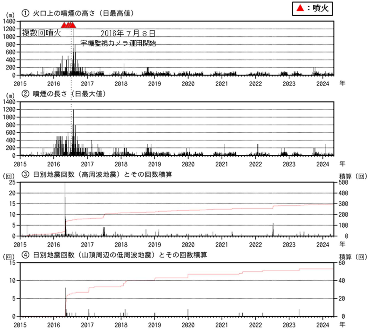
図3 新潟焼山 火山活動経過図（短期）（2015年1月1日～2024年4月30日）
