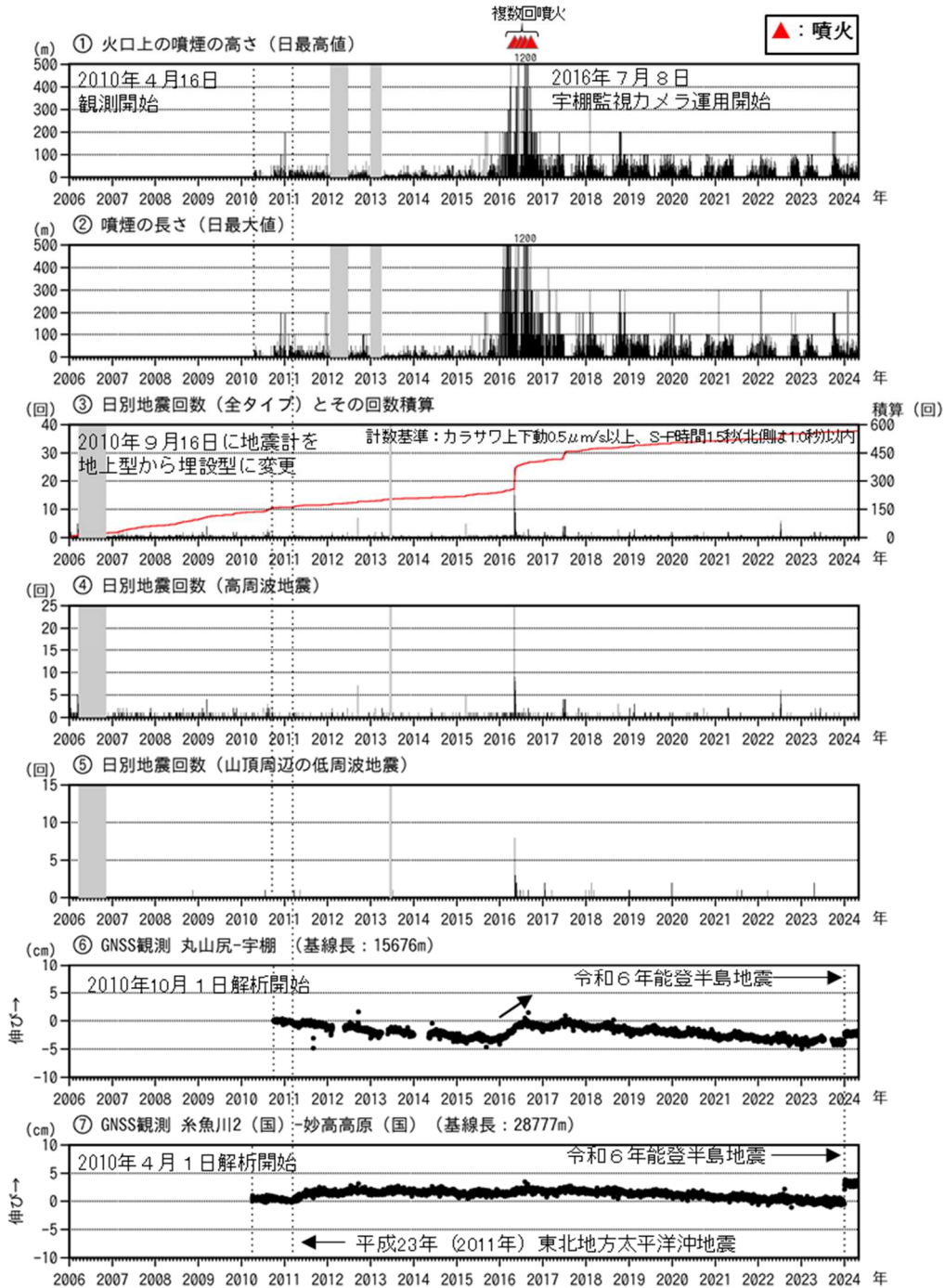
図2 新潟焼山 火山活動経過図（2006年1月1日～2024年4月30日）
