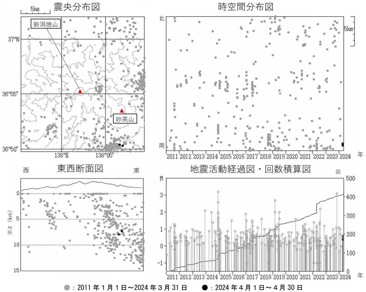
図4 新潟焼山 広域地震観測網による山体・周辺の地震活動（2011年1月1日～2024年4月30日）
