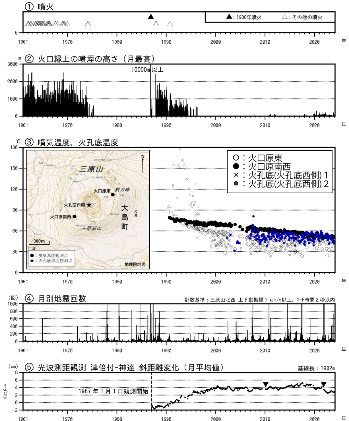
図1 伊豆大島 長期間の火山活動経過図 (1961年1月～2024年2月29日)
