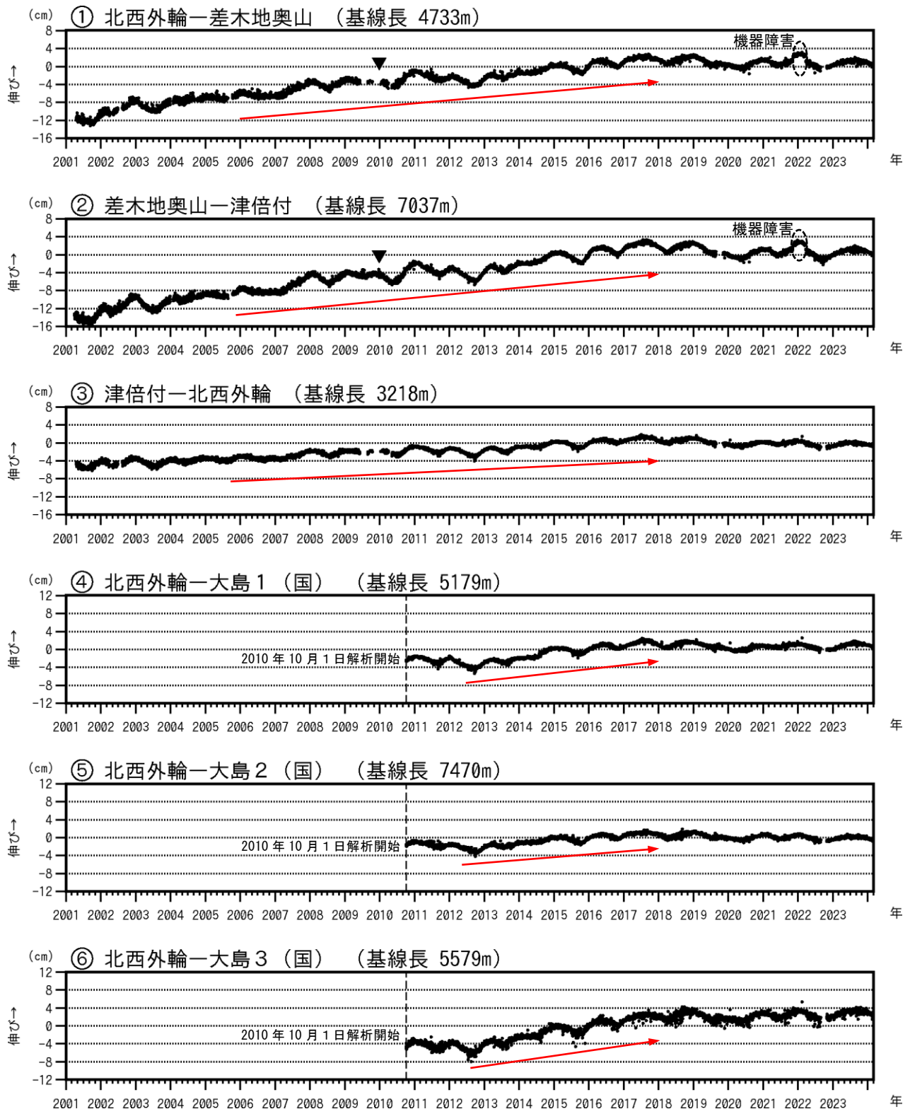
図3-1 伊豆大島 GNSS 連続観測による基線長変化(2001年1月～2024年2月29日)
