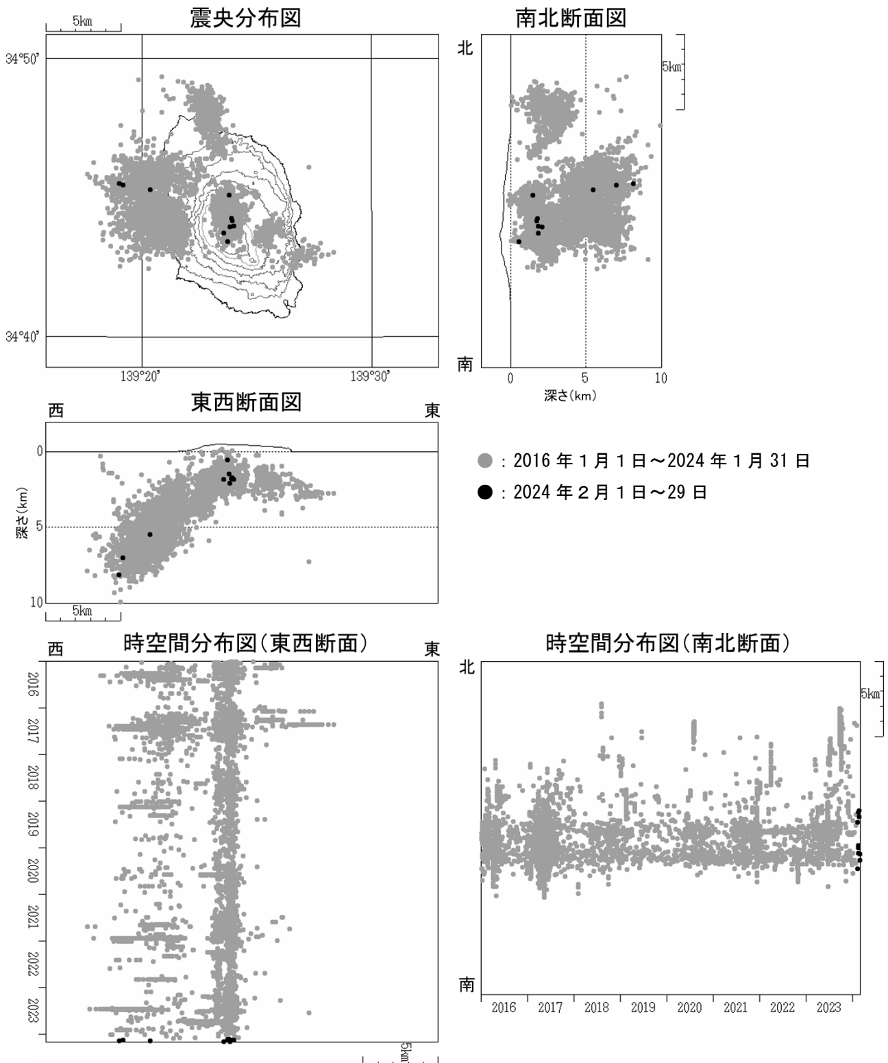
図4 伊豆大島 震源分布図（2016 年 1 月 1 日～2024 年 2 月 29 日）
