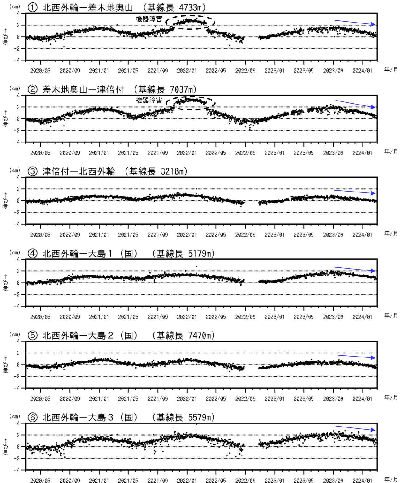
図3-2 伊豆大島 GNSS 連続観測による基線長変化(2020年3月～2024年2月29日)
