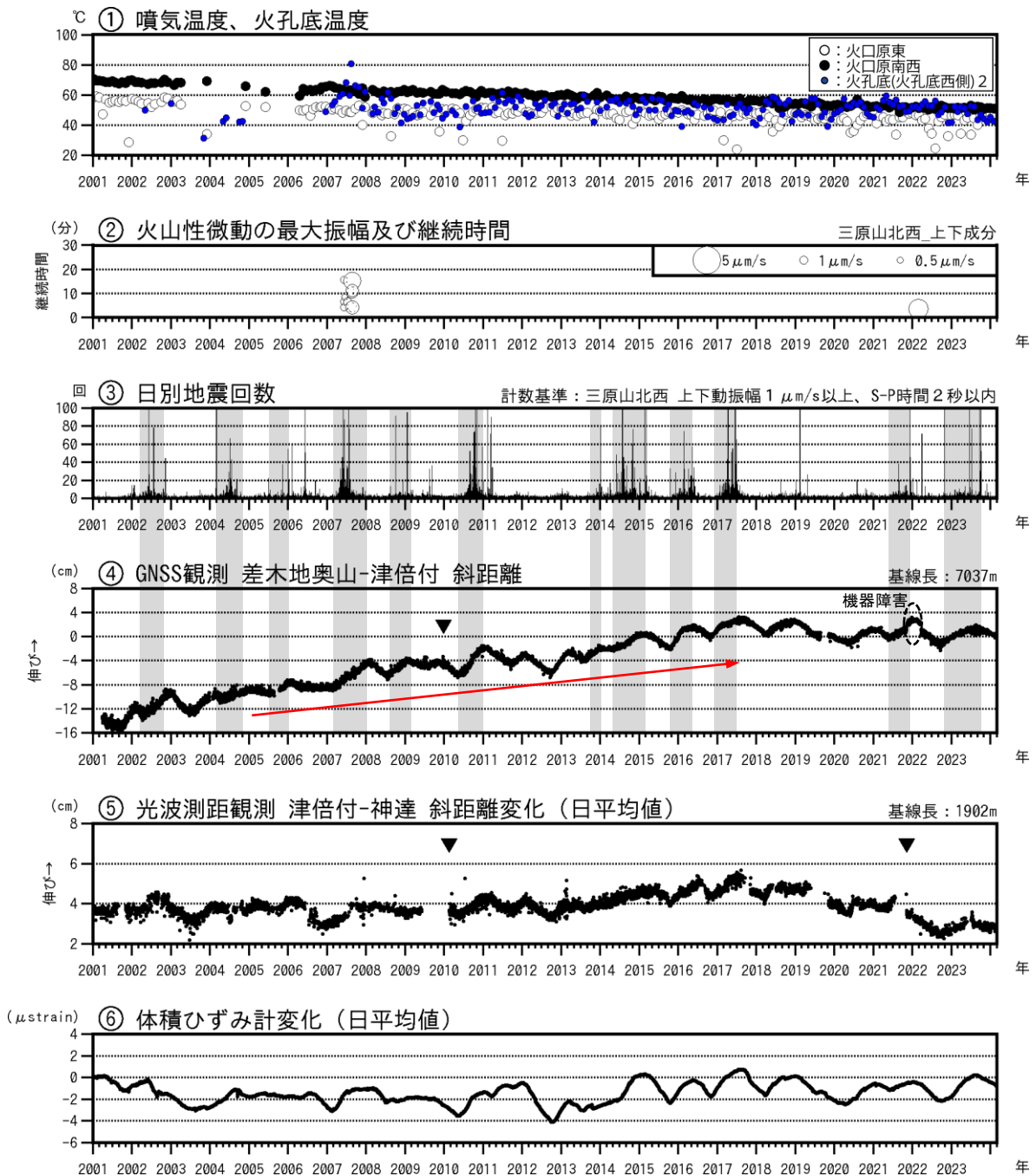
図2 伊豆大島 最近の火山活動経過図（2001年1月～2024年2月29日）
