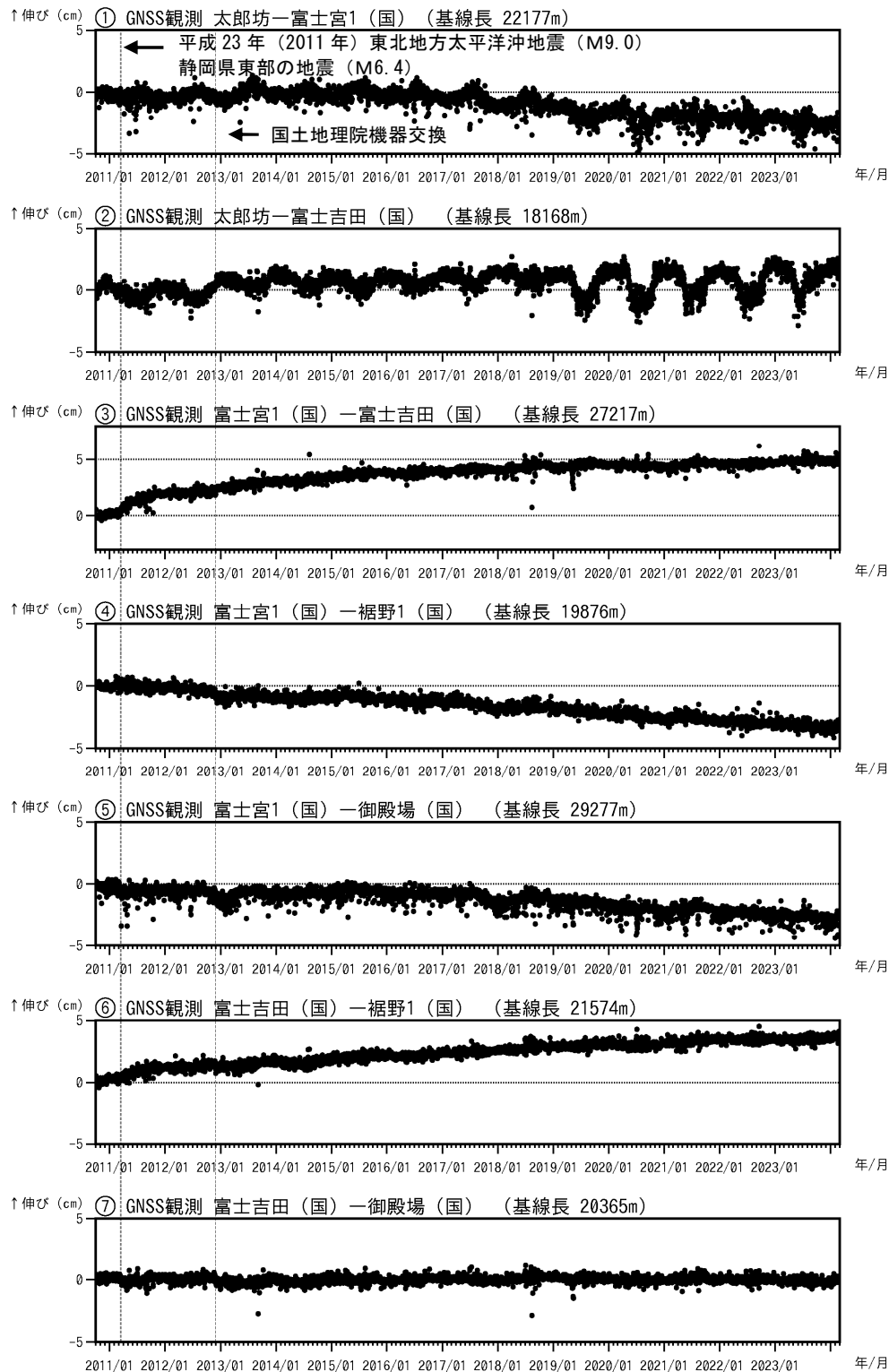
図4 富士山 GNSS 連続観測による基線長変化 (2010 年 10 月 1 日～2024 年 2 月 29 日) (国): 国土地理院 「平成 23 年 (2011 年) 東北地方太平洋沖地震」及び 2011 年 3 月 15 日に発生した静岡県東部の地震 (M 6.4) によるステップ状の変化を補正しています。 ①～⑦は図5の GNSS 基線①～⑦に対応しています。
