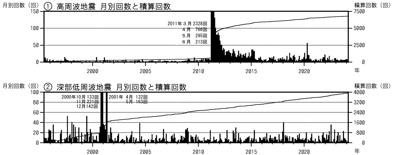
図2 富士山 月別地震回数（1995年6月1日～2024年2月29日）
