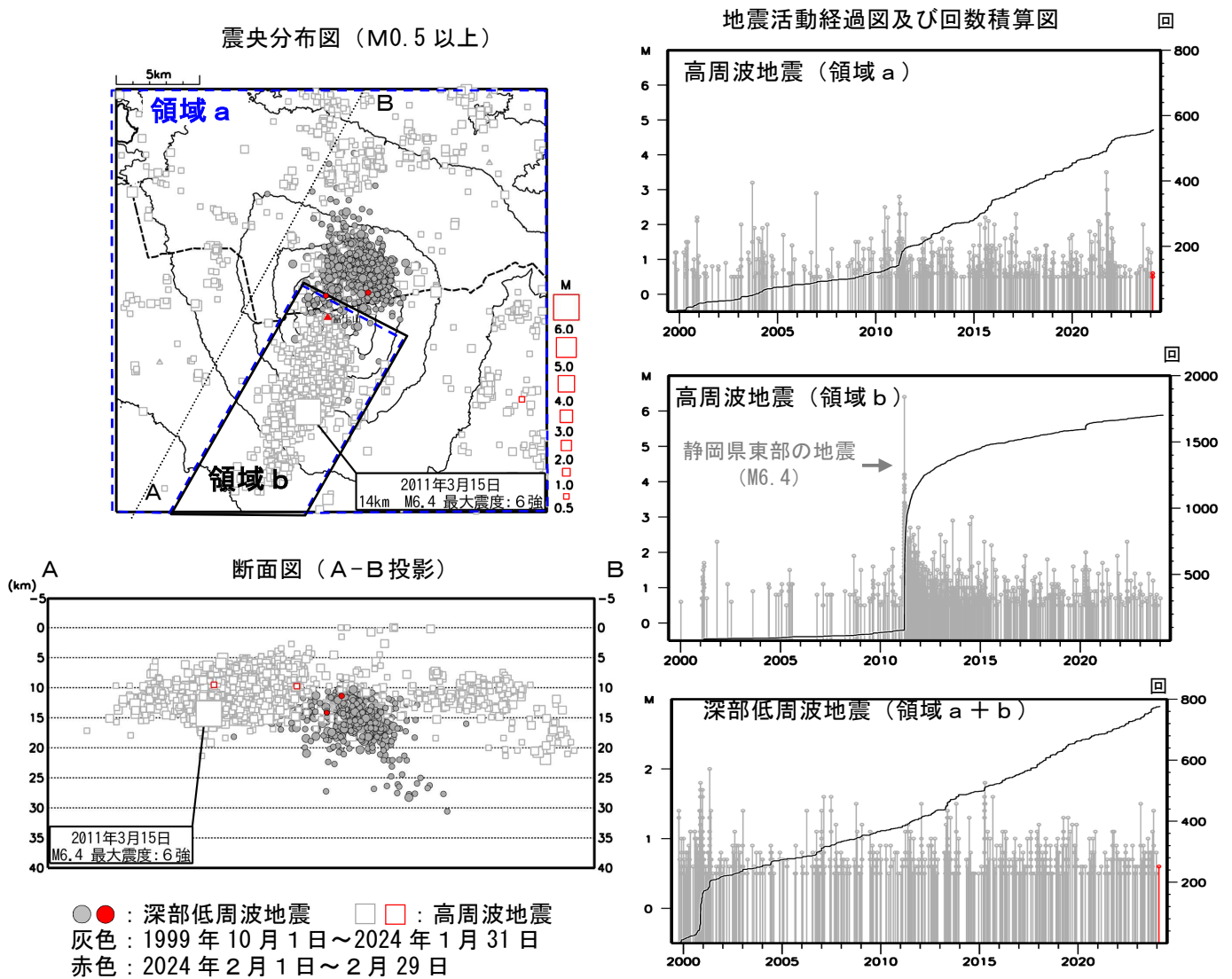
図3 富士山 広域地震観測網による山体及び周辺の地震活動（1999年10月1日～2024年2月29日）
