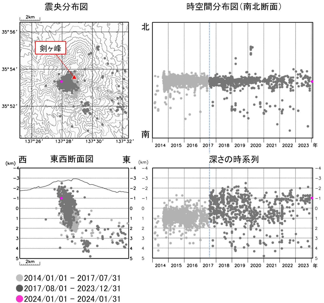
図4 御嶽山 震源分布図（2014年1月1日～2024年1月31日） 2017年8月1日（水色破線）以降の震源分布は、震源計算に使用する観測点を新たに追加して再計算したものを示しています。
