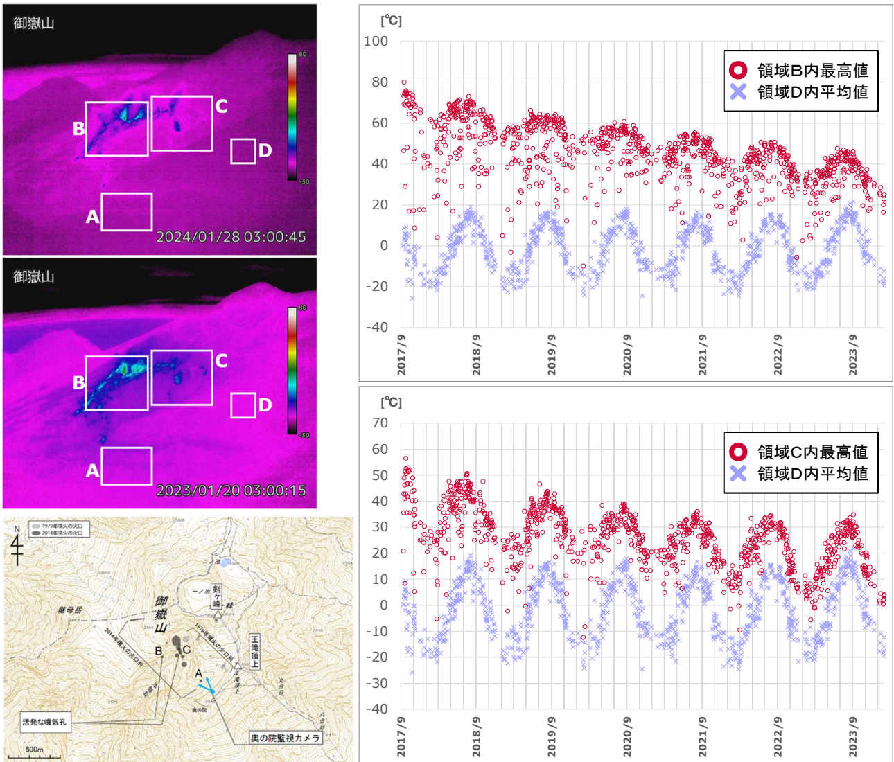
図3 御嶽山 奥の院赤外熱映像カメラによる剣ヶ峰南西側における最高温度の推移 (2017年9月13日～2024年1月31日)
