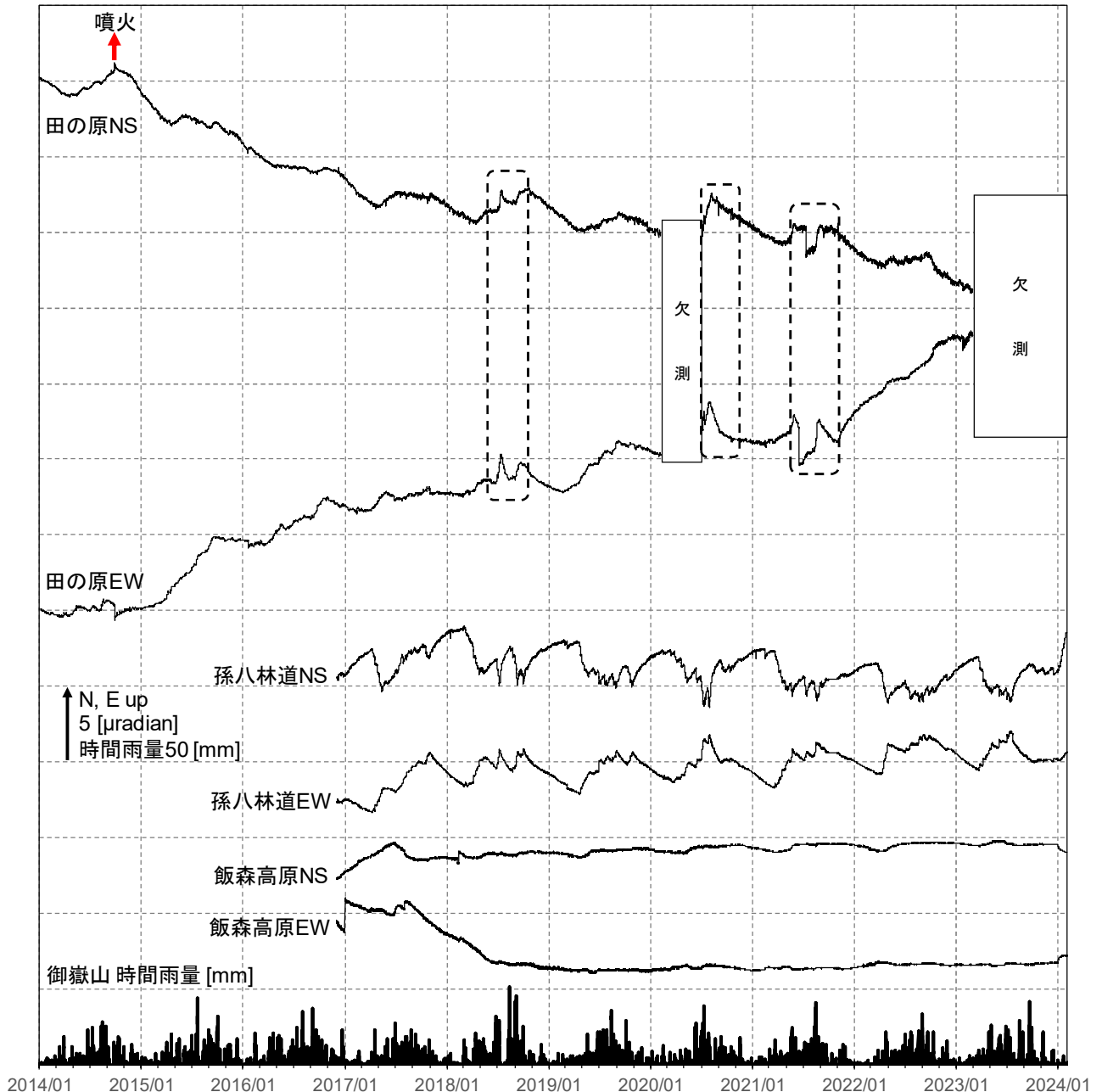
図6 御嶽山 傾斜変動（2014年1月1日～2024年1月31日）
