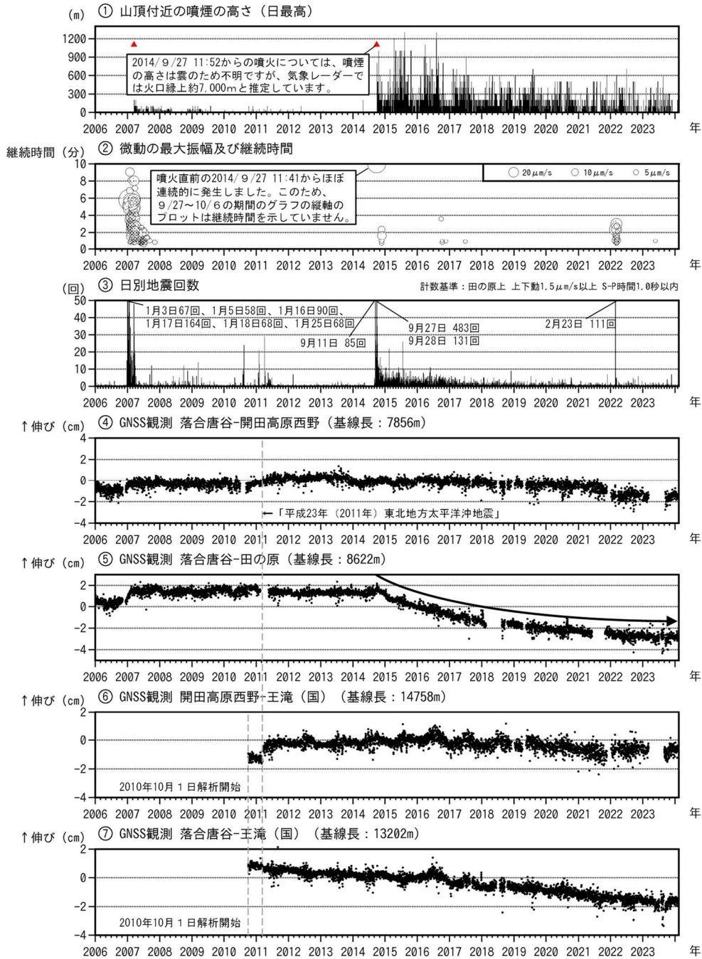
図1 御嶽山 長期間の火山活動経過図（2006年1月1日～2024年1月31日）
