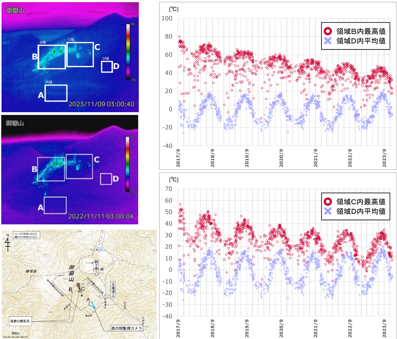
図3 御嶽山 奥の院赤外熱映像カメラによる剣ヶ峰南西側における最高温度の推移 (2017年9月13日～2023年11月30日)
