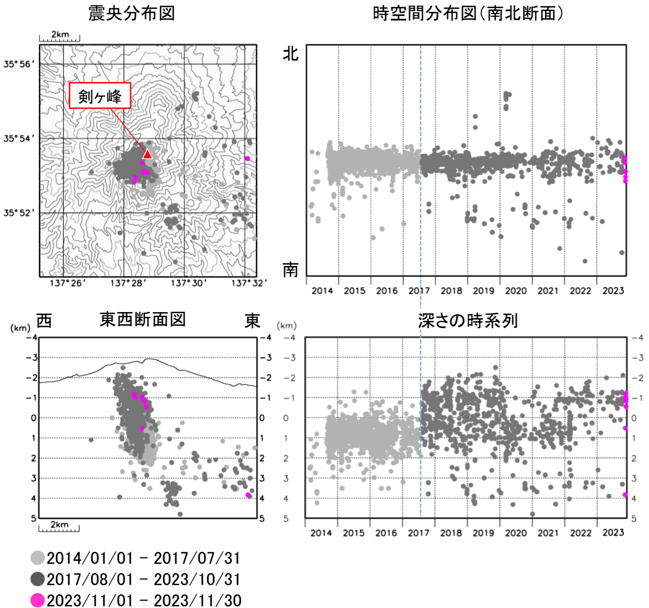
図4 御嶽山 震源分布図（2014年1月1日～2023年11月30日） 2017年8月1日（水色破線）以降の震源分布は、震源計算に使用する観測点を新たに追加して再計算したものを示しています。
