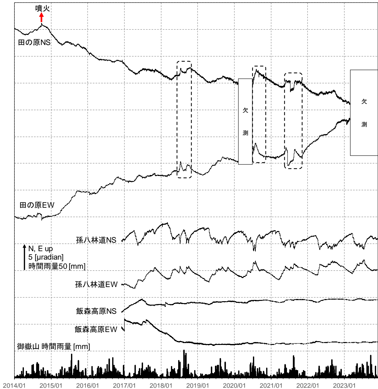
図6 御嶽山 傾斜変動（2014年1月1日～2023年11月30日） データは時間平均値、田の原及び孫八林道観測点のデータは潮汐補正済みです。 2018年7月頃及び2020年7月頃の破線で囲んだ部分は、降水による影響と考えられる変動を示します。 2021年6月頃の破線で囲んだ部分は、降水及び田の原観測点の近傍での建設工事の影響と考えられる変動を示します。
