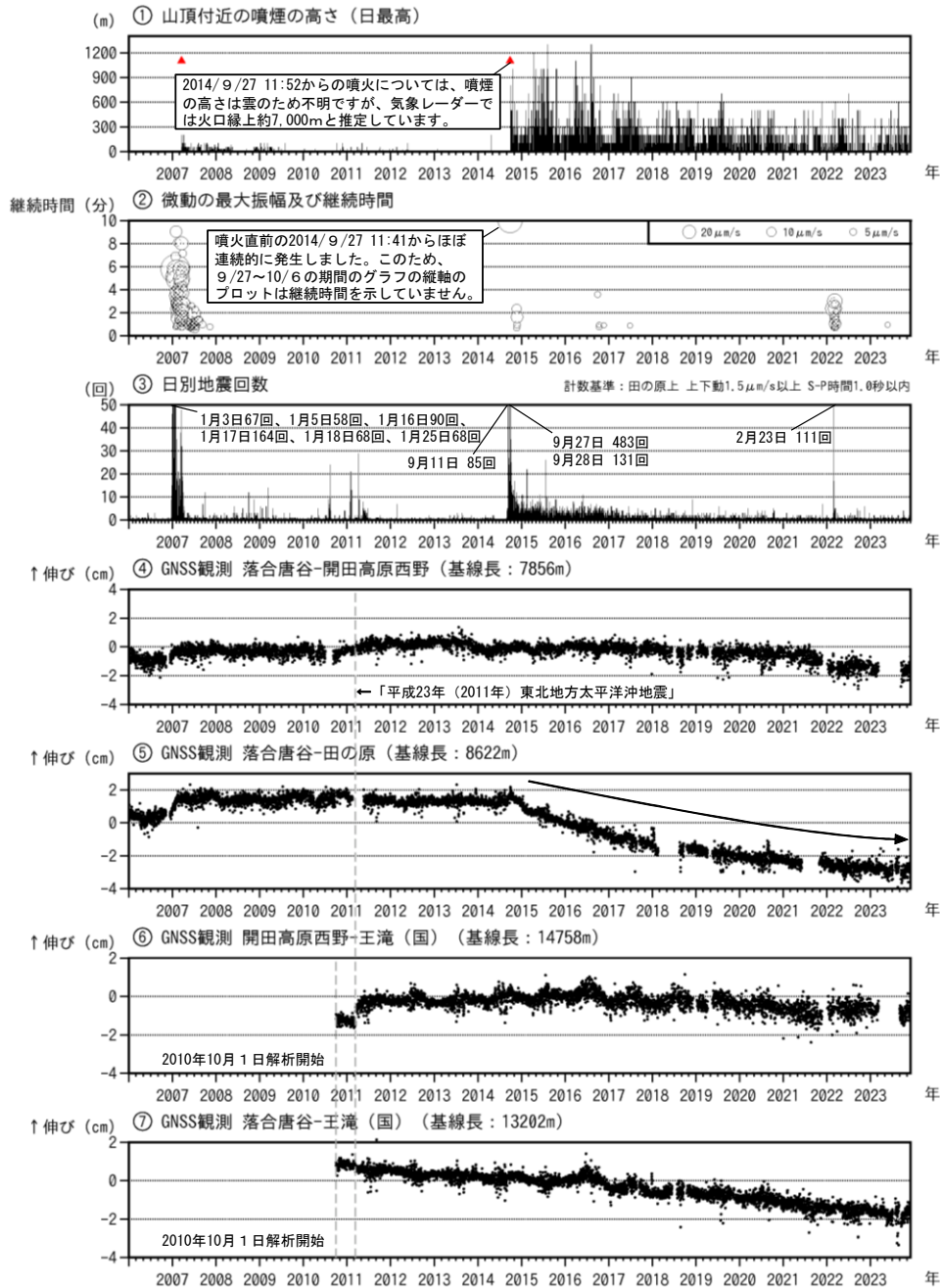
図1 御嶽山 長期間の火山活動経過図 (2006年1月1日~2023年11月30日)
