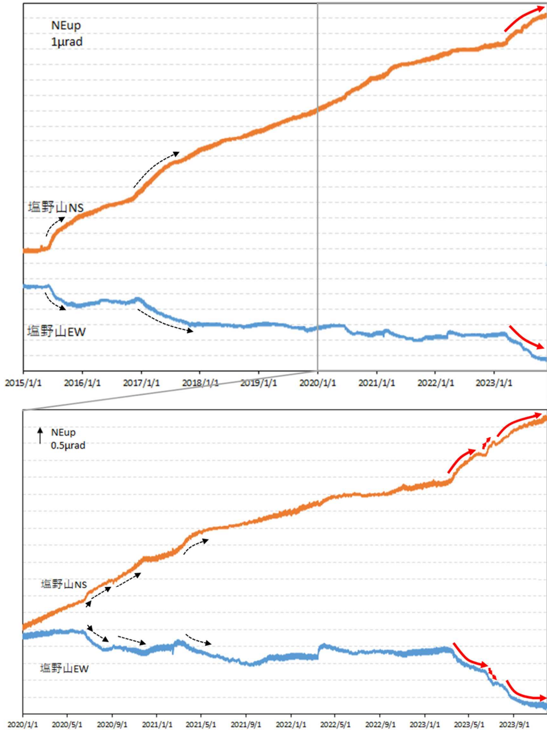
図8 浅間山 塩野山観測点における傾斜データ（2015年1月1日～2023年11月30日） データは時間平均値を使用しており、長期にわたるトレンドを補正しています。 下段は上段に比べて縦軸を拡大しています。
