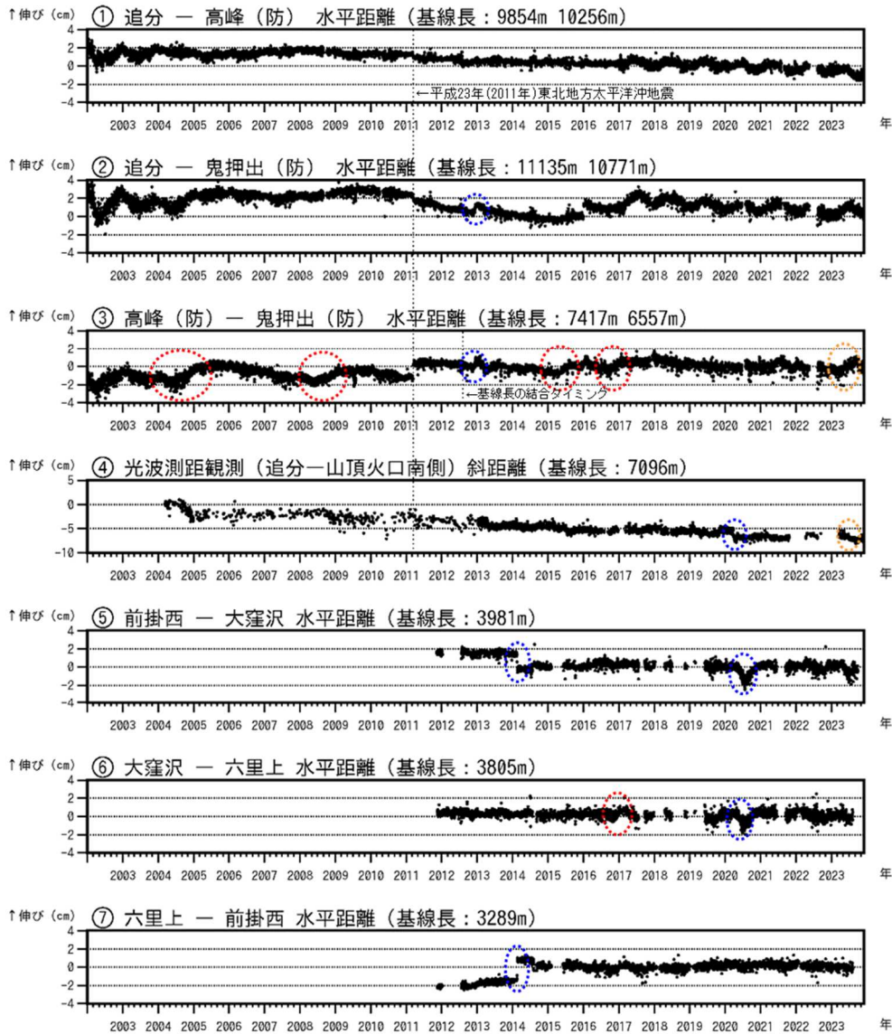
図 6 - 1 浅間山 GNSS 連続観測及び光波測距観測の結果(2002 年 1 月 1 日~2023 年 11 月 30 日)
