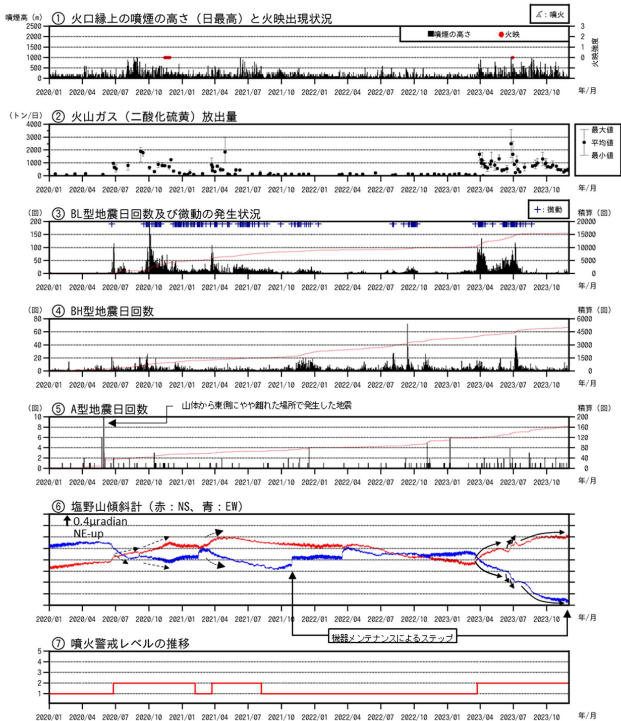
図3 浅間山 火山活動経過図（2020年1月1日～2023年11月30日）
