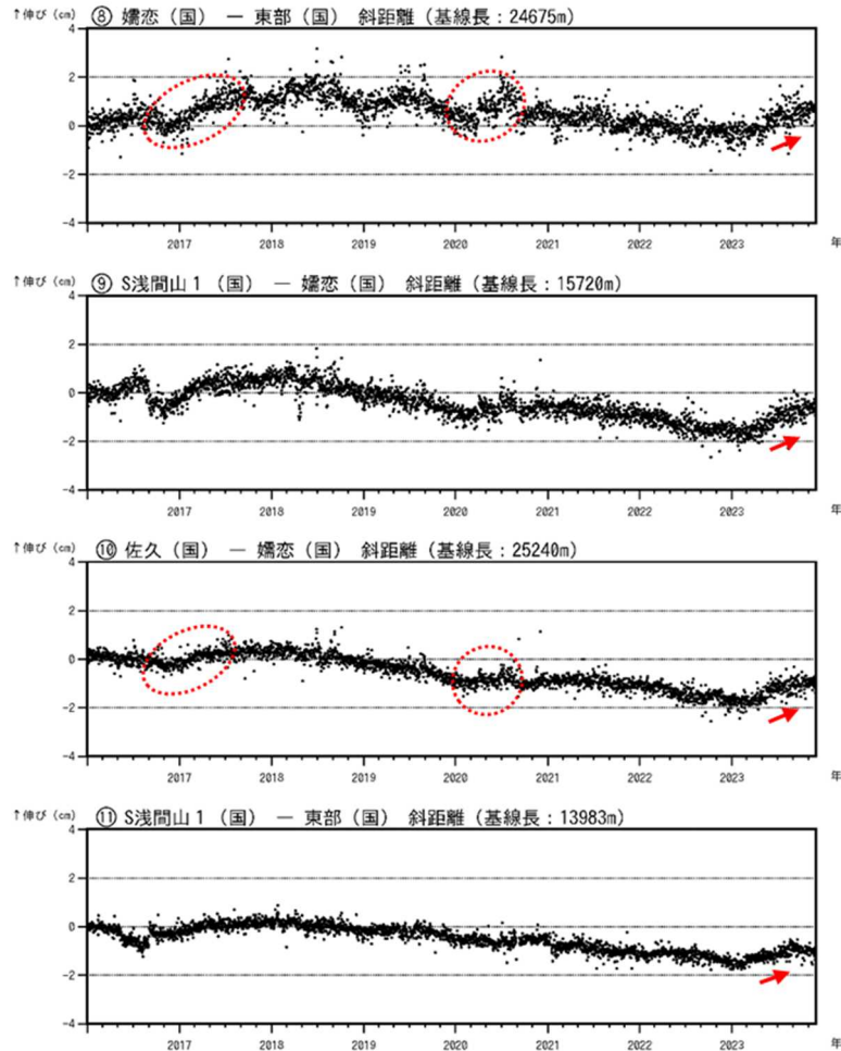
図6-2 浅間山 GNSS 連続観測結果(2016年1月1日~2023年11月30日) ⑧⑨⑩⑪は図7の⑧⑨⑩⑪にそれぞれ対応しています。空白部分は欠測を示します。(国)：国土地理院。
