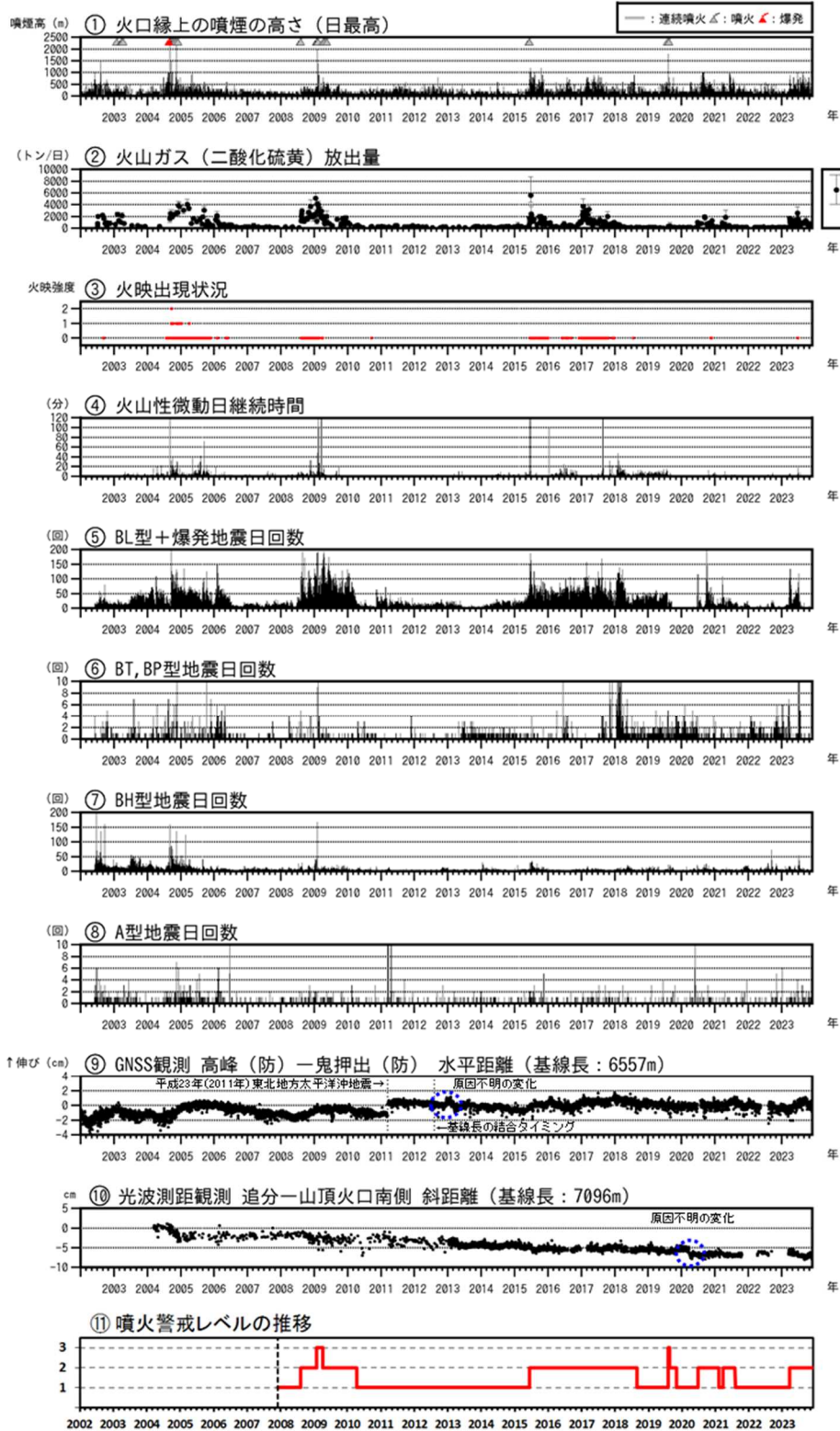
図4 浅間山 火山活動経過図（2002年1月1日～2023年11月30日）
