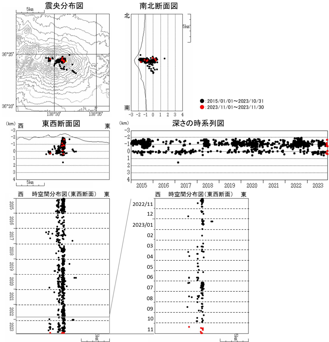
図5 浅間山 震源分布図（2015年1月1日～2023年11月30日）
