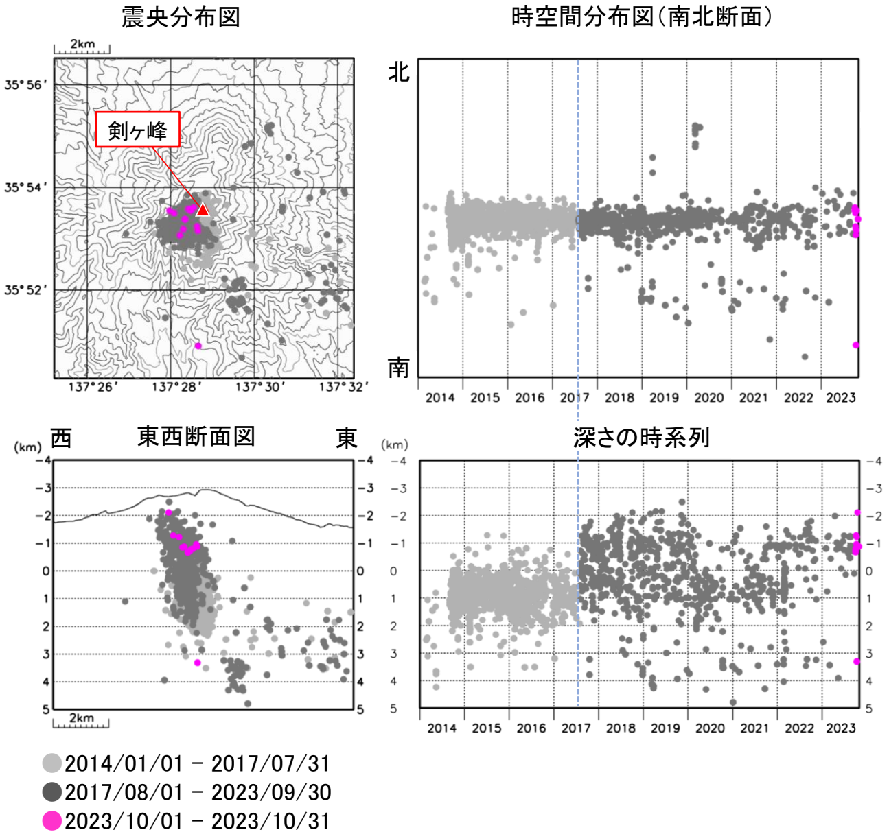
図4 御嶽山 震源分布図（2014年1月1日～2023年10月31日） 2017年8月1日（水色破線）以降の震源分布は、震源計算に使用する観測点を新たに追加して再計算したものを示しています。
