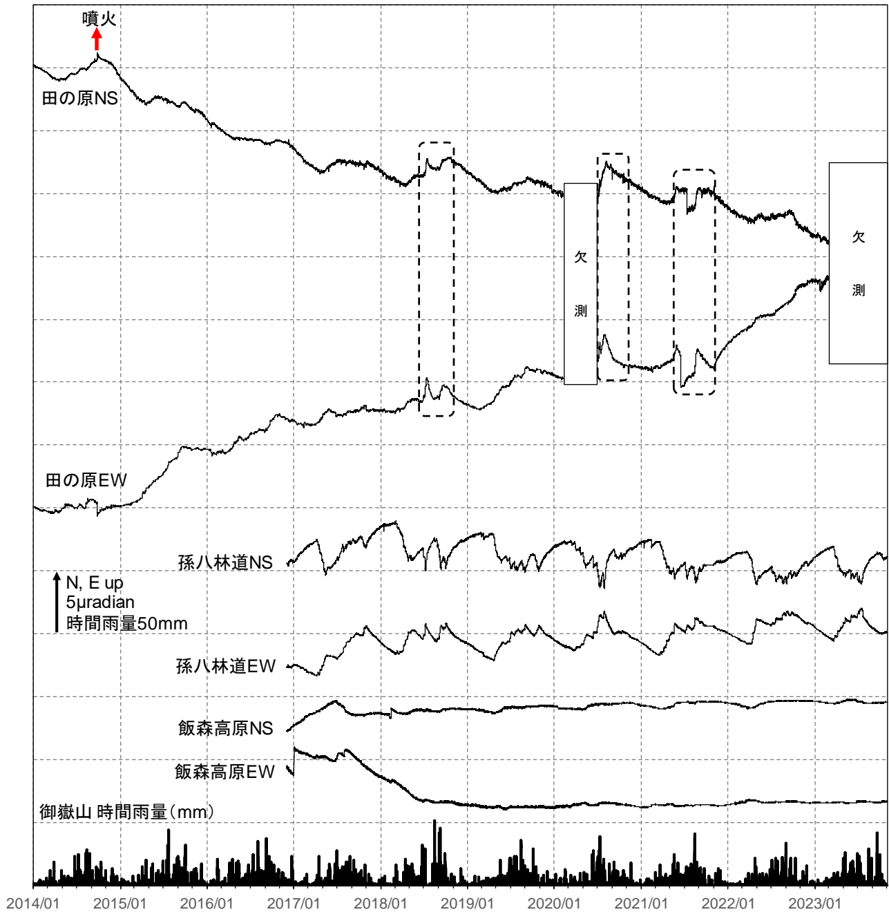
図6 御嶽山 傾斜変動（2014年1月1日～2023年10月31日） データは時間平均値、田の原及び孫八林道観測点のデータは潮汐補正済みです。 2018年7月頃及び2020年7月頃の破線で囲んだ部分は、降水による影響と考えられる変動を示します。 2021年6月頃の破線で囲んだ部分は、降水及び田の原観測点の近傍での建設工事の影響と考えられる変動を示します。
