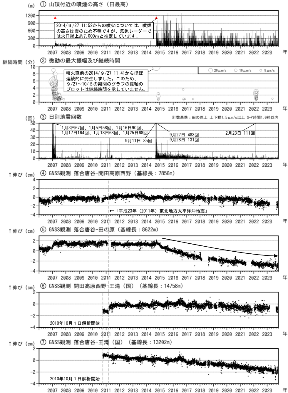
図1 御嶽山 長期間の火山活動経過図 (2006年1月1日~2023年10月31日)
