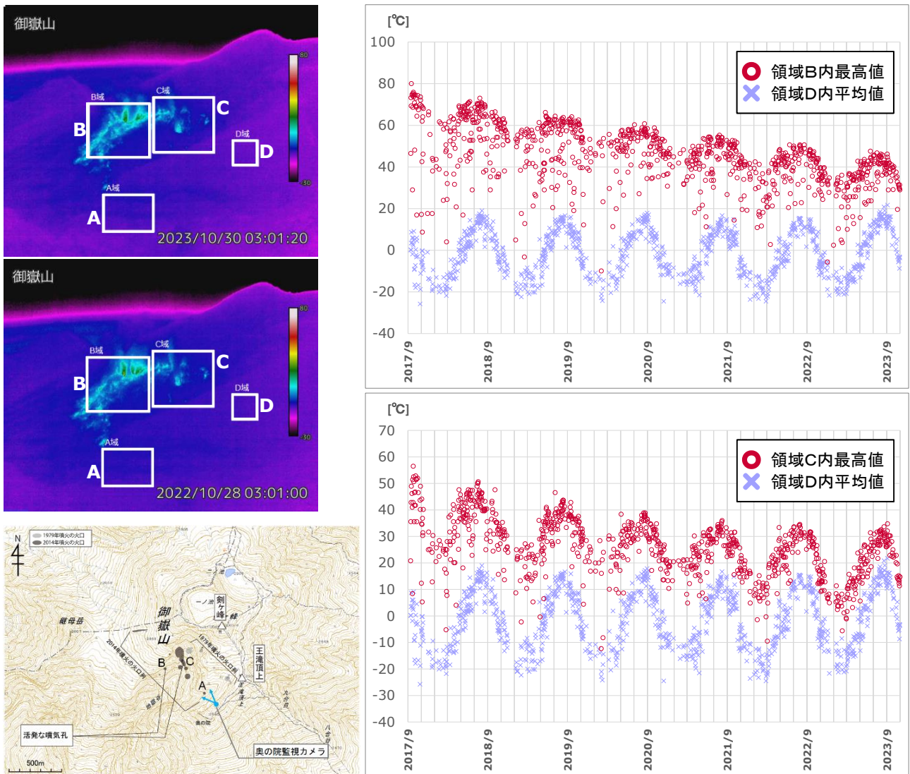
図3 御嶽山 奥の院赤外熱映像カメラによる剣ヶ峰南西側における最高温度の推移 (2017年9月13日~2023年10月31日)
