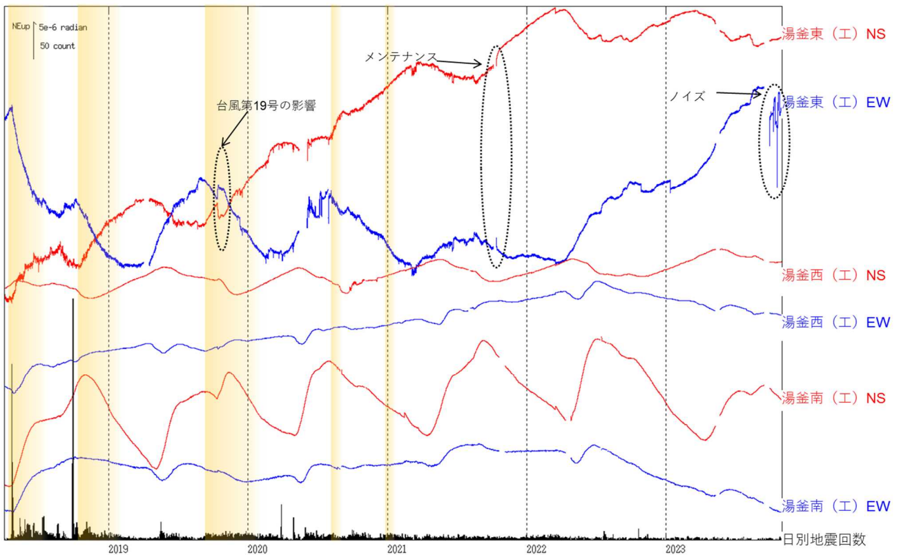
図5 草津白根山（白根山（湯釜付近）） 傾斜変動（2018年4月1日～2023年10月31日）
