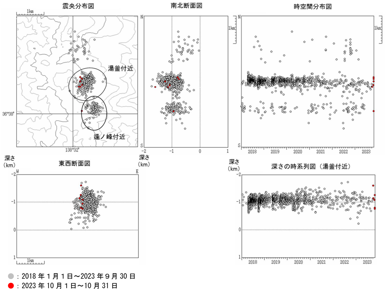
図4 草津白根山 震源分布図（2018年1月1日～2023年10月31日）
