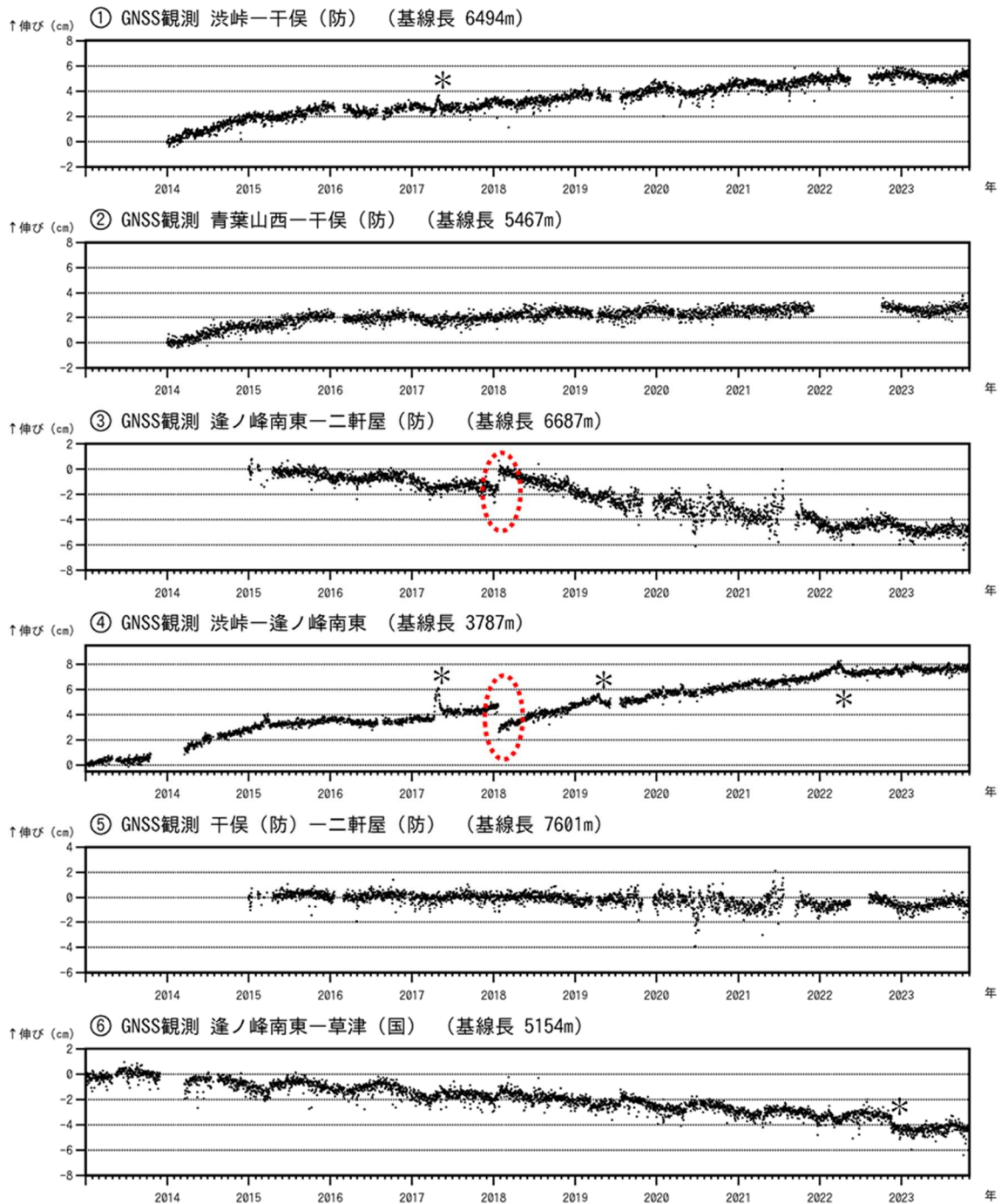
図6 草津白根山 GNSS連続観測の結果（2013年1月1日～2023年10月31日）
