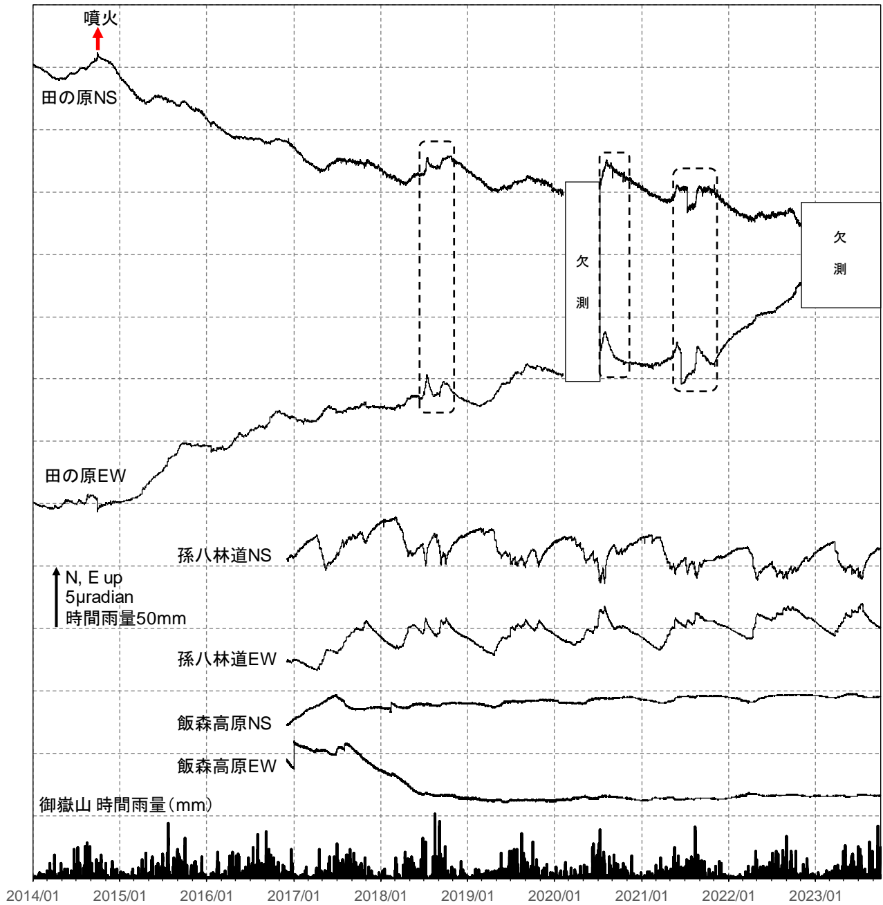
図6 御嶽山 傾斜変動（2014年1月1日～2023年9月30日）
