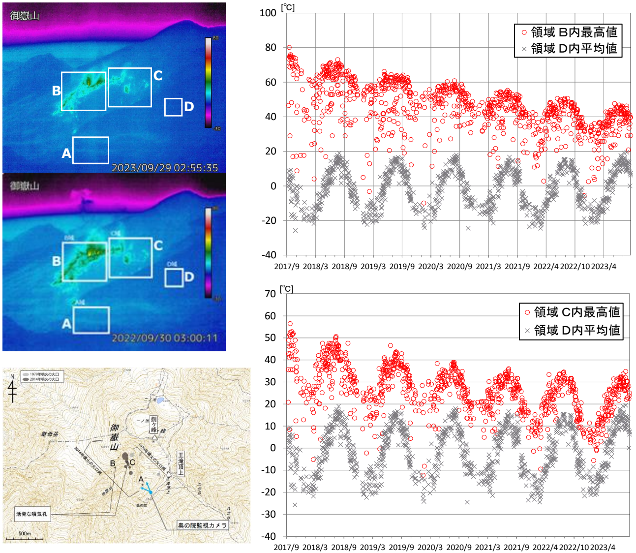
図3 御嶽山 奥の院赤外熱映像カメラによる剣ヶ峰南西側における最高温度の推移 (2017年9月13日～2023年9月30日)
