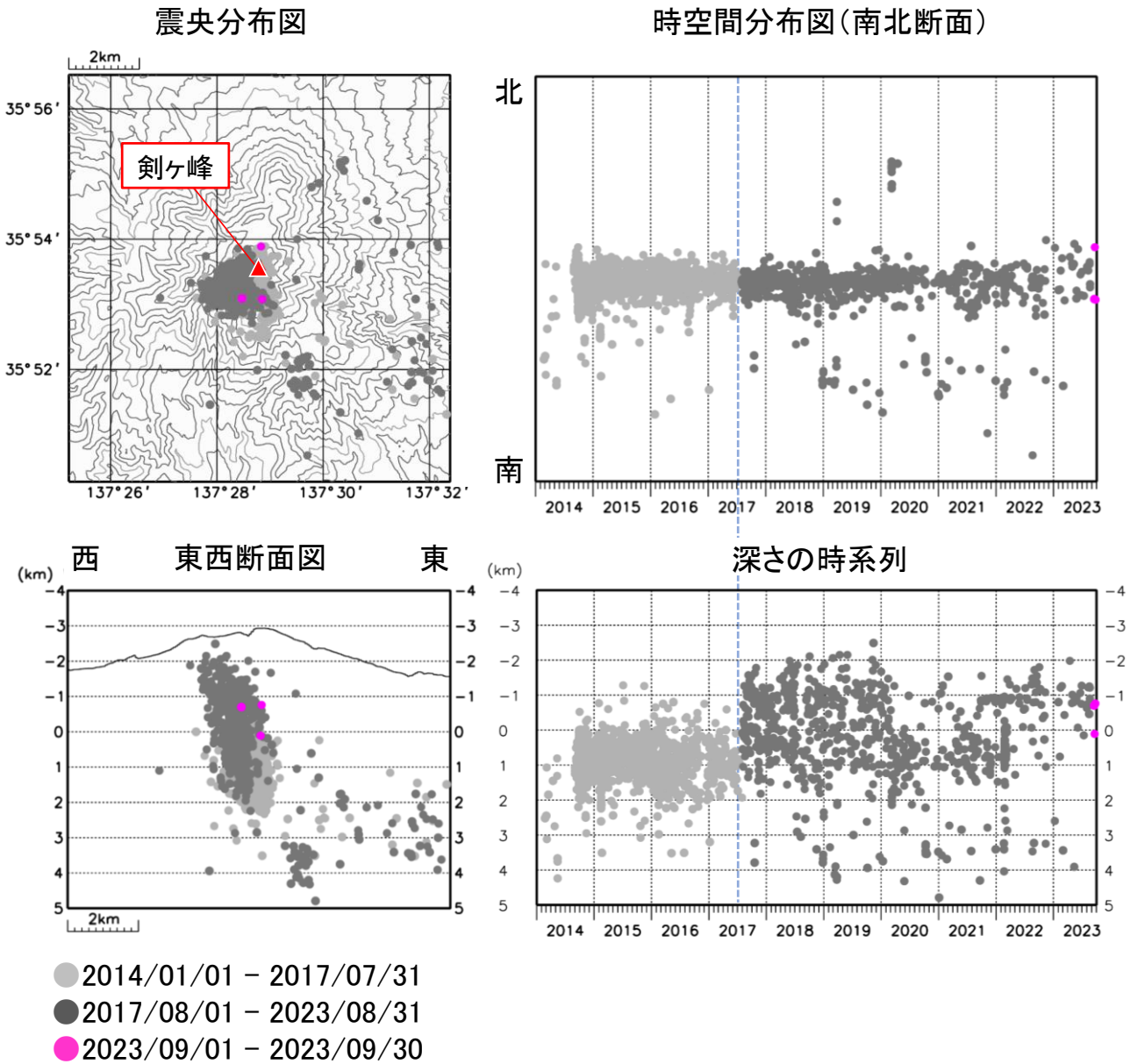
図4 御嶽山 震源分布図（2014年1月1日～2023年9月30日） 2017年8月1日（水色破線）以降の震源分布は、震源計算に使用する観測点を新たに追加して再計算したものを示しています。
