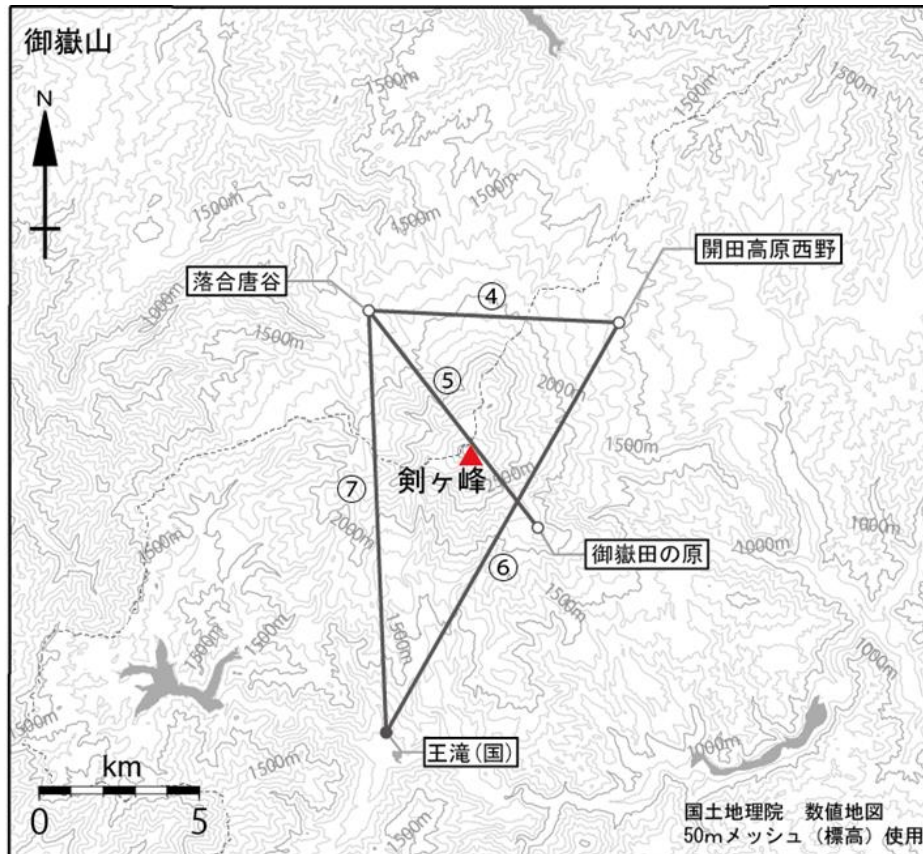
図5 御嶽山 GNSS 連続観測点と基線番号 白丸（○）は気象庁、黒丸（●）は気象庁以外の機関の観測点位置を示しています。 （国）：国土地理院 図中のGNSS基線④～⑦は図1の④～⑦にそれぞれ対応しています。
