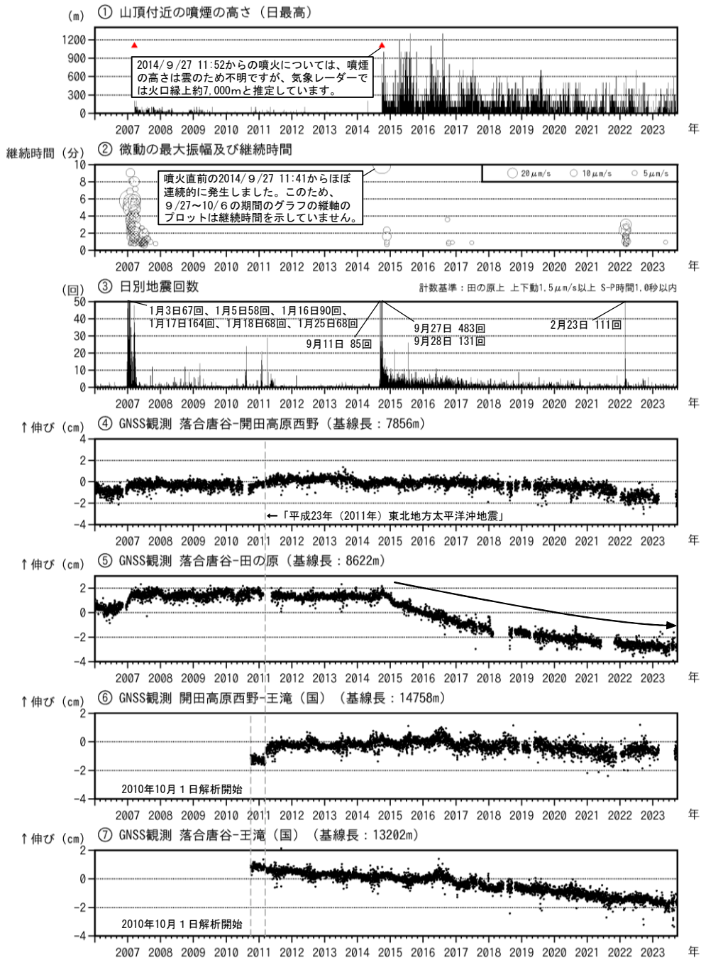
図1 御嶽山 長期間の火山活動経過図（2006年1月1日～2023年9月30日）
