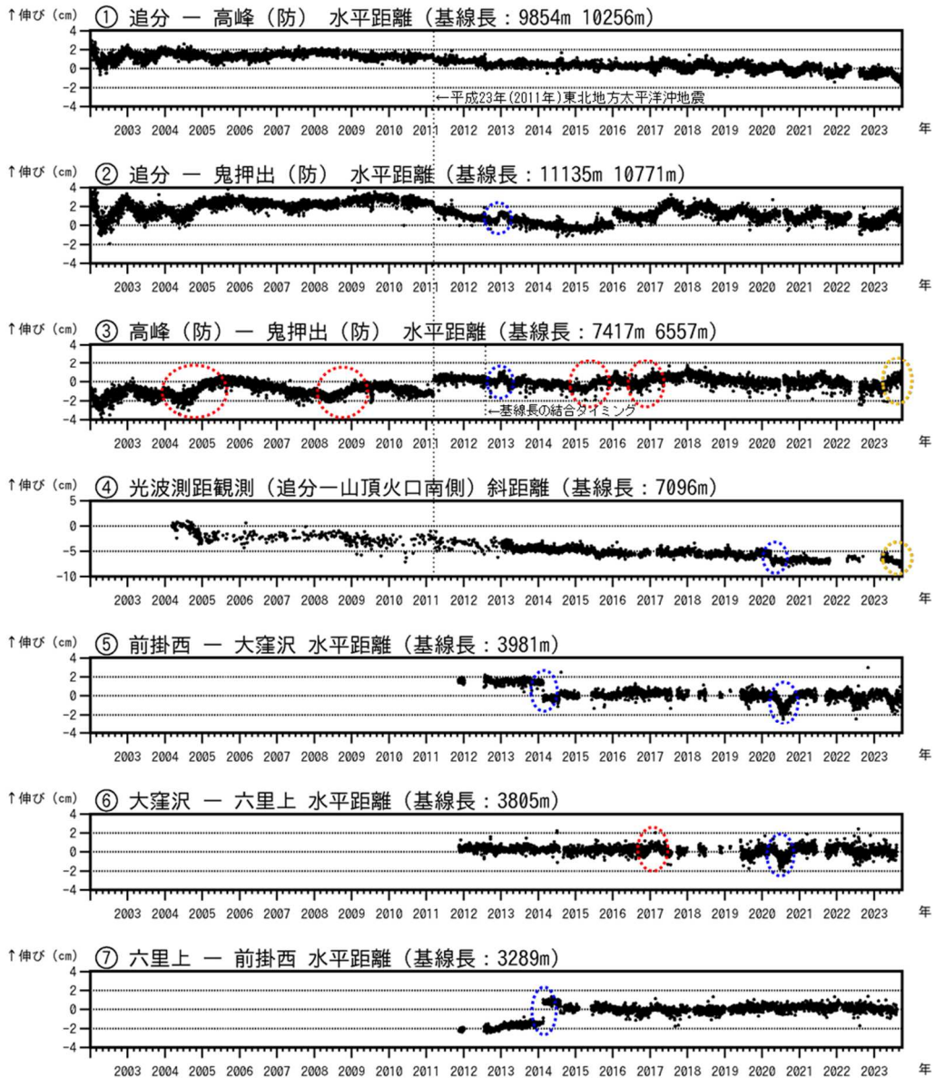
図6-1 浅間山 GNSS 連続観測及び光波測距観測の結果(2002年1月1日~2023年9月30日)
