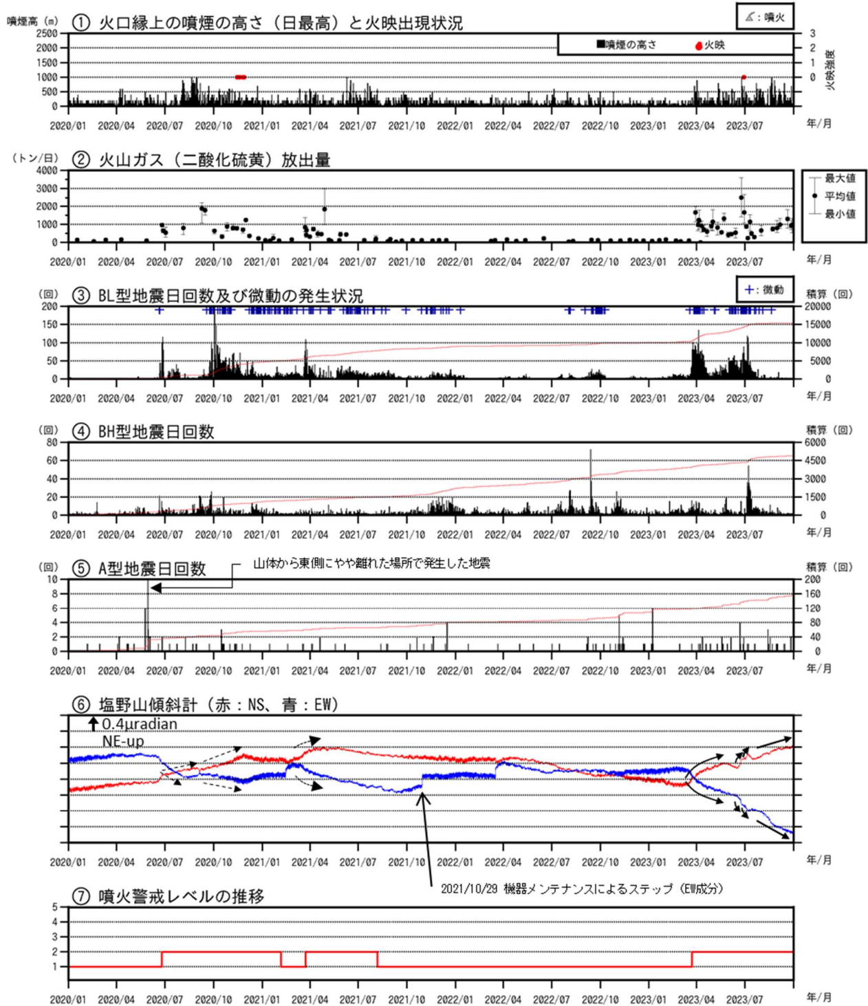
図3 浅間山 火山活動経過図（2020年1月1日～2023年9月30日）
