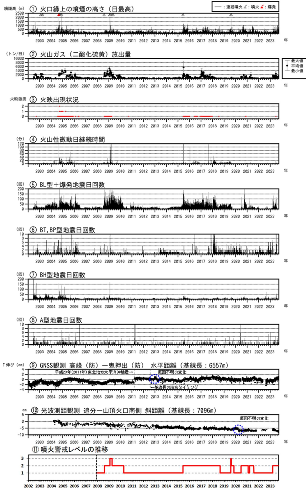
図4 浅間山 火山活動経過図（2002年1月1日～2023年9月30日）
