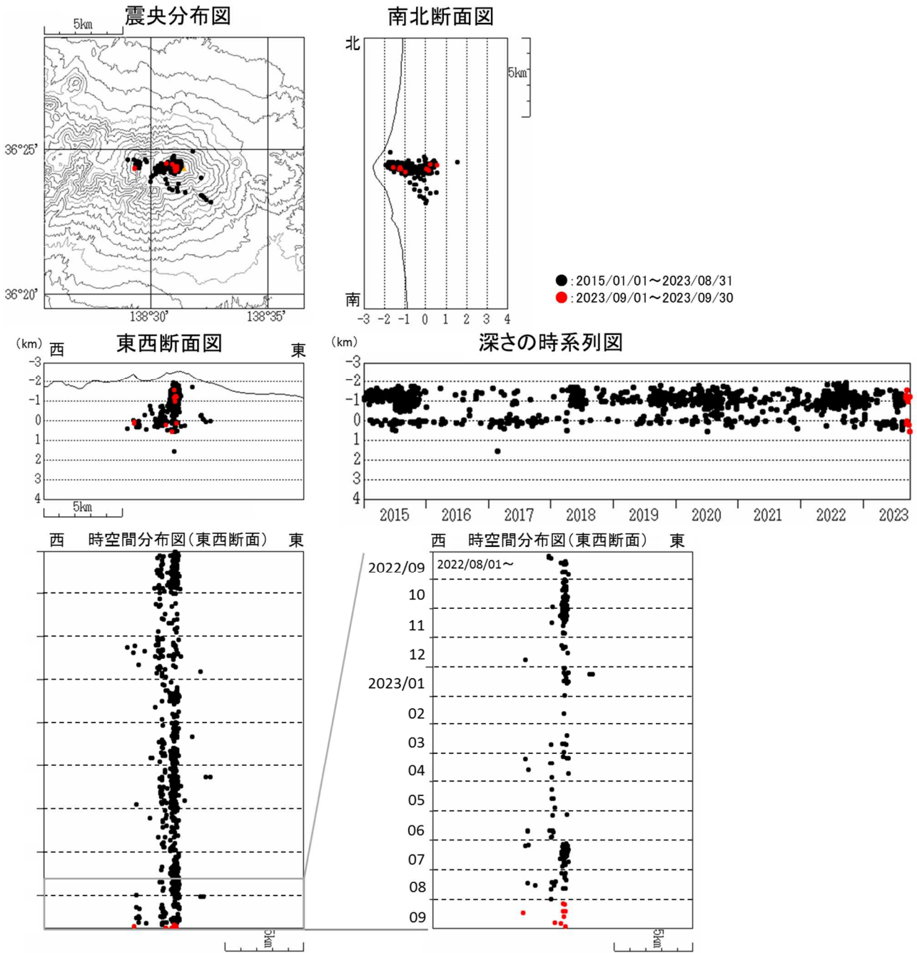
図5 浅間山 震源分布図 (2015年1月1日~2023年9月30日)
