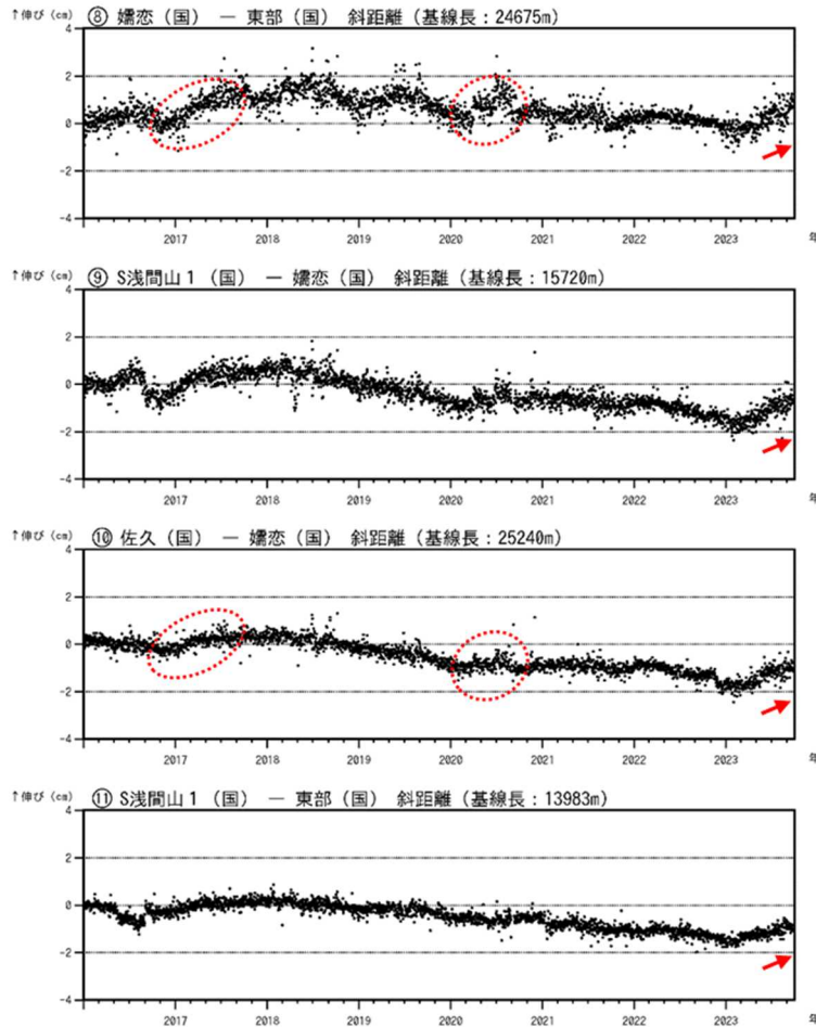
図6-2 浅間山 GNSS 連続観測結果(2016年1月1日~2023年9月30日) ⑧⑨⑩⑪は図7の⑧⑨⑩⑪にそれぞれ対応しています。空白部分は欠測を示します。(国)：国土地理院。
