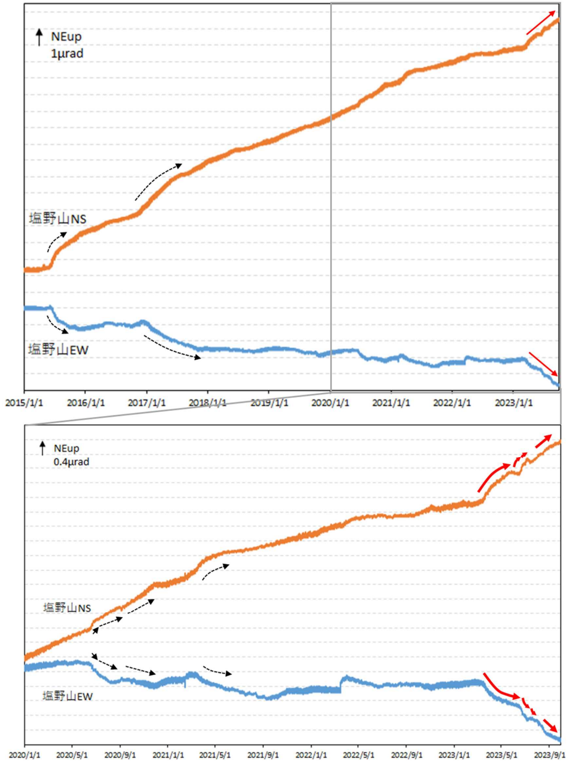
図8 浅間山 塩野山観測点における傾斜データ（2015年1月1日～2023年9月30日） データは時間平均値を使用しており、長期にわたるトレンドを補正しています。 下段は上段に比べて縦軸を拡大しています。
