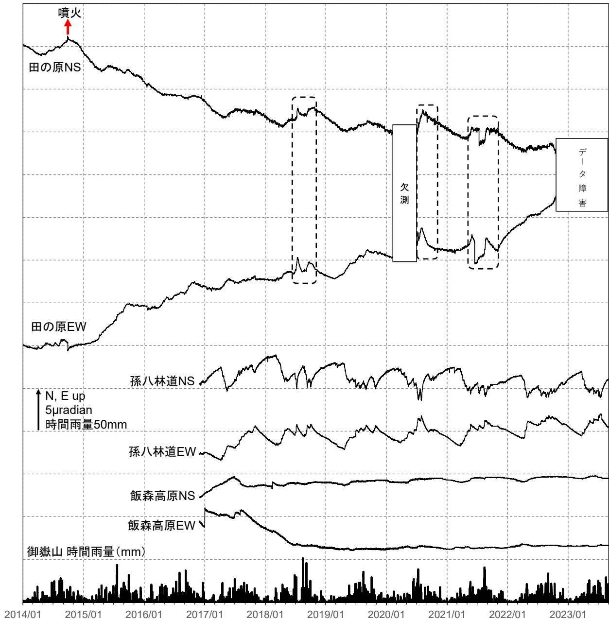
図4 御嶽山 傾斜変動（2014年1月1日～2023年8月31日）
