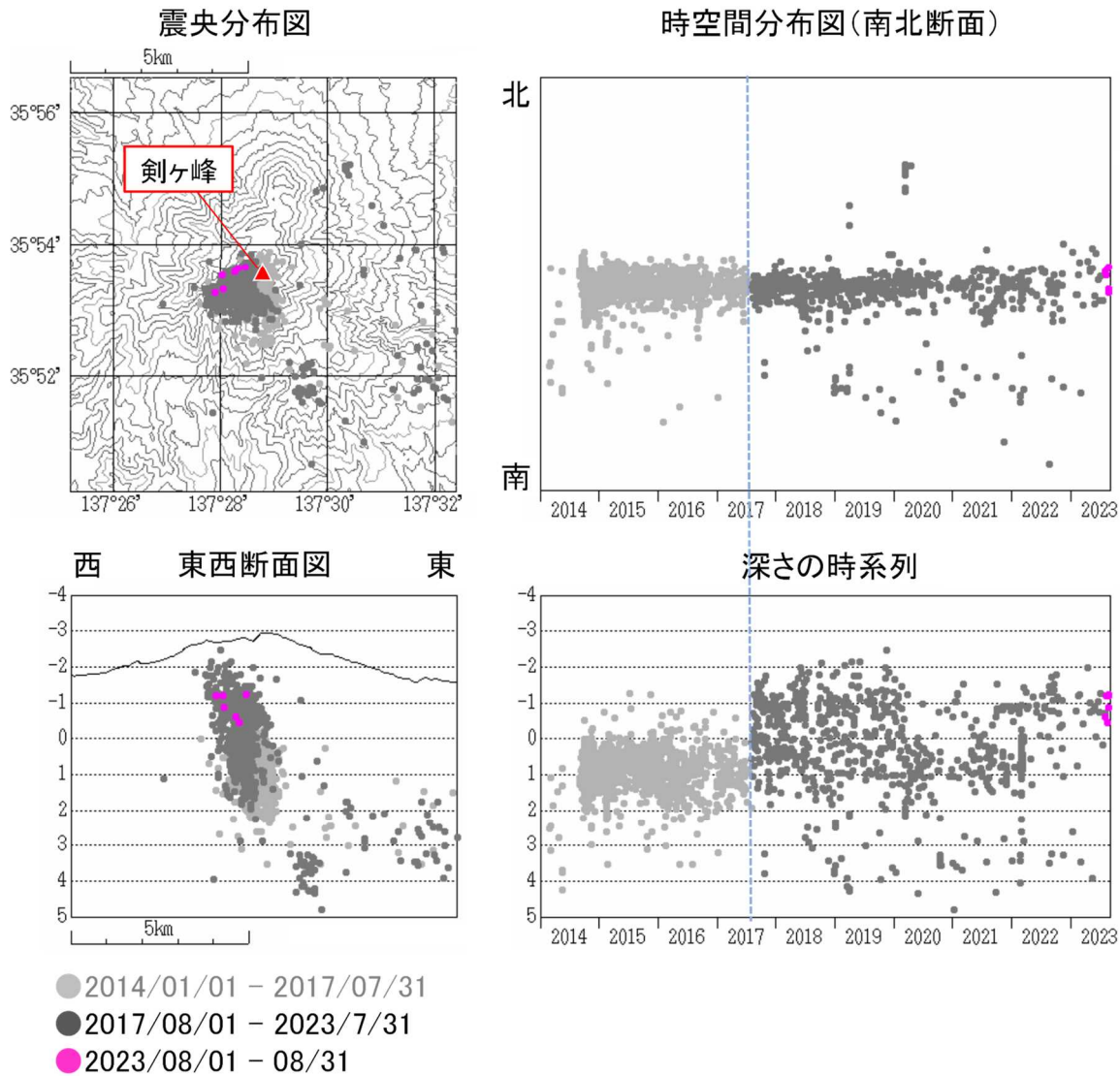
図2 御嶽山 震源分布図（2014年1月1日～2023年8月31日） 2017年8月1日（水色破線）以降の震源分布は、震源計算に使用する観測点を新たに追加して再計算したものを示しています。 観測点の稼働状況により、求まる震源の数の減少や位置の精度低下が生じる場合があります。
