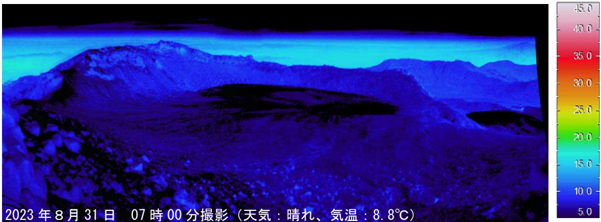
図7-2 御嶽山 一ノ池及び二ノ池の可視画像及び赤外熱映像装置による地表面温度分布 観測位置及び撮影方向は図7-1に示しています。
