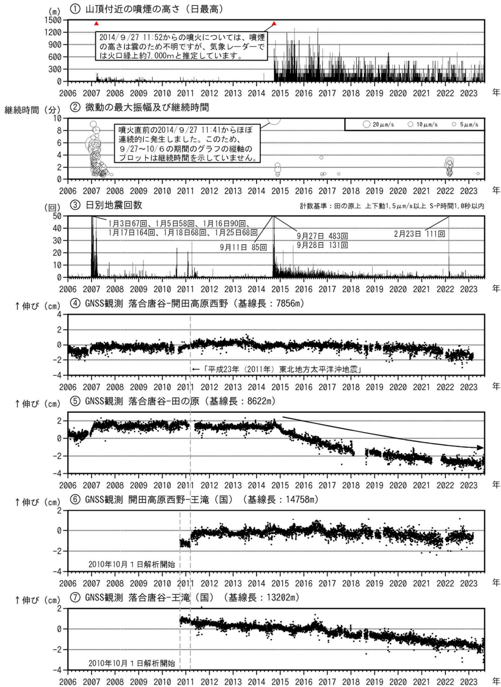
図1 御嶽山 長期間の火山活動経過図（2006年1月1日～2023年8月31日）
