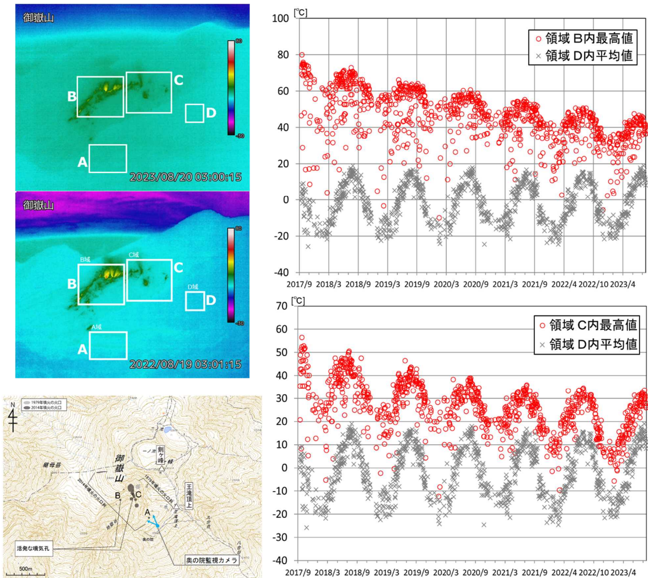
図6 御嶽山 奥の院赤外熱映像カメラによる剣ヶ峰南西側における最高温度の推移 (2017年9月13日～2023年8月31日)
