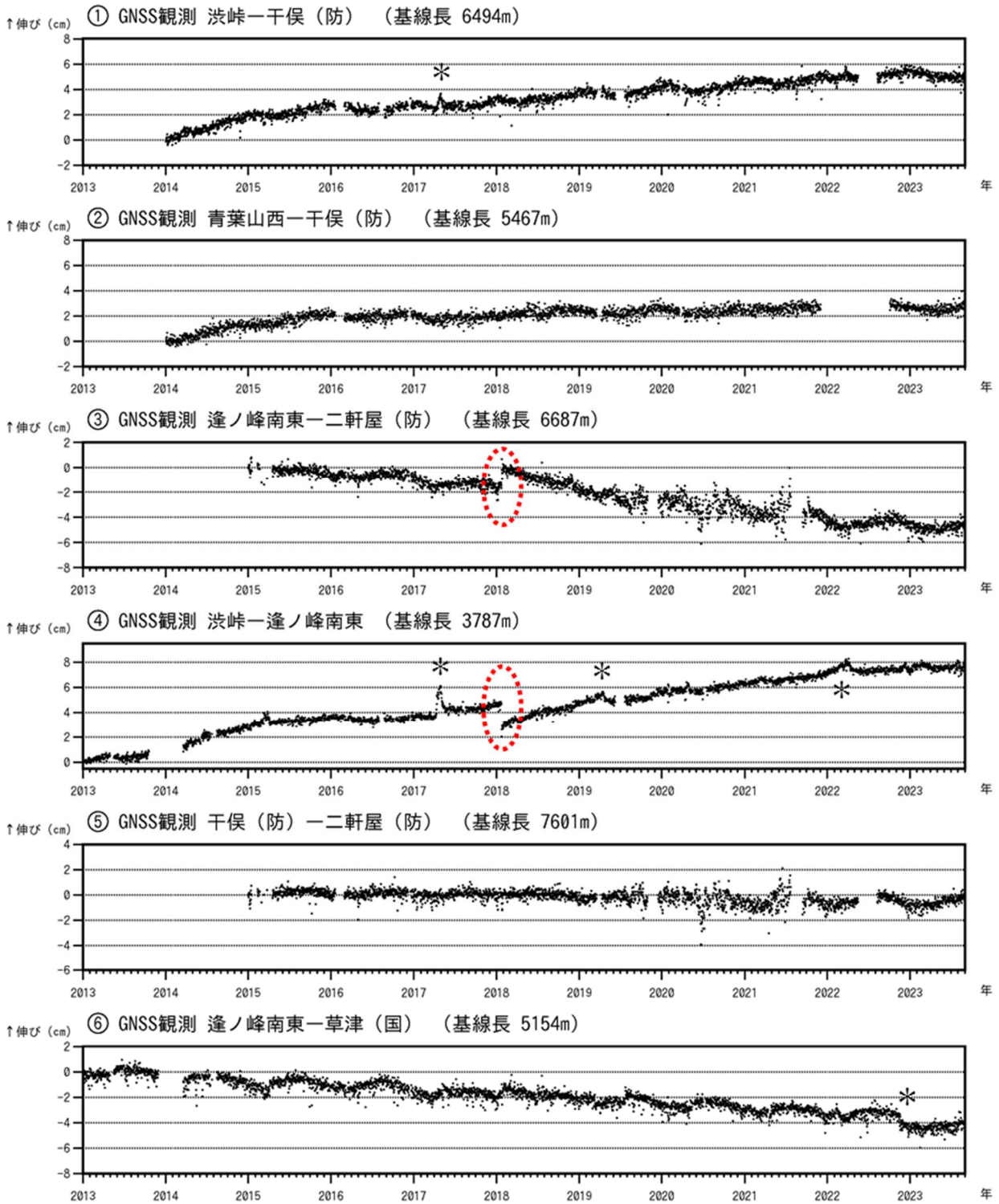
図6 草津白根山 GNSS連続観測の結果（2013年1月1日～2023年8月31日）
