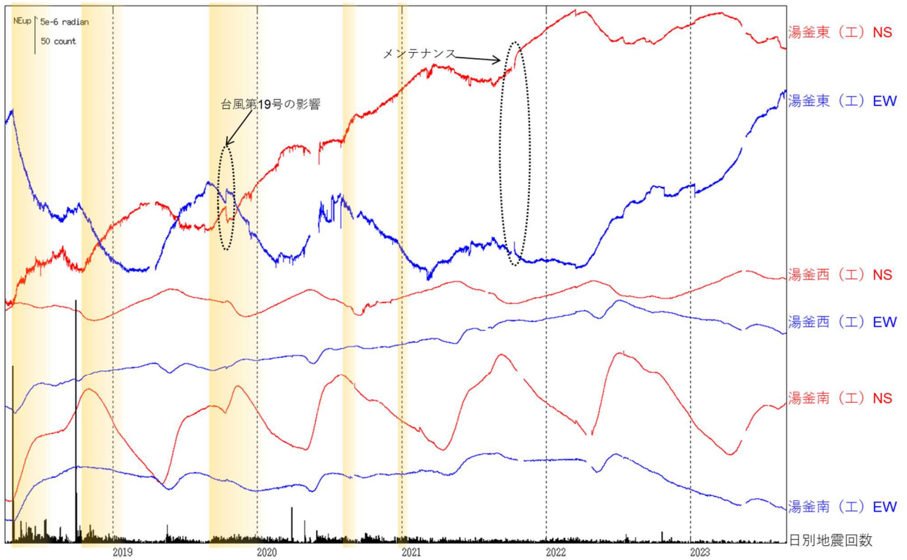
図5 草津白根山（白根山（湯釜付近）） 傾斜変動（2018年4月1日～2023年8月31日）
