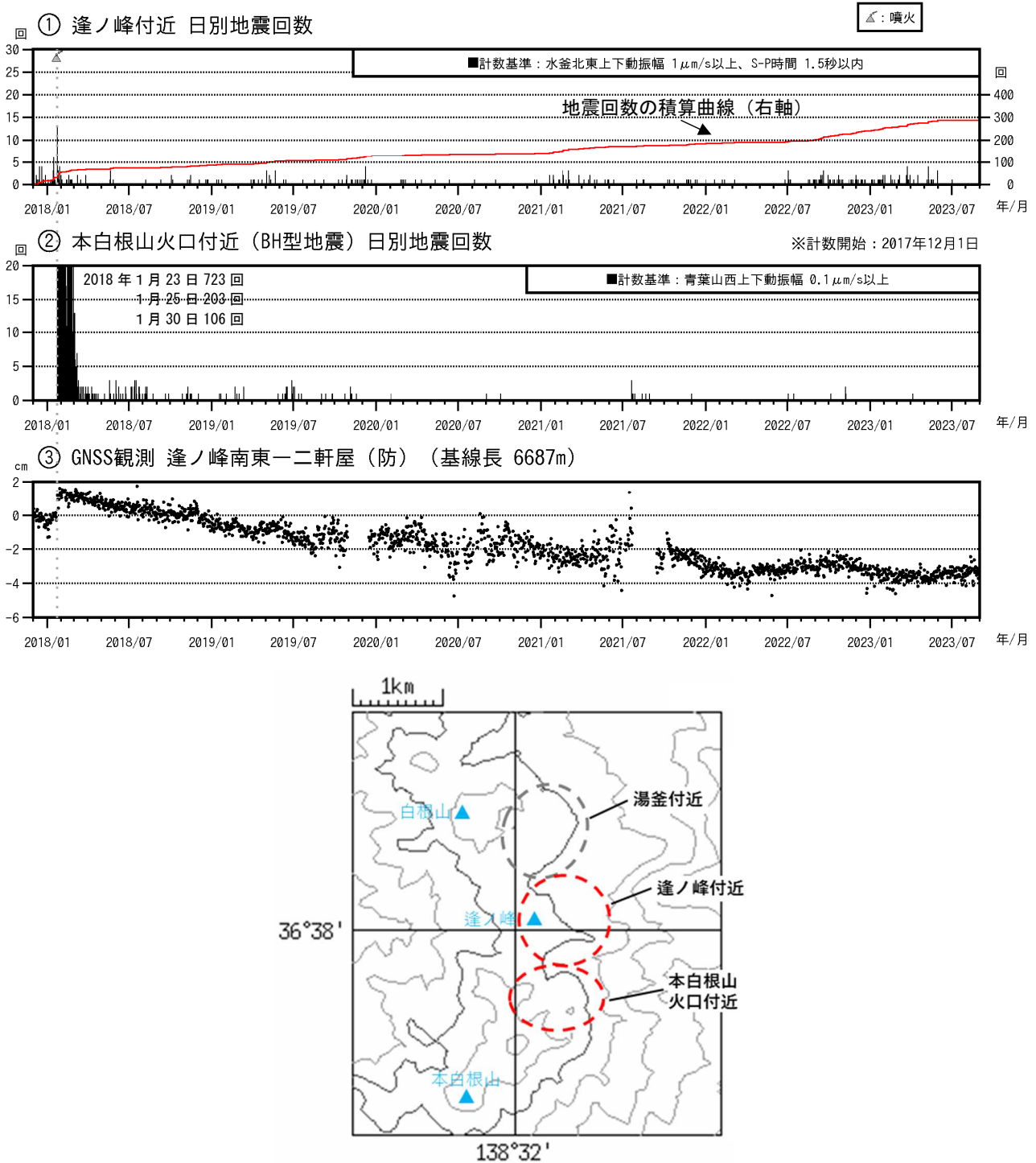
図 13 草津白根山（本白根山） 火山活動経過図（2017年12月1日～2023年8月31日） 草津白根山では、火山性地震はその発生領域から、「湯釜付近」、「逢ノ峰付近」、「本白根山火口付近」に分けています。本白根山の火山活動については、逢ノ峰付近と本白根山火口付近の地震活動に注目して監視しています。火山性地震の種類については図 14 を参照してください。 ③は図 7 の③の基線に対応しています。 最下段の図は、①②の地震の震源の概ねの位置を示しています。 ・逢ノ峰付近を震源とする火山性地震は、少ない状態で経過しました。 ・噴火発生後、本白根山火口付近でBH型の火山性地震が多発しましたが、2018年12月以降は、少ない状態で経過しています。なお、BH型地震は、初動が不明瞭なため、震源は求まっていません。 ・③の基線では、2018年1月の噴火に伴う変化が認められた後、2020年1月にかけて、噴火後の収縮によるものと考えられる変動がみられました。
