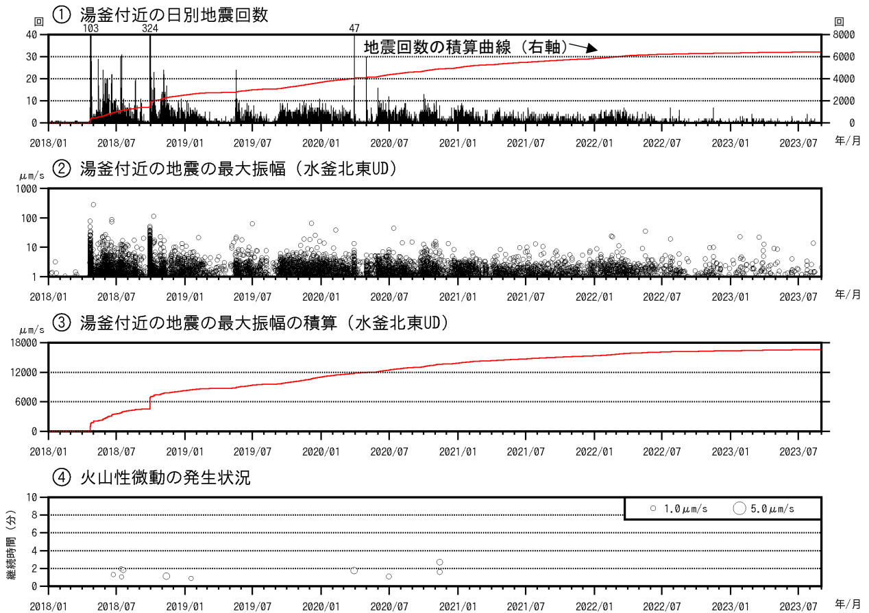
図1 草津白根山（白根山（湯釜付近）） 湯釜付近の地震活動及び火山性微動の発生状況 （2018年1月1日～2023年8月31日）
