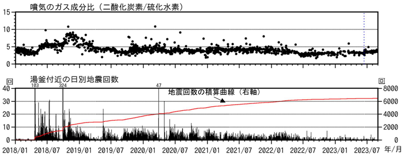
図8 草津白根山（白根山（湯釜付近）） 火山ガス観測結果（2018年1月～2023年8月）
