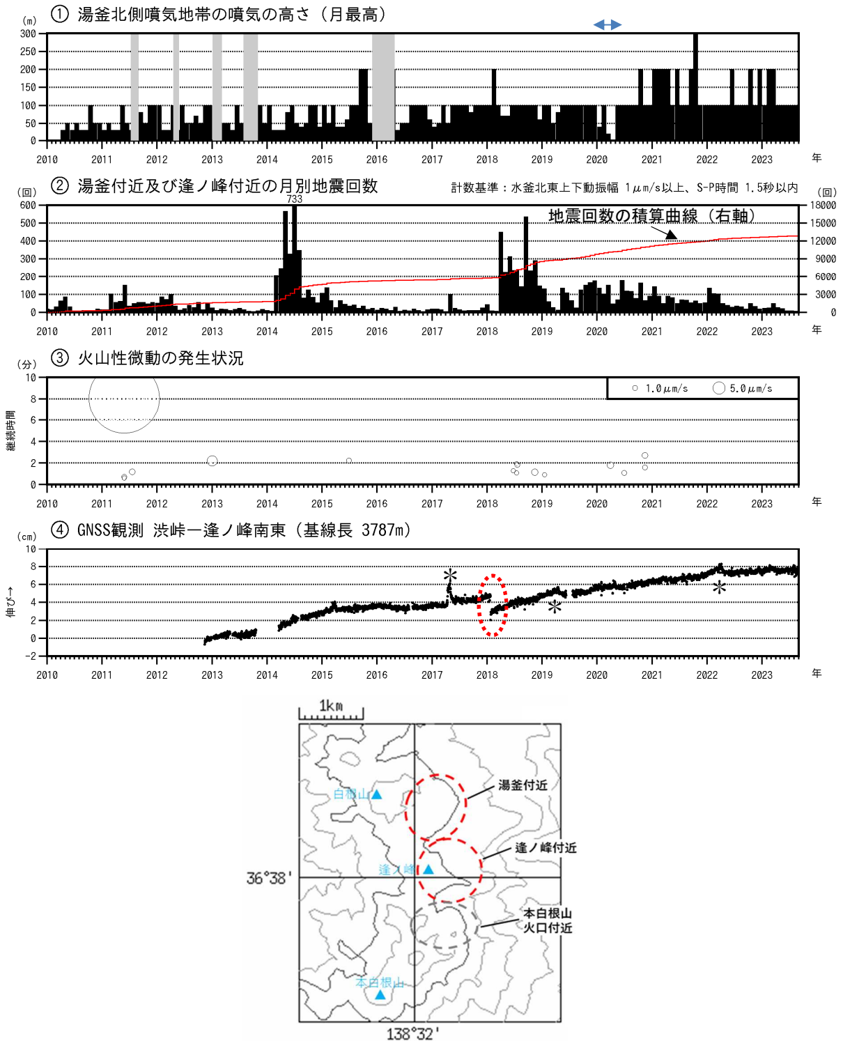
図3 草津白根山（白根山（湯釜付近））火山活動経過図（2010年1月1日～2023年8月31日）
