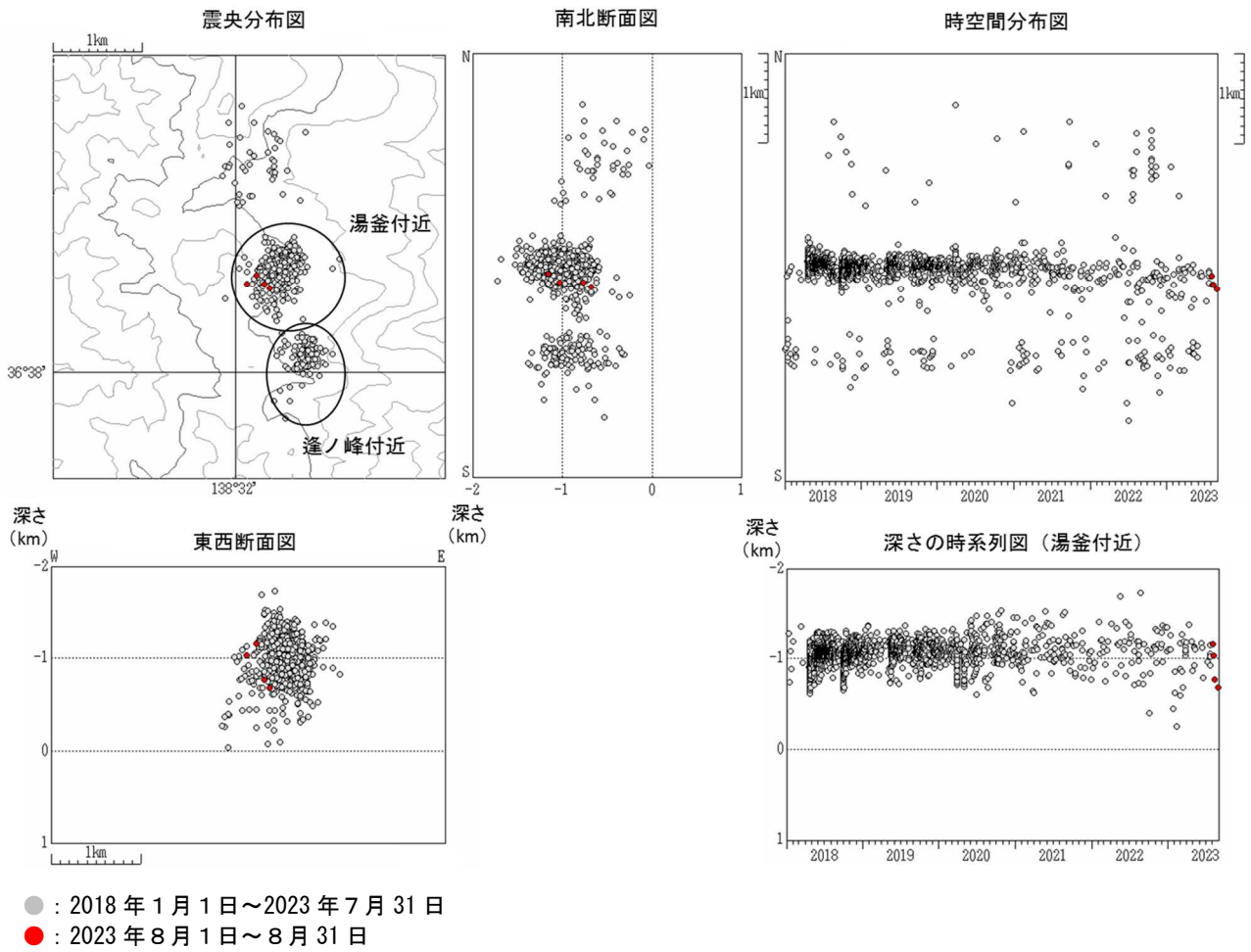
図4 草津白根山 震源分布図（2018年1月1日～2023年8月31日）
