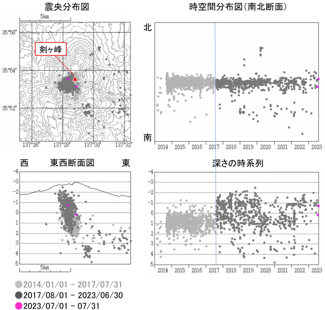
図2 御嶽山 震源分布図（2014年1月1日～2023年7月31日） 2017年8月1日（水色破線）以降の震源分布は、震源計算に使用する観測点を新たに追加して再計算したものを示しています。
