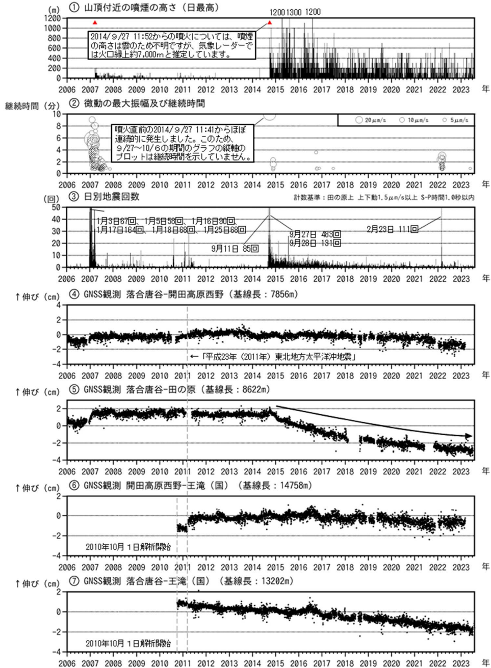
図1 御嶽山 長期間の火山活動経過図（2006年1月1日～2023年7月31日）
