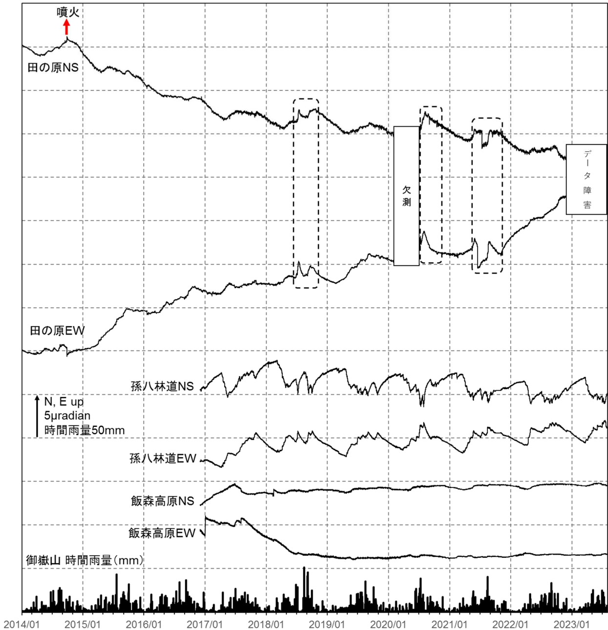
図4 御嶽山 傾斜変動（2014年1月1日～2023年7月31日）
