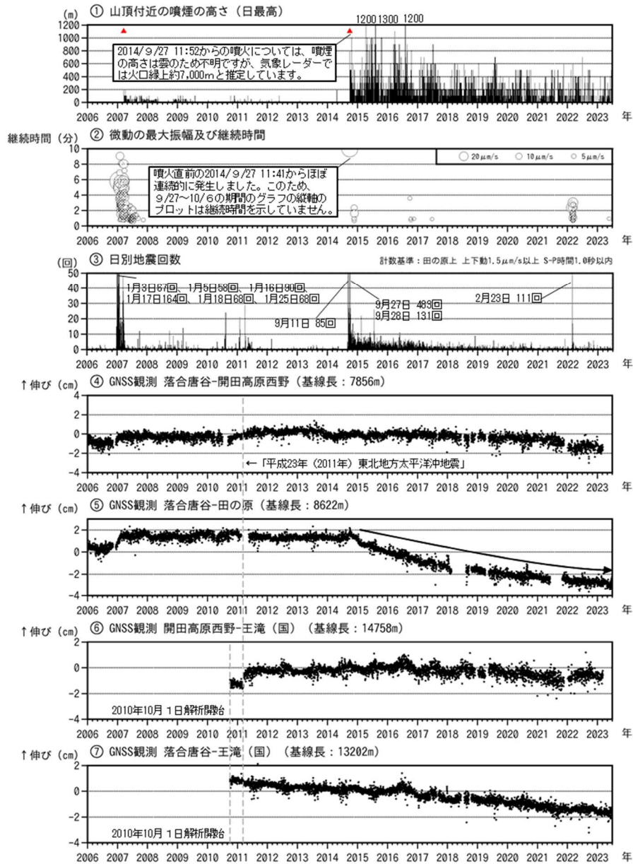
図1 御嶽山 長期間の火山活動経過図（2006年1月1日～2023年6月30日）
