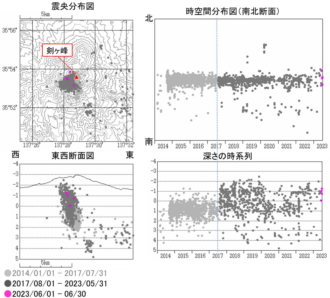
図2 御嶽山 震源分布図（2014年1月1日～2023年6月30日） 2017年8月1日（水色破線）以降の震源分布は、震源計算に使用する観測点を新たに追加して再計算したものを示しています。 観測点の稼働状況により、求まる震源の数の減少や位置の精度低下が生じる場合があります。
