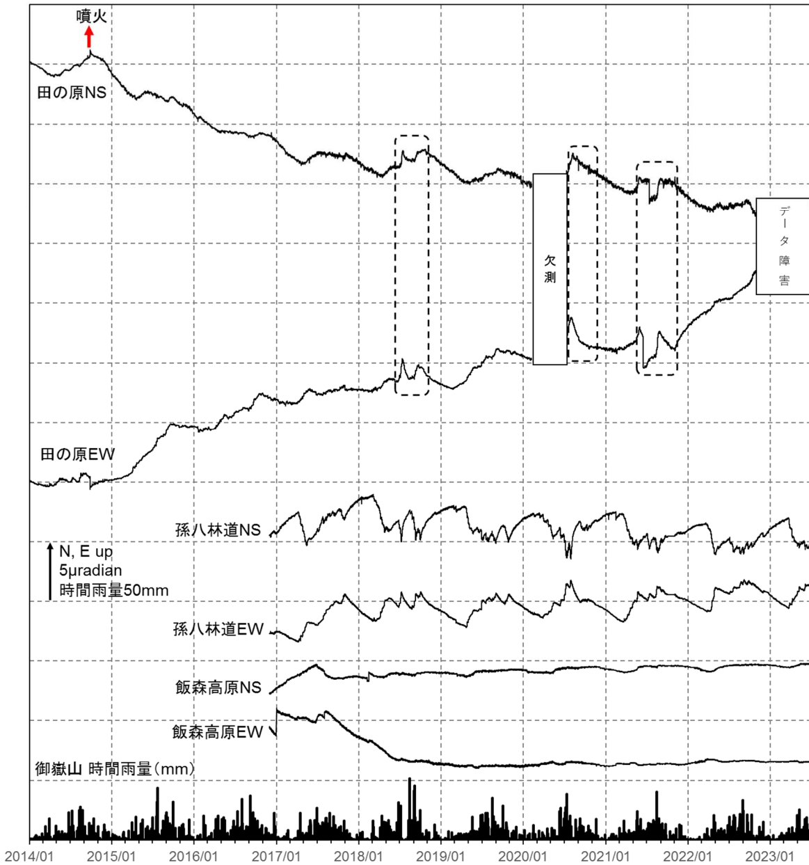
図4 御嶽山 傾斜変動（2014年1月1日～2023年6月30日）
