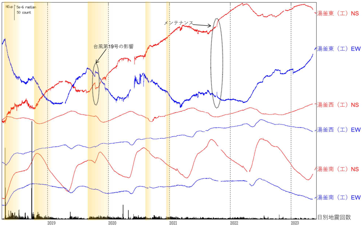
図5 草津白根山（白根山（湯釜付近）） 傾斜変動（2018年4月1日～2023年5月31日）
