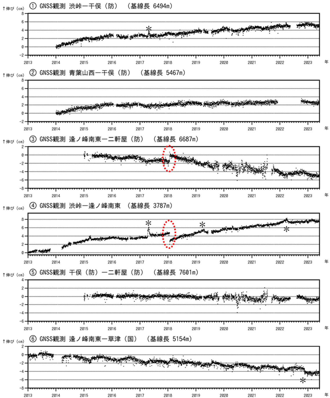
図6 草津白根山 GNSS 連続観測の結果（2013年1月1日～2023年5月31日）
