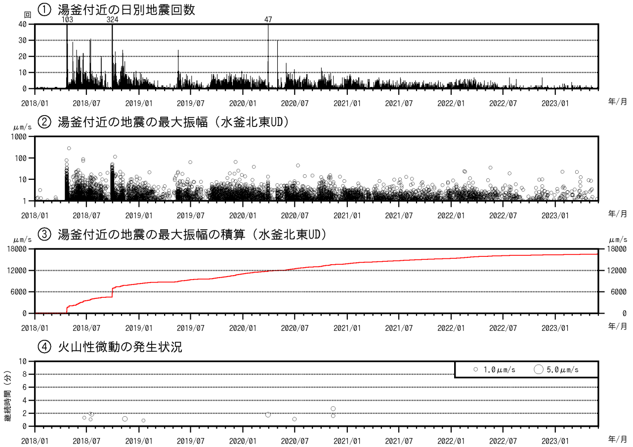
図1 草津白根山（白根山（湯釜付近）） 湯釜付近の地震活動及び火山性微動の発生状況 （2018年1月1日～2023年5月31日） ・湯釜付近を震源とする火山性地震は、少ない状態で経過しました。
