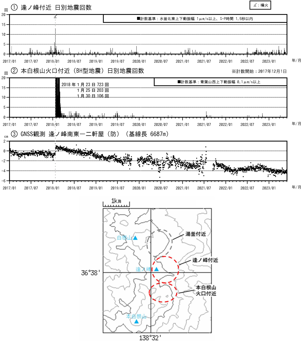
図13 草津白根山（本白根山） 火山活動経過図（2017年1月1日～2023年5月31日） 草津白根山では、火山性地震はその発生領域から、「湯釜付近」、「逢ノ峰付近」、「本白根山火口付近」に分けています。本白根山の火山活動については、逢ノ峰付近と本白根山火口付近の地震活動に注目して監視しています。火山性地震の種類については図14を参照してください。 ③は図7の③の基線に対応しています。 最下段の図は、①②の地震の震源の概ねの位置を示しています。 ・逢ノ峰付近の火山性地震は、少ない状態で経過しました。 ・噴火発生後、本白根山火口付近でBH型の火山性地震が多発しましたが、2018年12月以降は、少ない状態で経過しています。なお、BH型地震は、初動が不明瞭なため、震源は求まっていません。 ・③の基線では、2018年1月の噴火に伴う変化が認められた後、2020年1月にかけて、噴火後の収縮によるものと考えられる変動がみられました。
