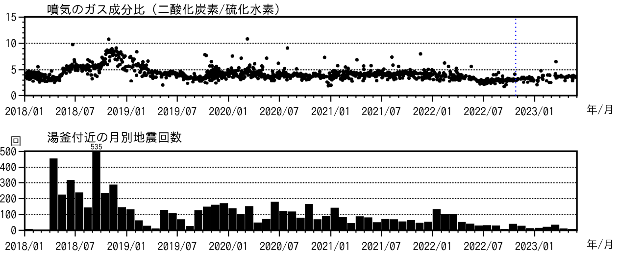
図8 草津白根山（白根山（湯釜付近）） 火山ガス観測結果（2018年1月～2023年5月）
