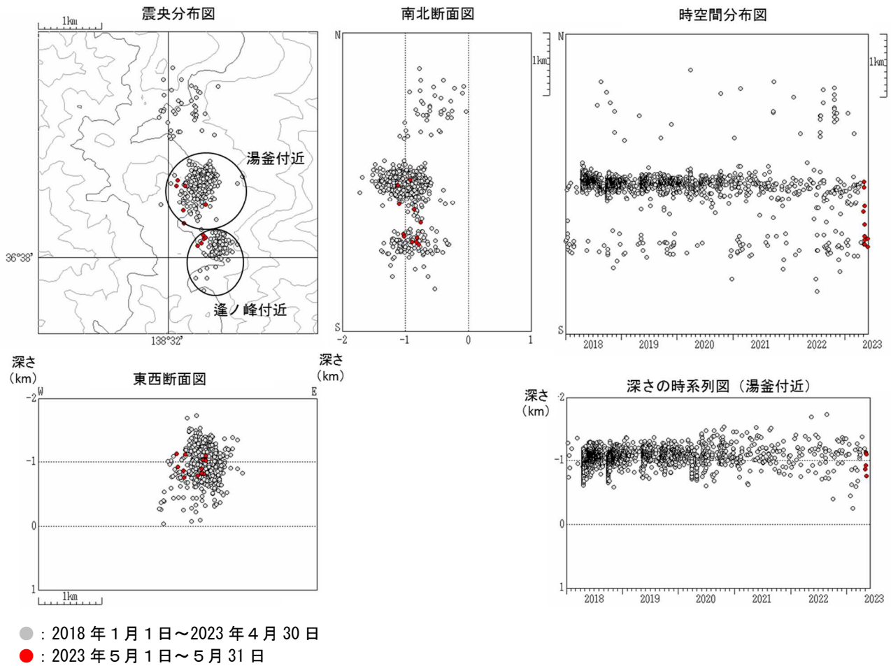
図4 草津白根山 震源分布図（2018年1月1日～2023年5月31日）
