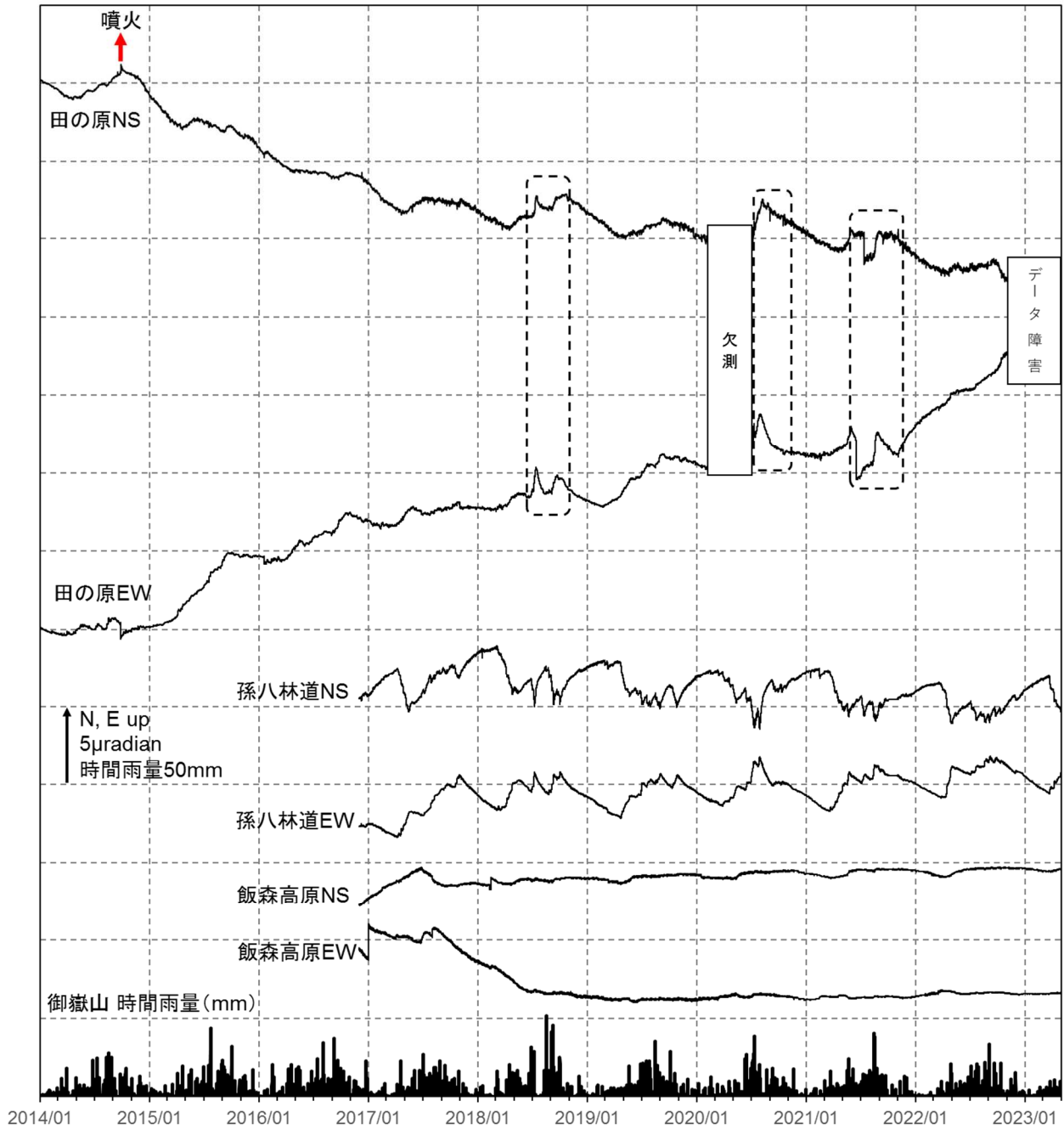
図4 御嶽山 傾斜変動（2014年1月1日～2023年4月30日） データは時間平均値、田の原及び孫八林道観測点のデータは潮汐補正済みです。 2018年7月頃及び2020年7月頃の破線で囲んだ部分は、降水による影響と考えられる変動を示します。 2021年6月頃の破線で囲んだ部分は、降水及び田の原観測点の近傍での建設工事の影響と考えられる変動を示します。
