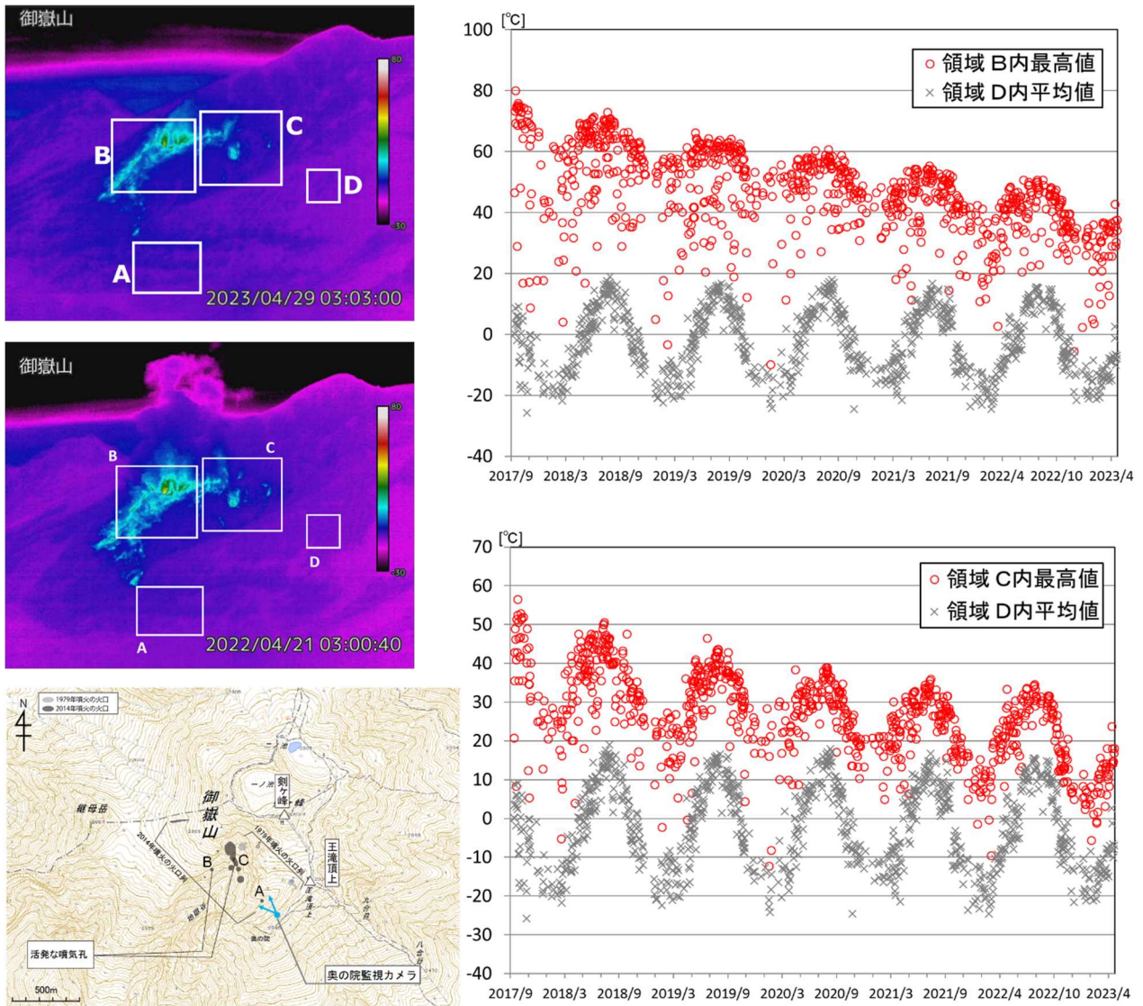
図6 御嶽山 奥の院赤外熱映像カメラによる剣ヶ峰南西側における最高温度の推移 (2017年9月13日～2023年4月30日)
