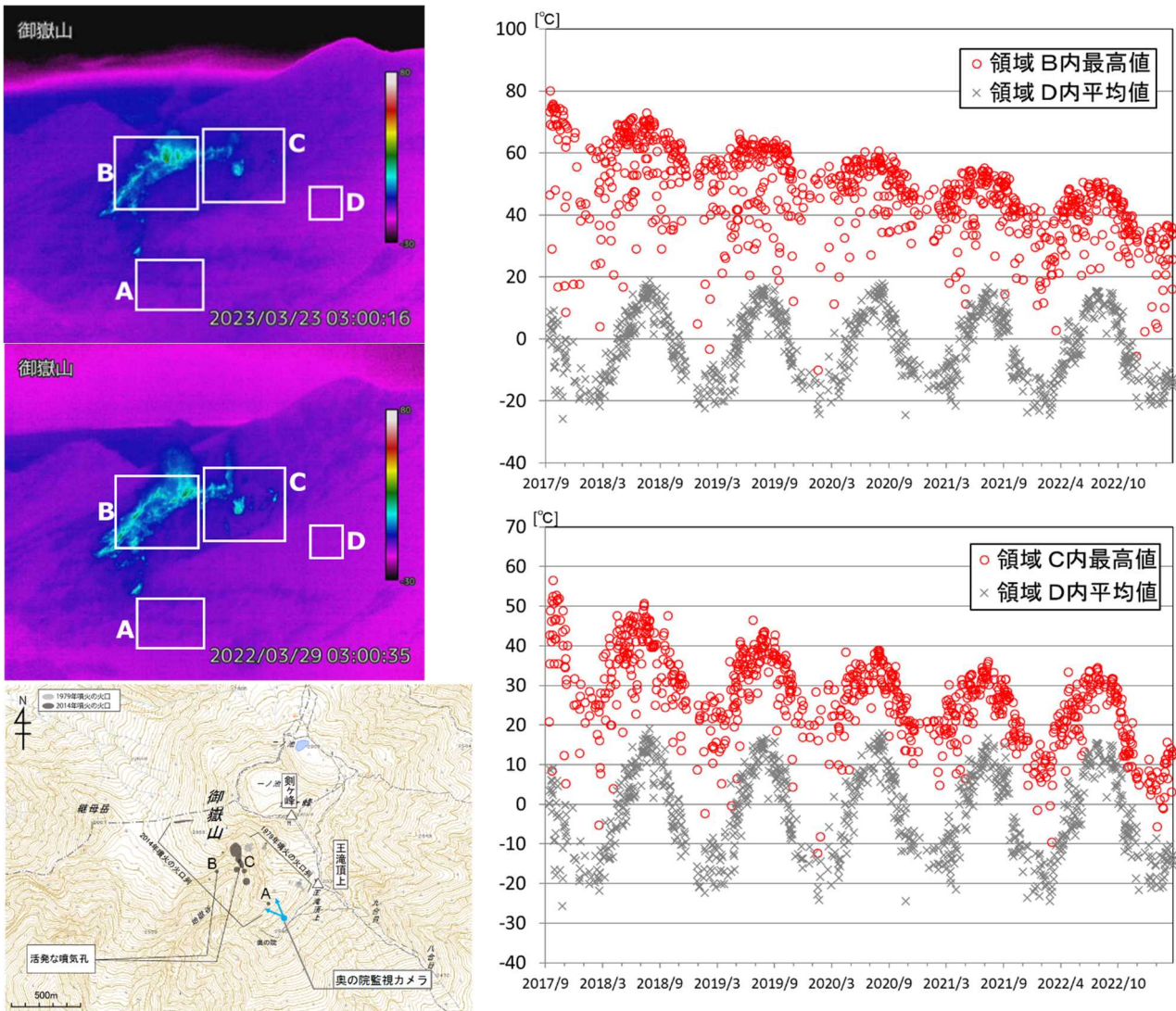
図6 御嶽山 奥の院赤外熱映像カメラによる剣ヶ峰南西側における最高温度の推移 (2017年9月13日～2023年3月31日)
