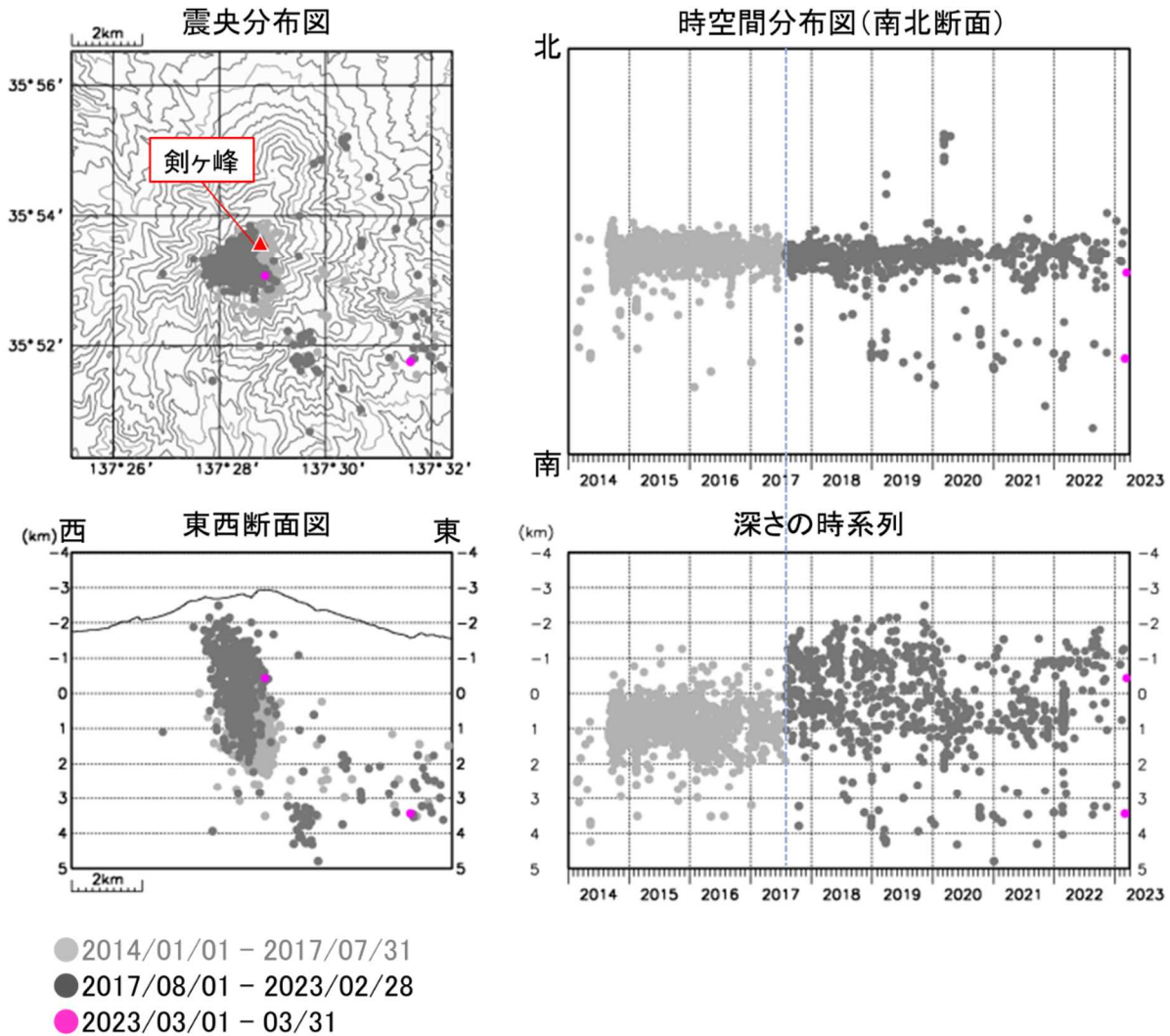
図2 御嶽山 震源分布図（2014年1月1日～2023年3月31日）
