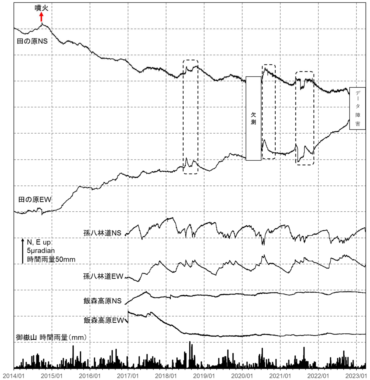
図4 御嶽山 傾斜変動（2014年1月1日～2023年3月31日）
