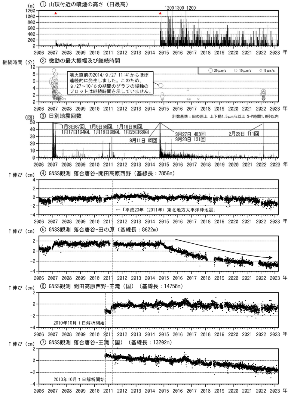
図1 御嶽山 長期間の火山活動経過図（2006年1月1日～2023年3月31日）
