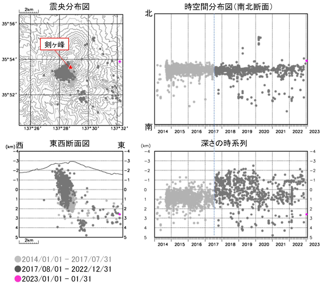
図2 御嶽山 震源分布図（2014年1月1日～2023年1月31日） 本火山活動解説資料（令和5年1月）より、2017年8月1日（水色破線）以降の震源分布は、震源計算に使用する観測点を新たに追加して再計算したものを示しています。 観測点の移動状況により、求まる震源の数の減少や位置の精度低下が生じる場合があります。
