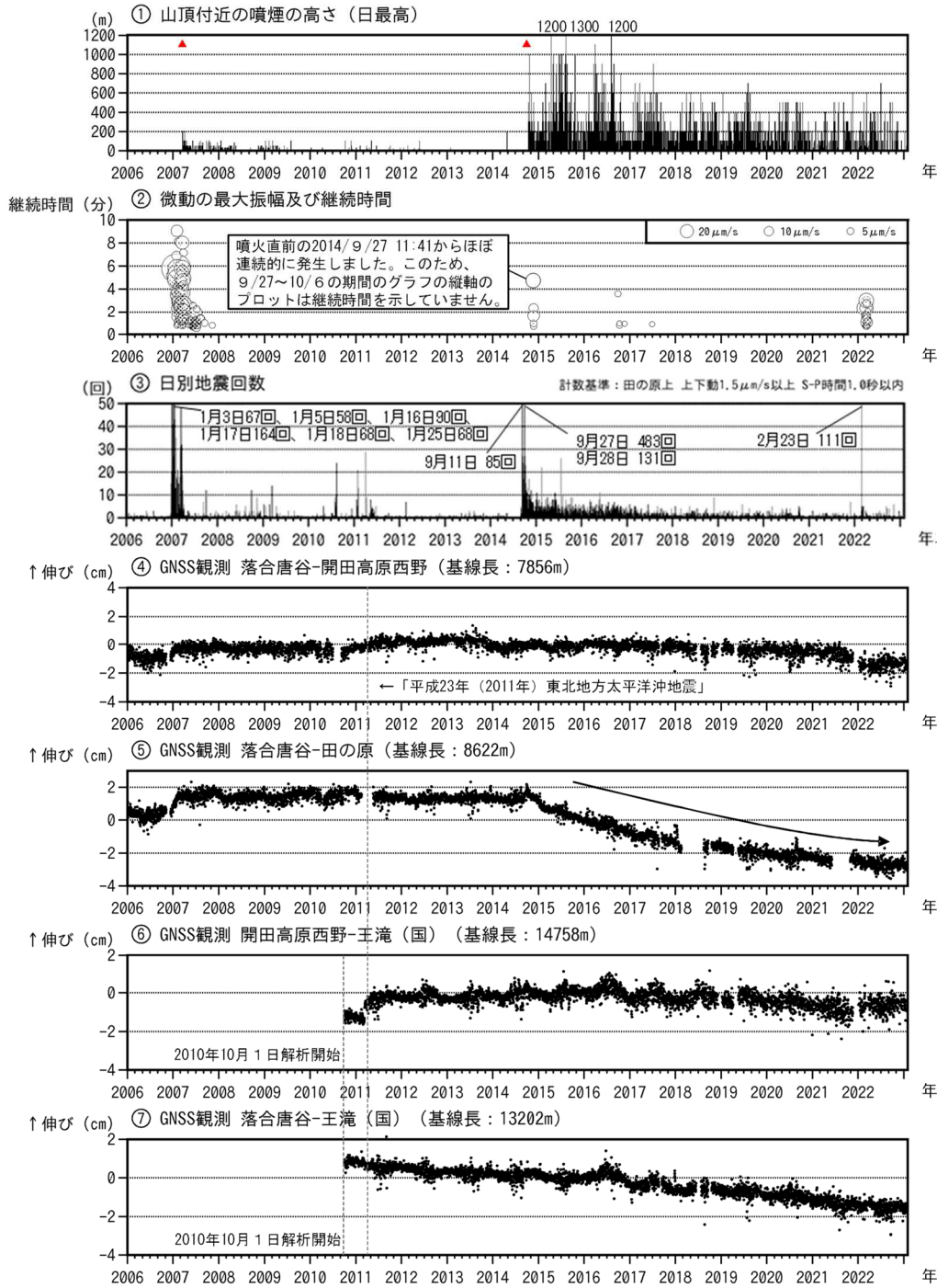
図1 御嶽山 長期間の火山活動経過図（2006年1月1日～2023年1月31日）
