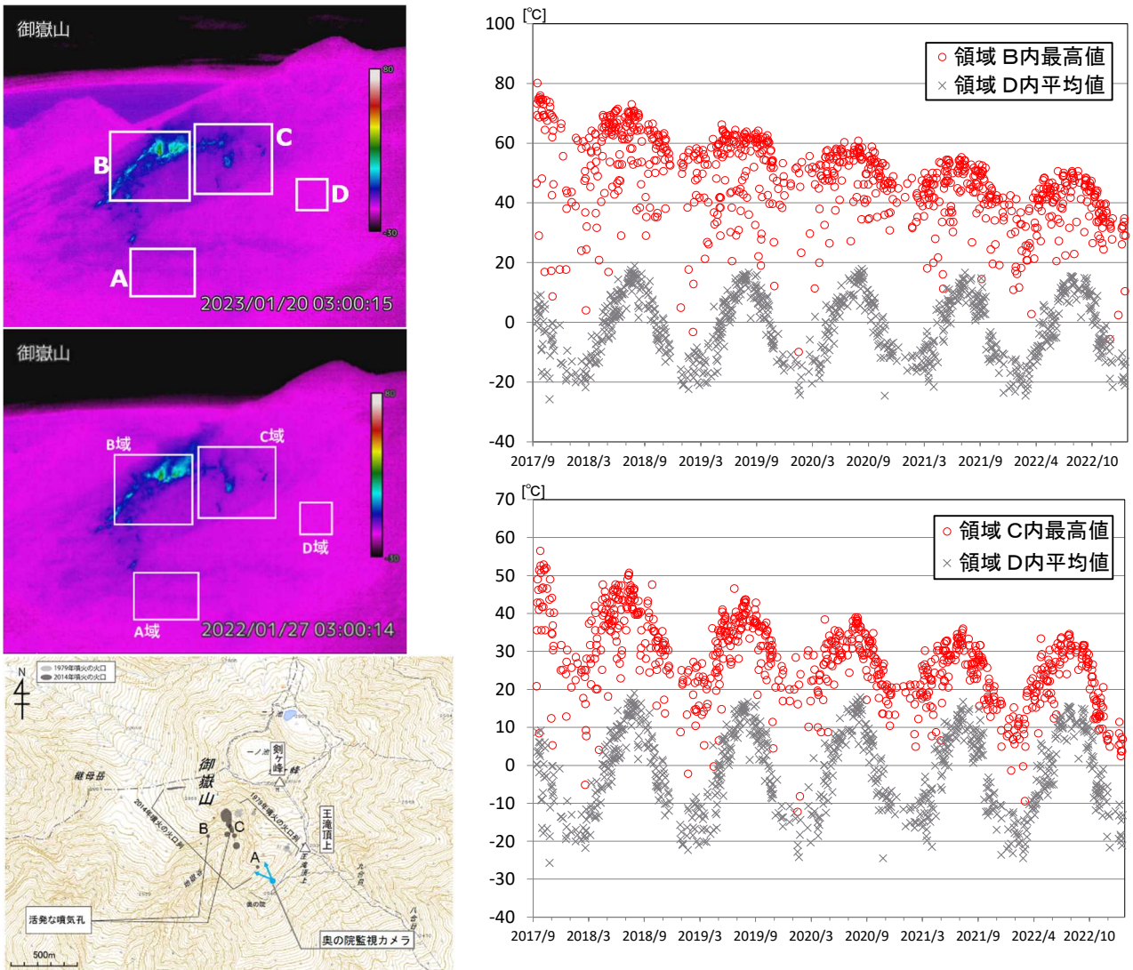
図6 御嶽山 奥の院赤外熱映像カメラによる剣ヶ峰南西側における最高温度の推移 (2017年9月13日～2023年1月31日)
