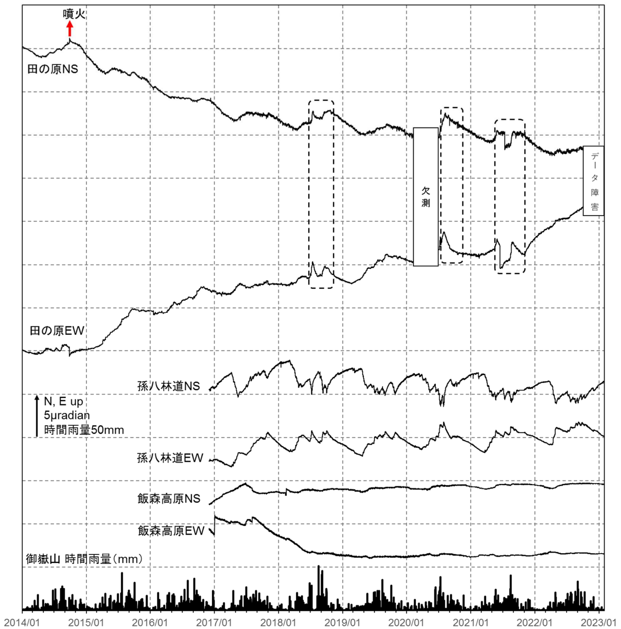
図4 御嶽山 傾斜変動（2014年1月1日～2023年1月31日）
