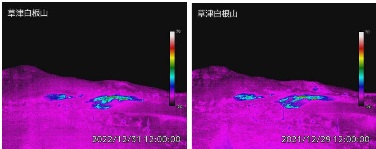
図2-2 草津白根山（白根山（湯釜付近））水釜北東2監視カメラによる湯釜火口北側噴気地帯の地熱域の分布状況
