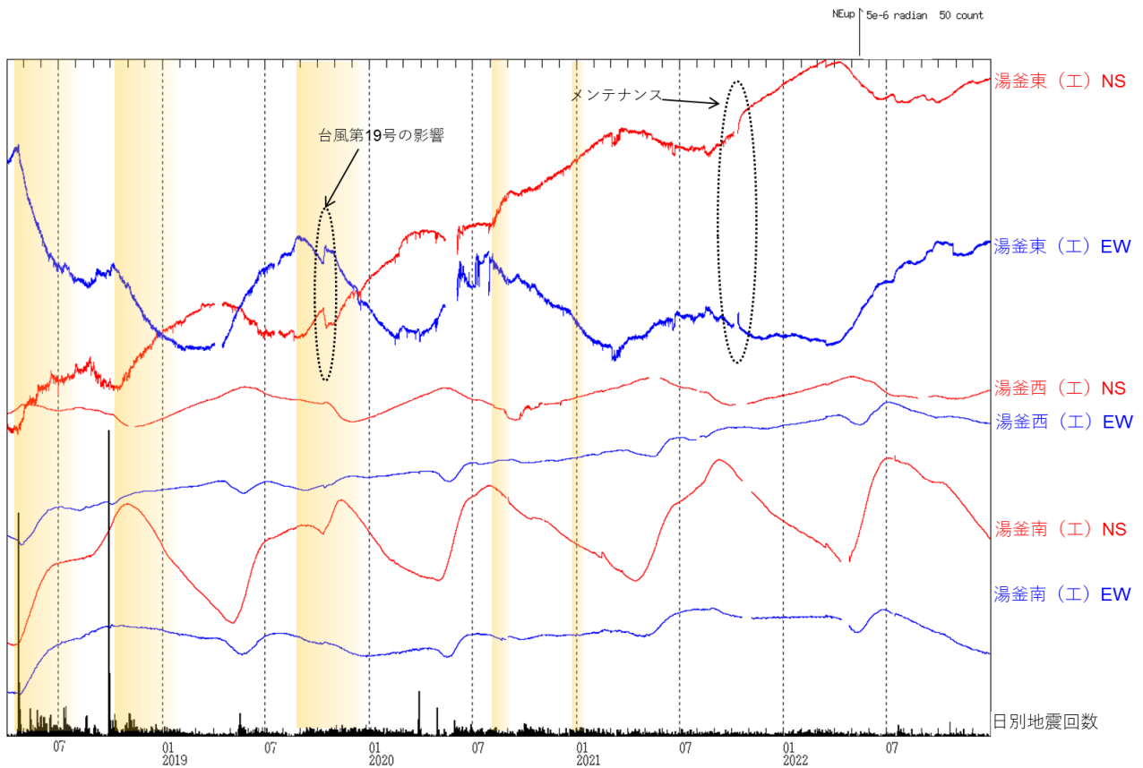
図5 草津白根山（白根山（湯釜付近）） 傾斜変動（2018年4月1日～2022年12月31日） （工）：東京工業大学
