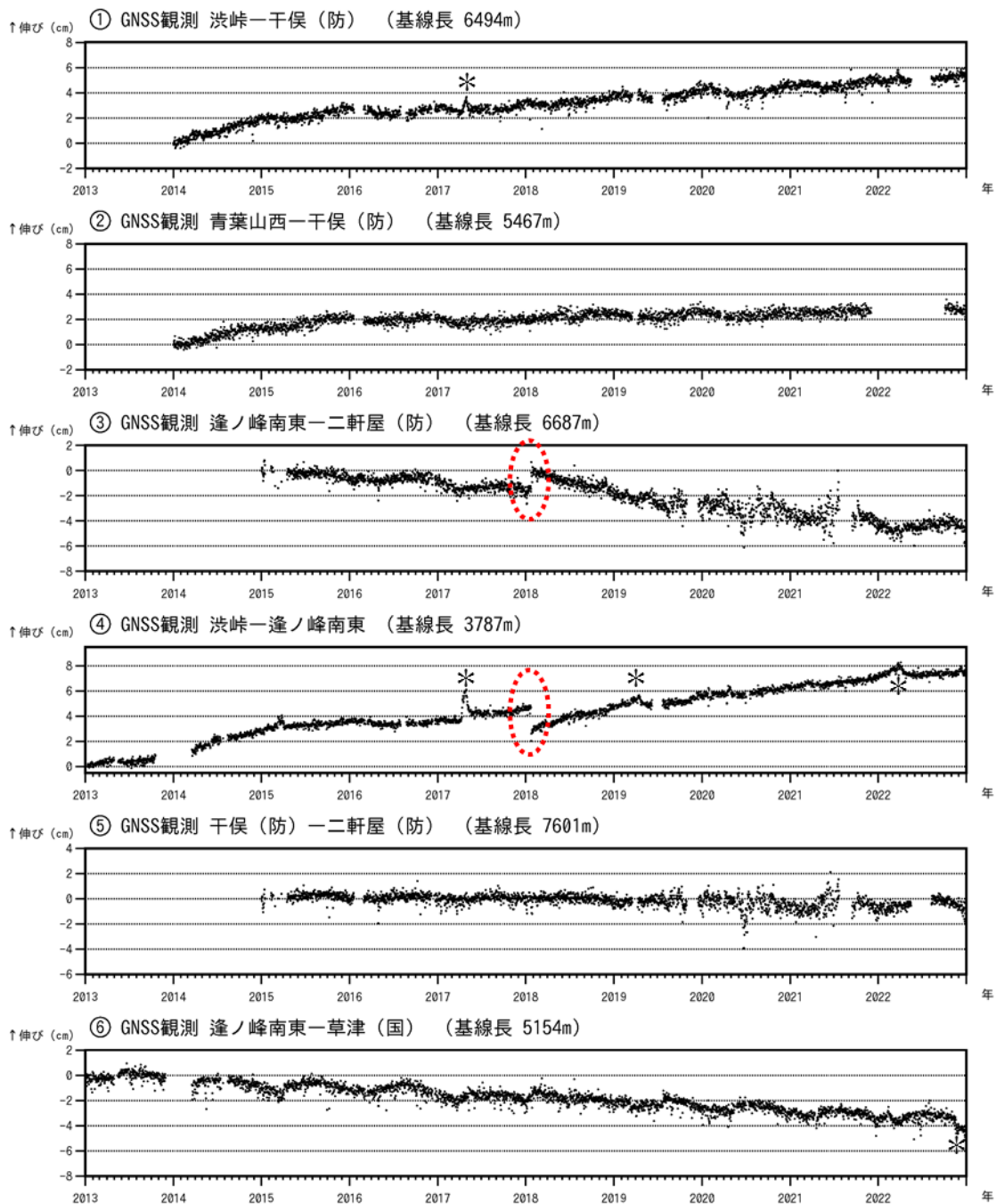
図6 草津白根山 GNSS 連続観測の結果（2013年1月1日～2022年12月31日）
