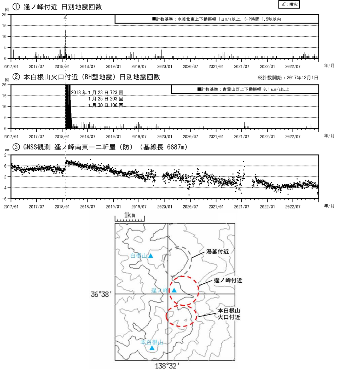
図12 草津白根山（本白根山） 火山活動経過図（2017年1月1日～2022年12月31日）
