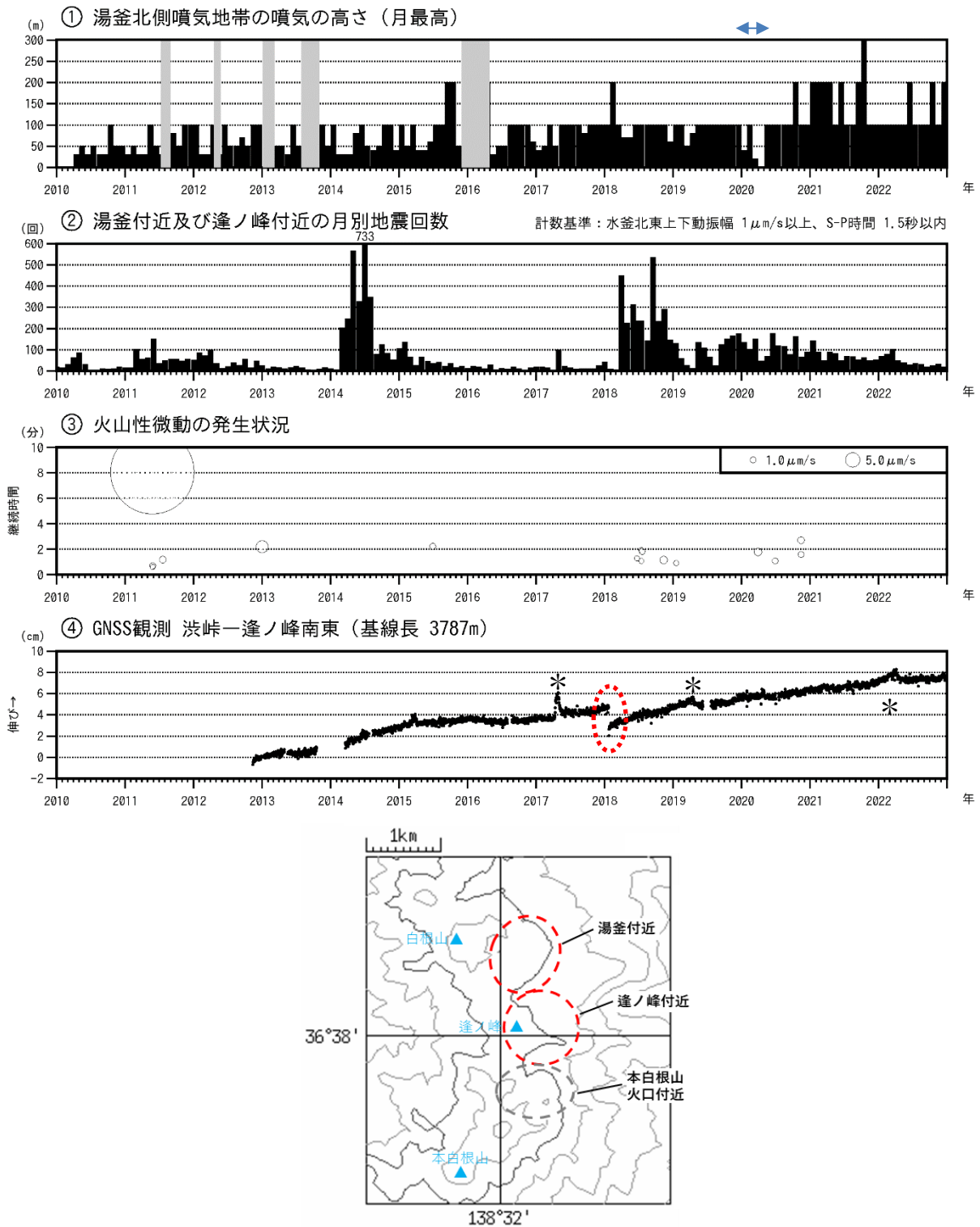
図3 草津白根山（白根山（湯釜付近））火山活動経過図（2010年1月1日～2022年12月31日）
