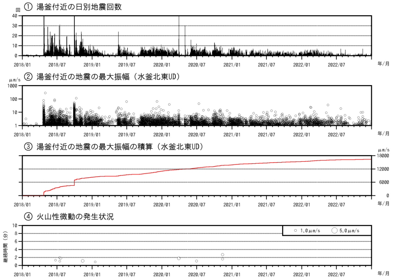
図1 草津白根山（白根山（湯釜付近）） 湯釜付近の地震活動及び火山性微動の発生状況 （2018年1月1日～2022年12月31日）
