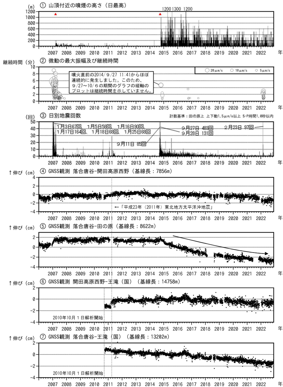
図1 御嶽山 長期間の火山活動経過図（2006年1月1日～2022年11月30日）
