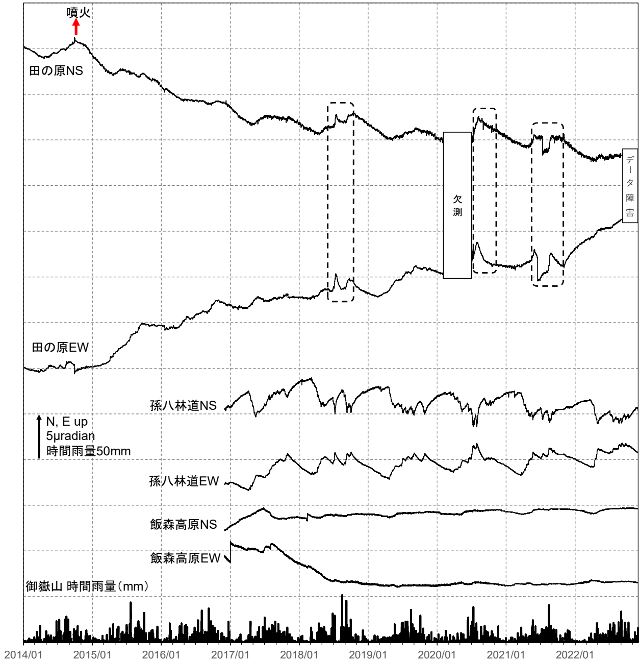
図4 御嶽山 傾斜変動（2014年1月1日～2022年11月30日）
