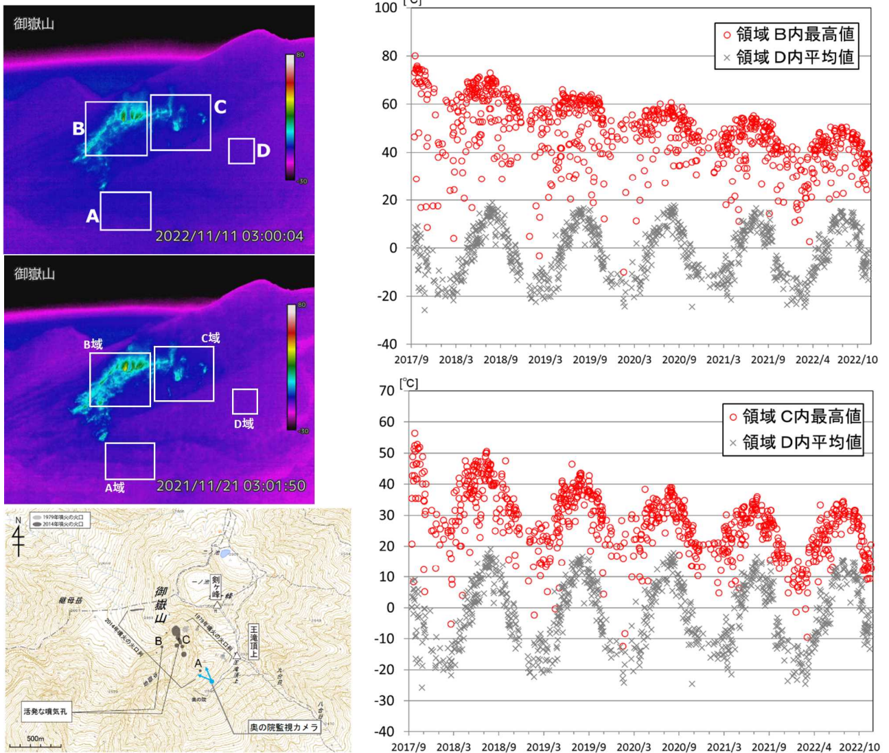
図6 御嶽山 奥の院赤外熱映像カメラによる剣ヶ峰南西側における最高温度の推移 (2017年9月13日～2022年11月30日)
