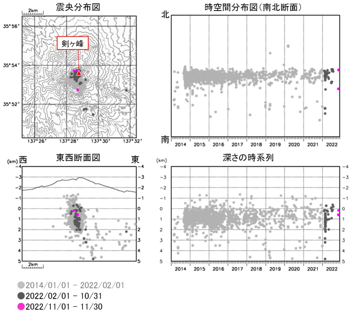
図2 御嶽山 震源分布図（2014年1月1日～2022年11月30日）
