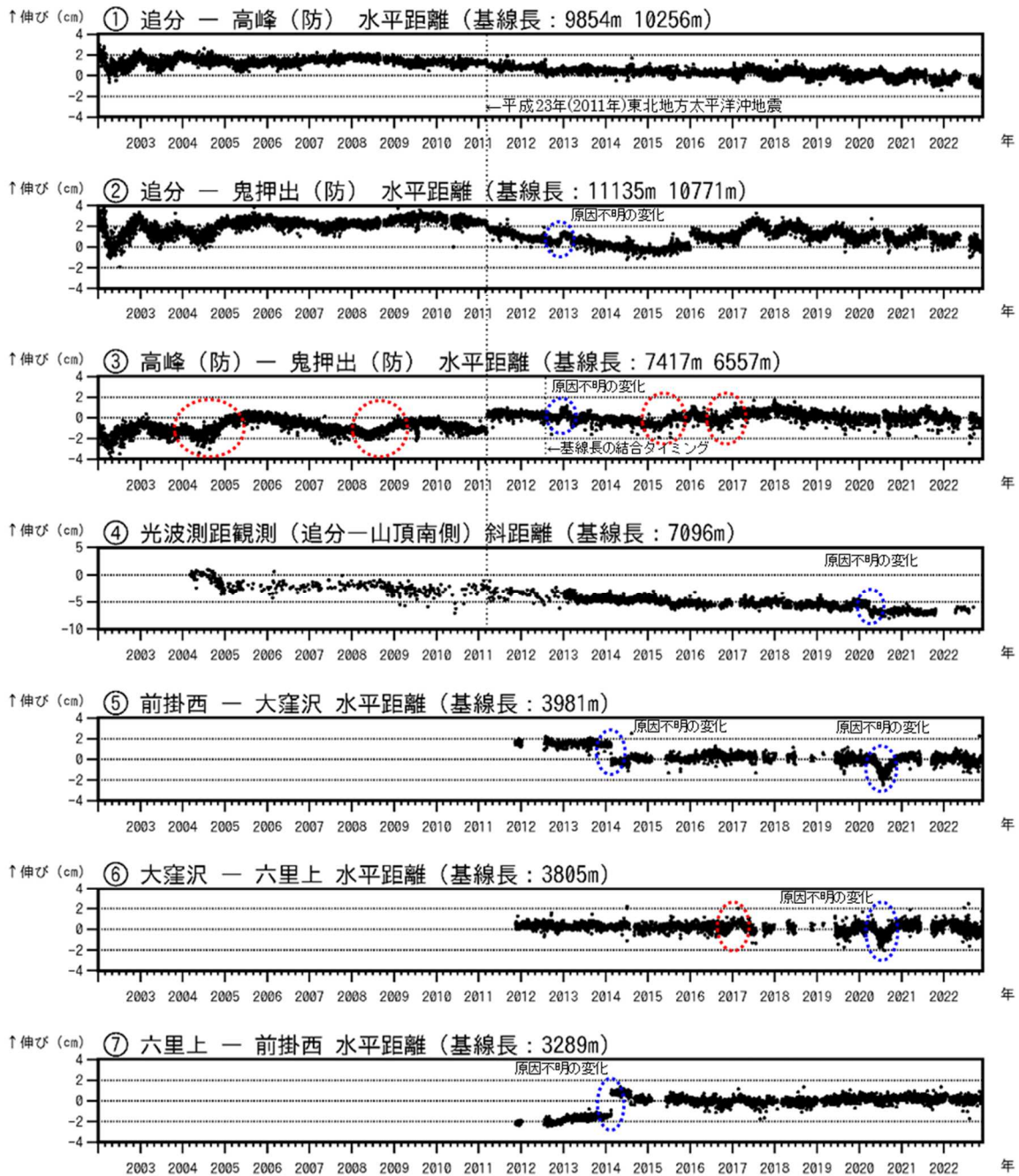
図6-1 浅間山 GNSS 連続観測及び光波測距観測の結果(2002年1月1日~2022年11月30日) GNSS 連続観測においては、2010年10月及び2016年1月に解析方法を変更しています。
