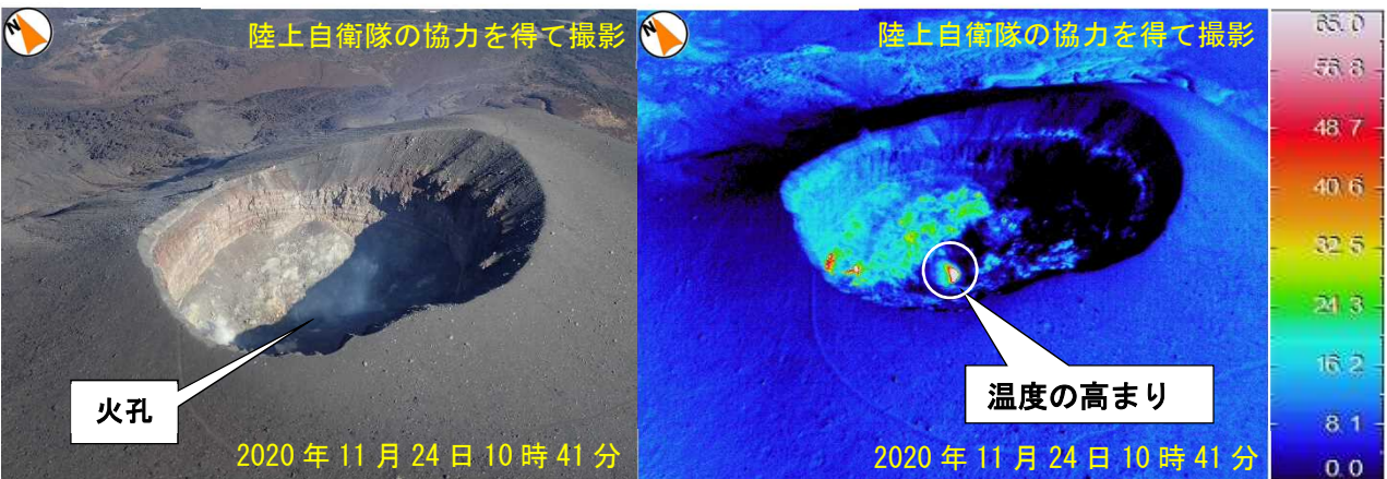
山頂火口の南西 高度約 3,000mから撮影（協力：陸上自衛隊） 撮影時の気象状況 天気：快晴、気温：約 9^{\circ}\text{C} 、湿度：約 9%
