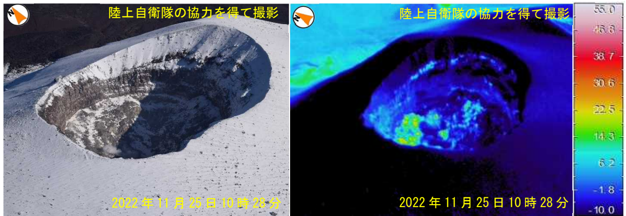
山頂火口の南西 高度約 3,100mから撮影（協力：陸上自衛隊） 撮影時の気象状況 天気：快晴、気温：約 -1.5^{\circ}\text{C} 、湿度：約 11%
