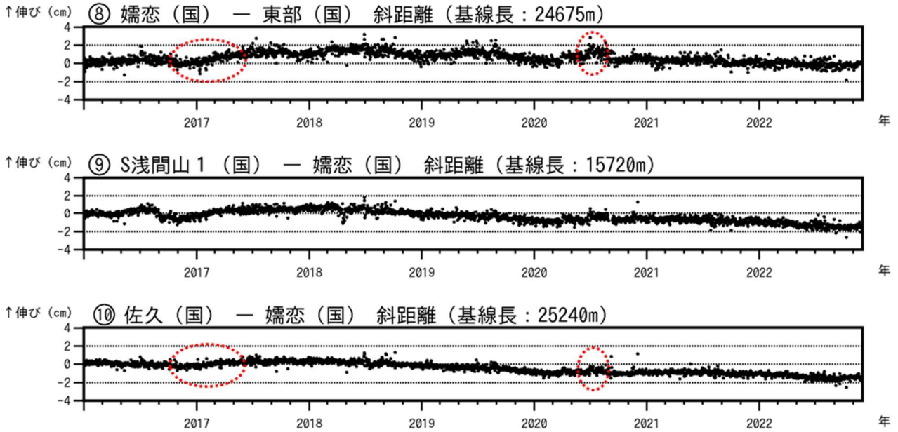
図6-2 浅間山 GNSS 連続観測結果(2016年1月1日~2022年11月30日)
