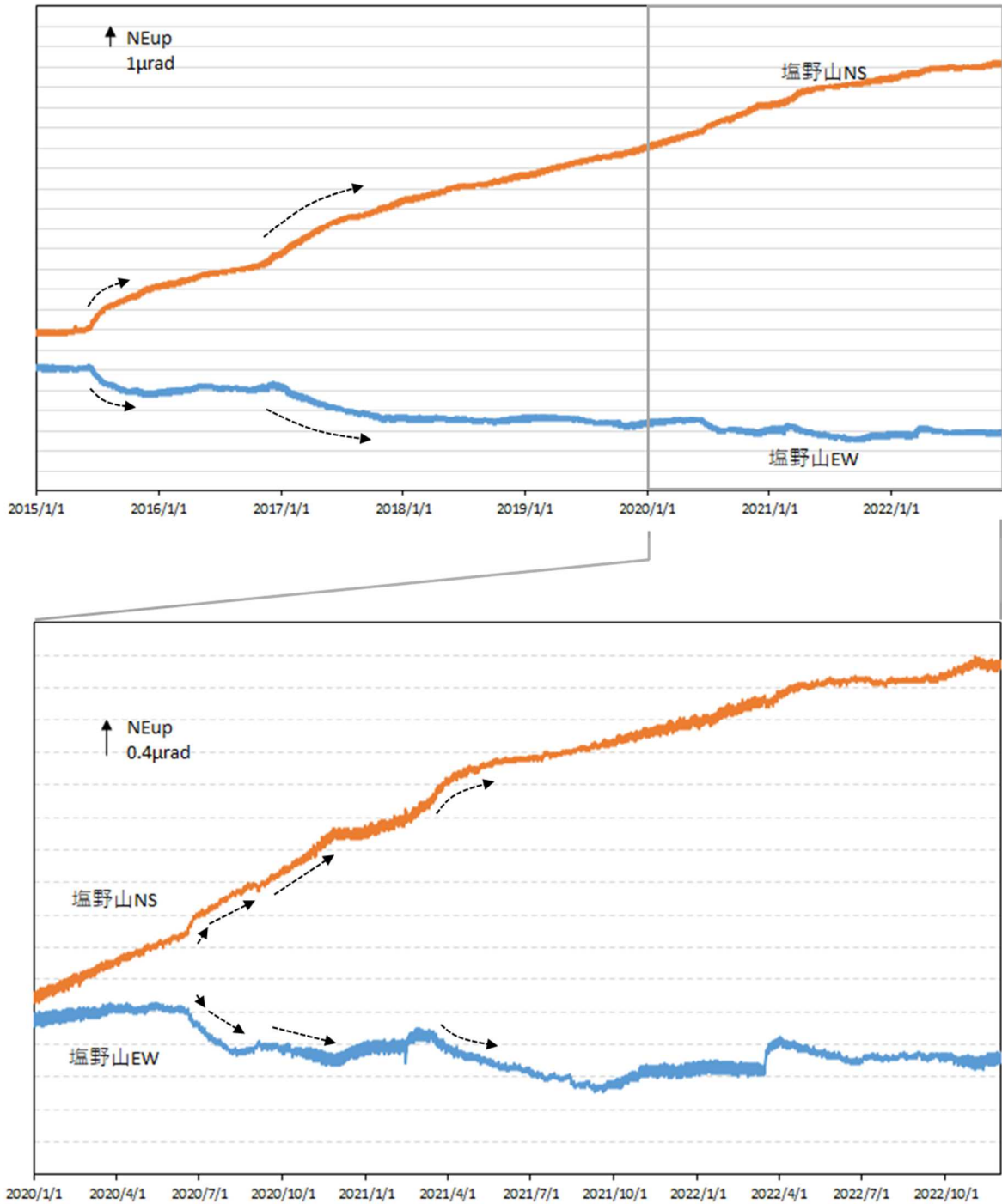
図8 浅間山 塩野山観測点における傾斜データ（2015年1月1日～2022年11月30日） データは時間平均値を使用しており、長期にわたるトレンドを補正しています。 下段は上段に比べて縦軸を拡大しています。
