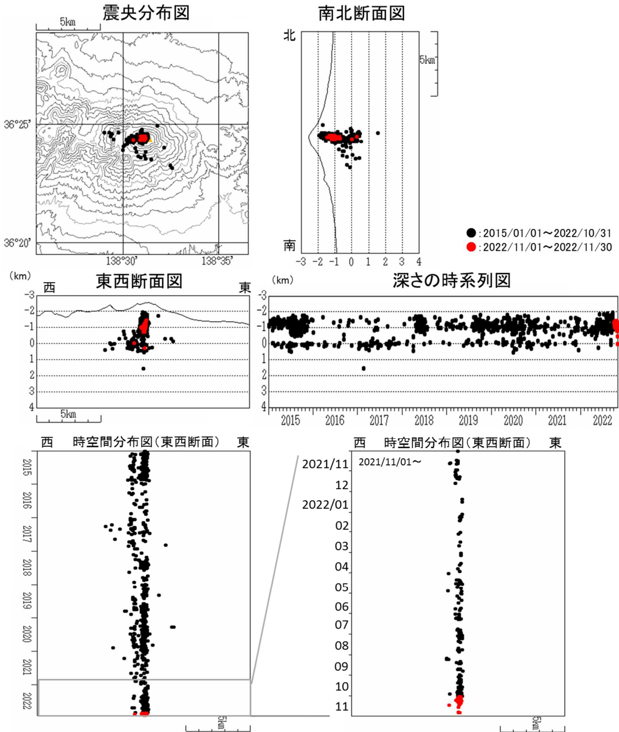
図5 浅間山 震源分布図（2015年1月1日～2022年11月30日）
