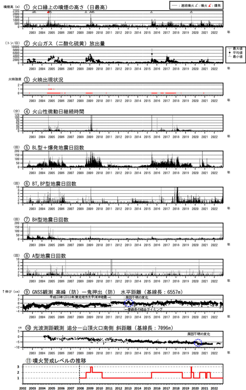
図4 浅間山 火山活動経過図（2002年1月1日～2022年11月30日）
