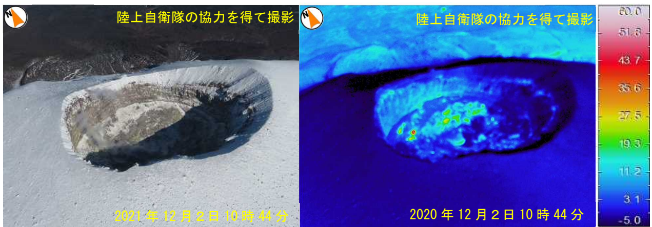
山頂火口の南西 高度約 3,000mから撮影（協力：陸上自衛隊） 撮影時の気象状況 天気：快晴、気温：約 -9^{\circ}\text{C} 、湿度：欠測
