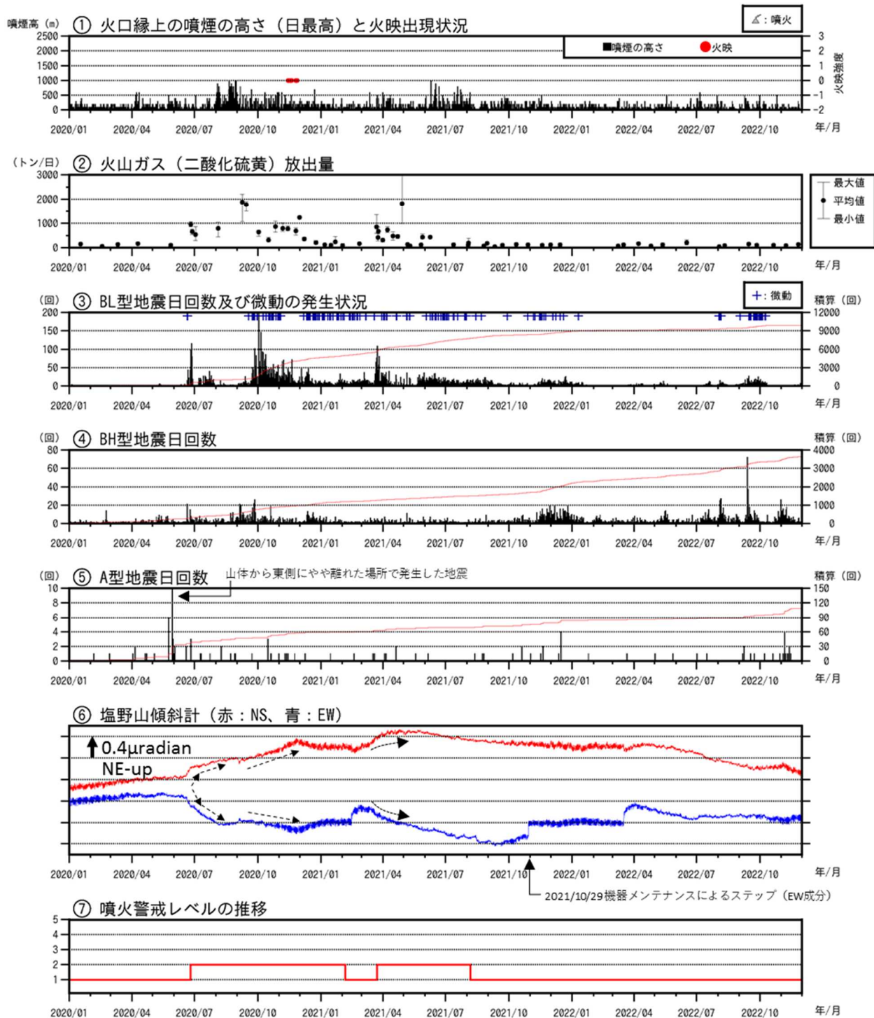
図3 浅間山 火山活動経過図（2020年1月1日～2022年11月30日）
