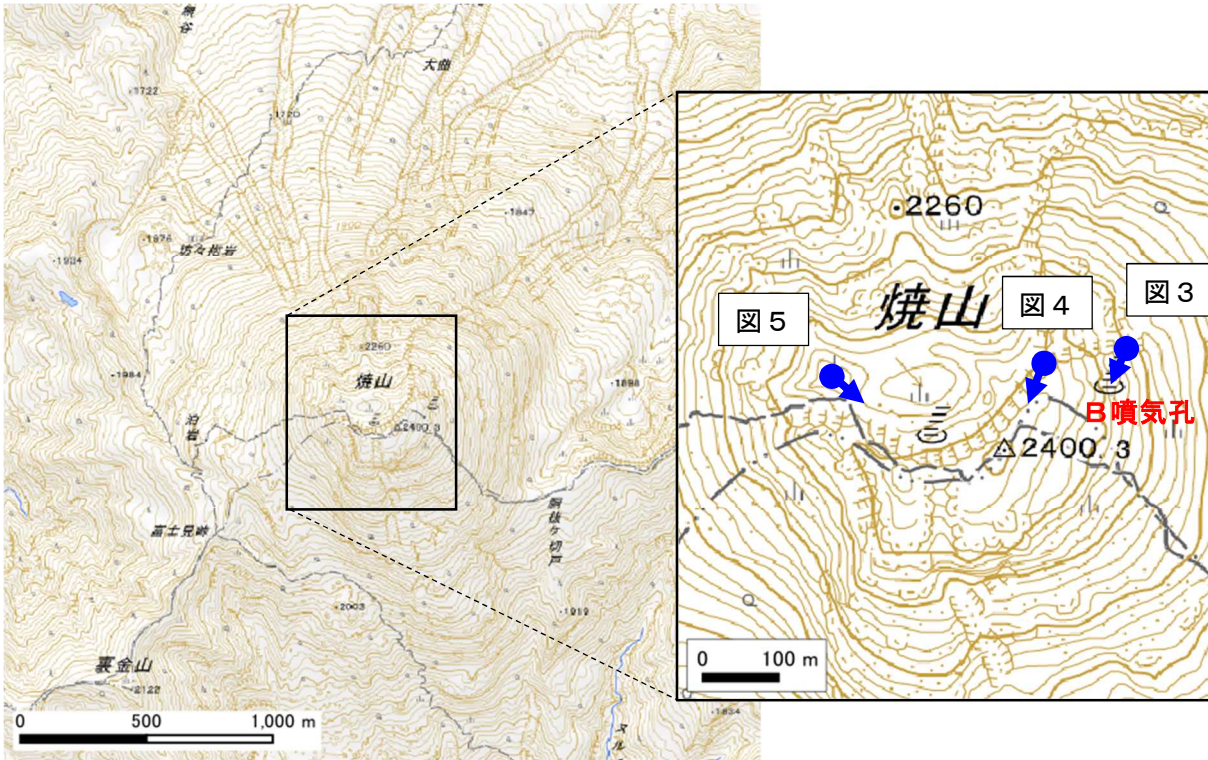
図2 新潟焼山 現地観測の観測点（図3、4、5の撮影位置と撮影方向） 矢印は、可視画像及び熱画像の撮影ポイント及び方向を示す。
