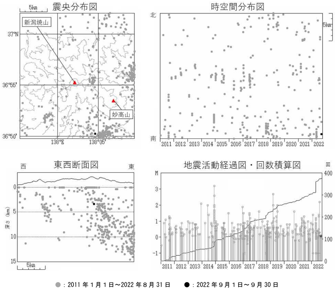
図8 新潟焼山 広域地震観測網による山体・周辺の地震活動(2011年1月1日～2022年9月30日)
