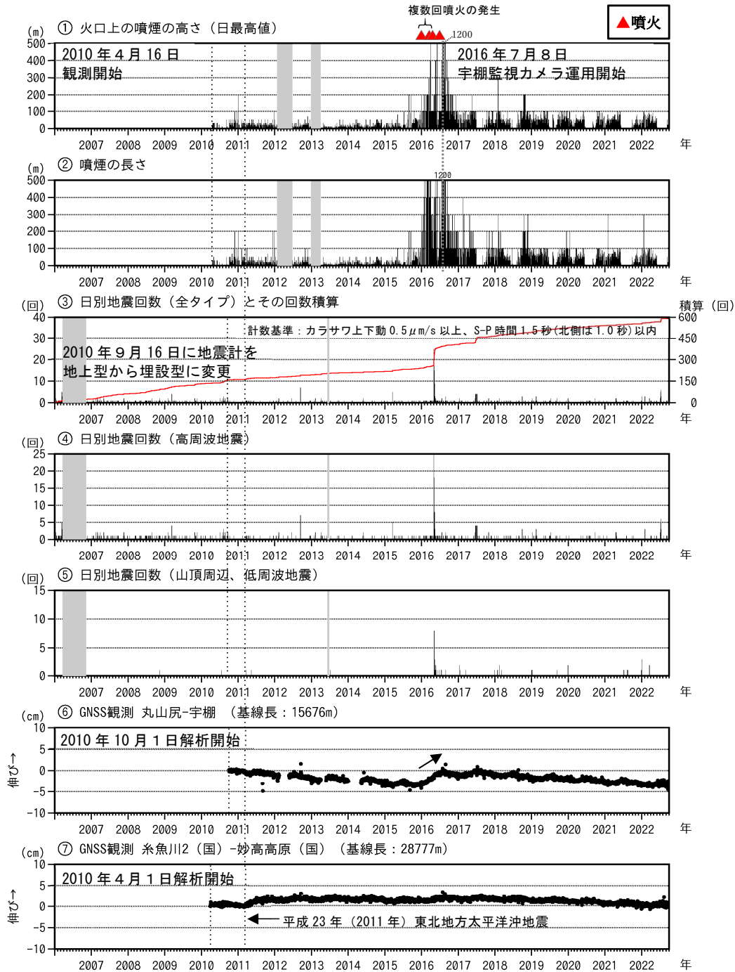
図6 新潟焼山 火山活動経過図（2006年1月1日～2022年9月30日）
