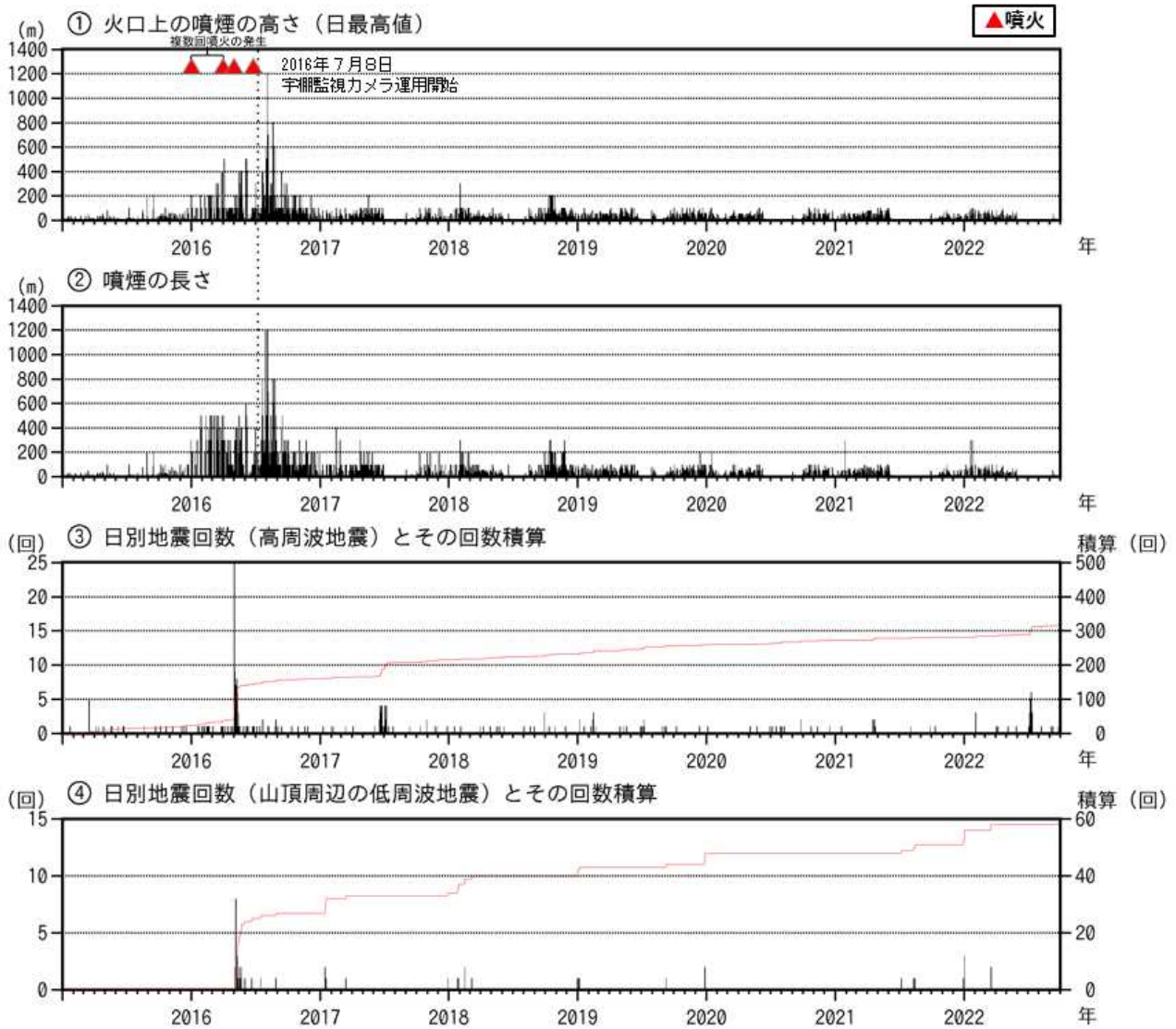
図7 新潟焼山 火山活動経過図（短期）（2015年1月1日～2022年9月30日）
