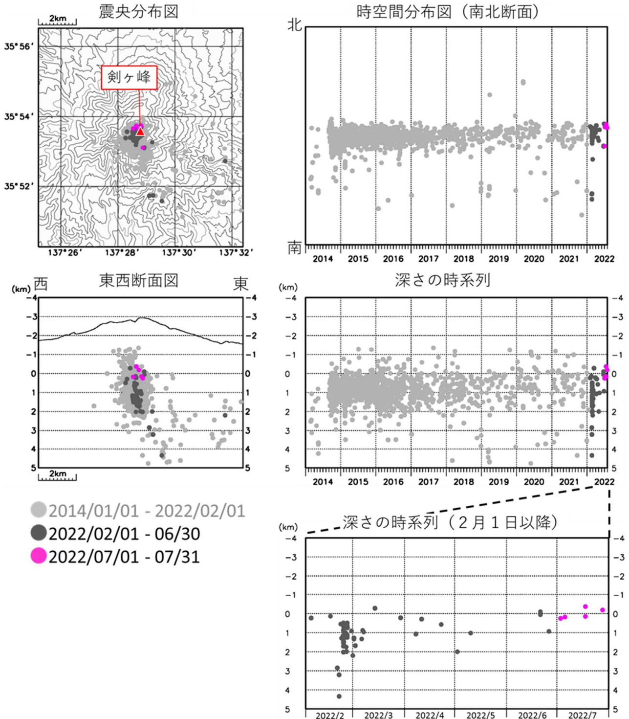
図2 御嶽山 震源分布図 (2014年1月1日~2022年7月31日) ※観測点の稼働状況により、求まる震源の数が減少したり、位置などの精度が低下したりする場合があります。
