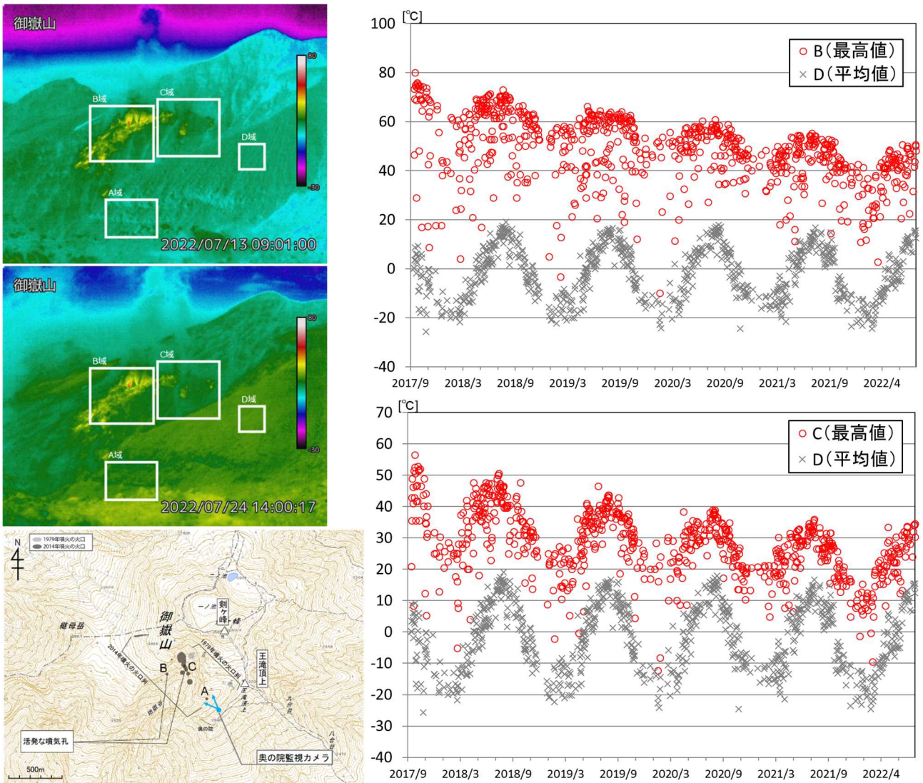
図6 御嶽山 奥の院赤外熱映像カメラによる剣ヶ峰南西側における最高温度の推移 (2017年9月13日～2022年7月31日)
