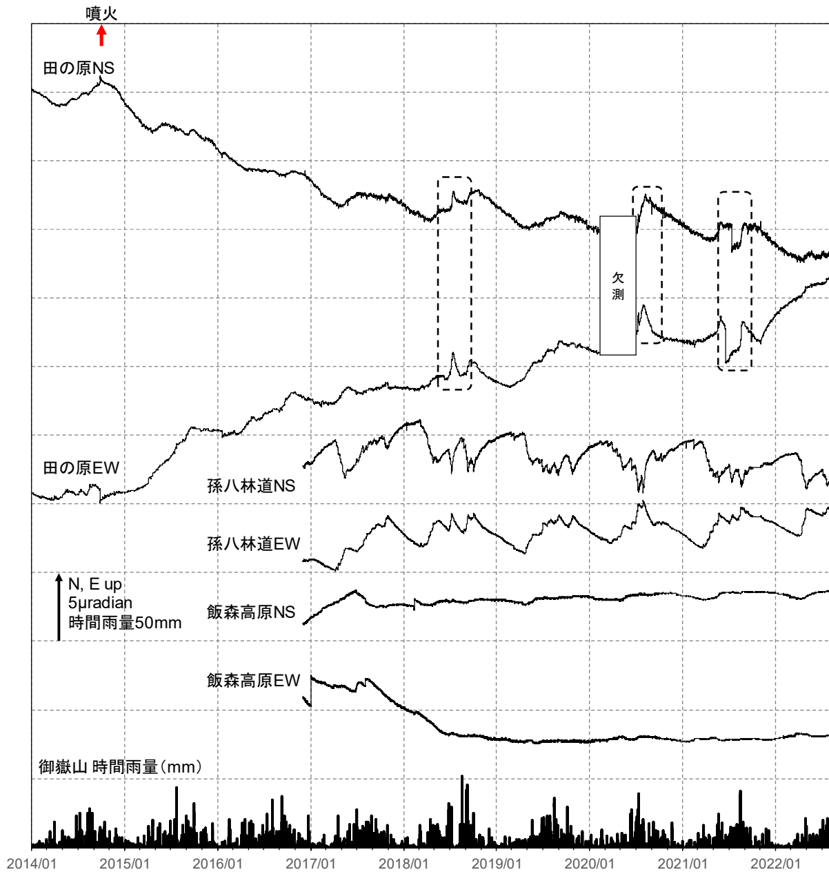
図4 御嶽山 傾斜変動（2014年1月1日～2022年7月31日）
