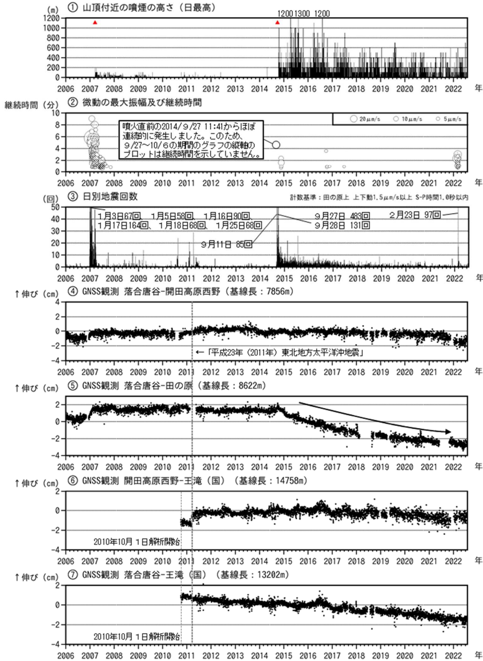
図1 御嶽山 長期間の火山活動経過図（2006年1月1日～2022年7月31日）
