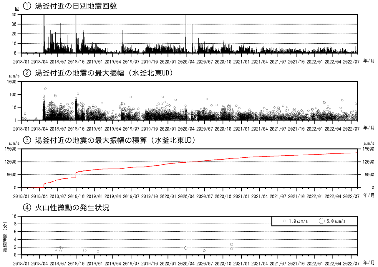
図1 草津白根山（白根山（湯釜付近）） 湯釜付近の地震活動及び火山性微動の発生状況 （2018年1月1日～2022年7月31日）
