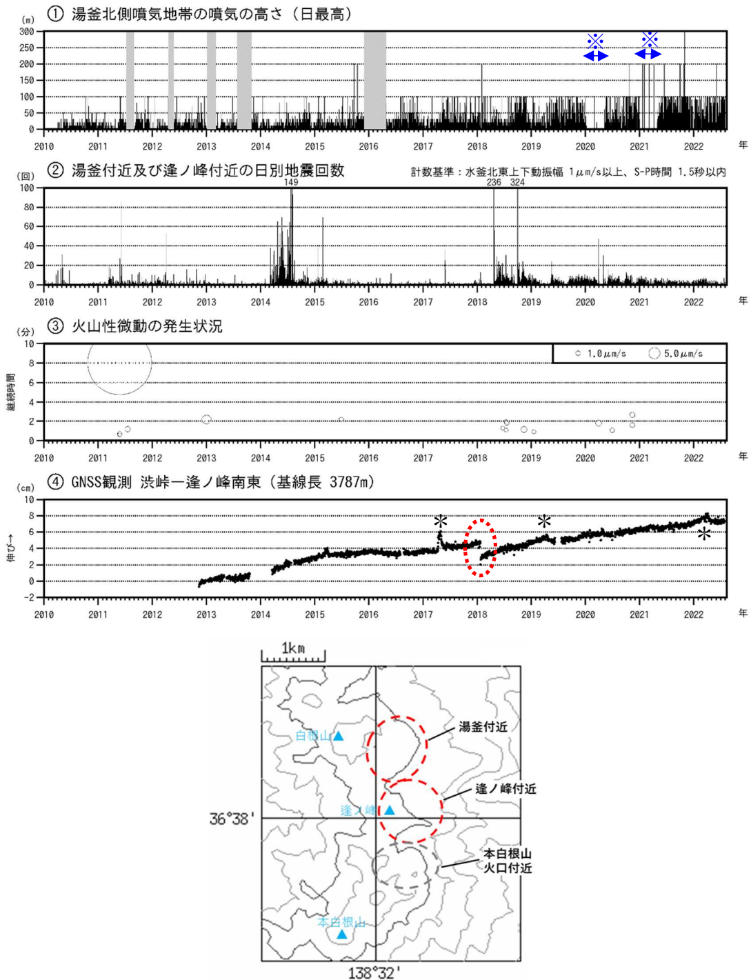
図3 草津白根山（白根山（湯釜付近））火山活動経過図（2010年1月1日～2022年7月31日） ①の灰色部分及び④の空白部分は欠測を示します。また、※の青矢印期間（2020年1月から4月にかけて、及び2021年1月から4月にかけて）は、一部の観測機器で障害が発生しているため、100m未満の噴気については観測できていない期間があります。 ④は図7の④の基線に対応しています。2016年1月以降のデータについては、解析方法を改良しています。*の変動は、渋峠または逢ノ峰南東 GNSS 連続観測点固有の変動に対応し、火山活動によるものではないと考えられます。 最下段の図は、図1①②③と図3②の地震の震源の概ねの位置を示しています。 ・草津白根山では、2014年や2018年に湯釜付近浅部への火山性流体の著しい供給の増加によると考えられる火山性地震の活発化と浅部の膨張などが観測されました。草津白根山の火山活動は、短期的には活動の消長があるものの、中長期的には活発な状態が継続していると考えられます。 ・GNSS 連続観測では、今期間、火山活動によるとみられる変動は認められません。 ・④の基線では、2018年1月の本白根山噴火に伴う変化（赤色破線）が認められた後、2020年1月にかけて、噴火後の本白根山の収縮によるものと考えられる変動がみられました。
