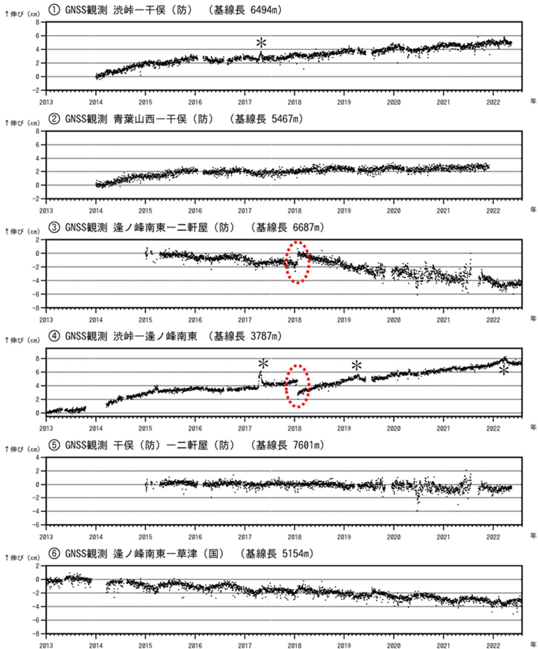
図6 草津白根山 GNSS連続観測の結果（2013年1月1日～2022年7月31日）
