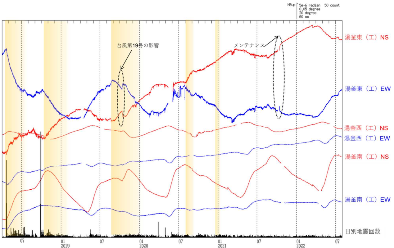
図5 草津白根山（白根山（湯釜付近）） 傾斜変動（2018年4月1日～2022年7月31日）
