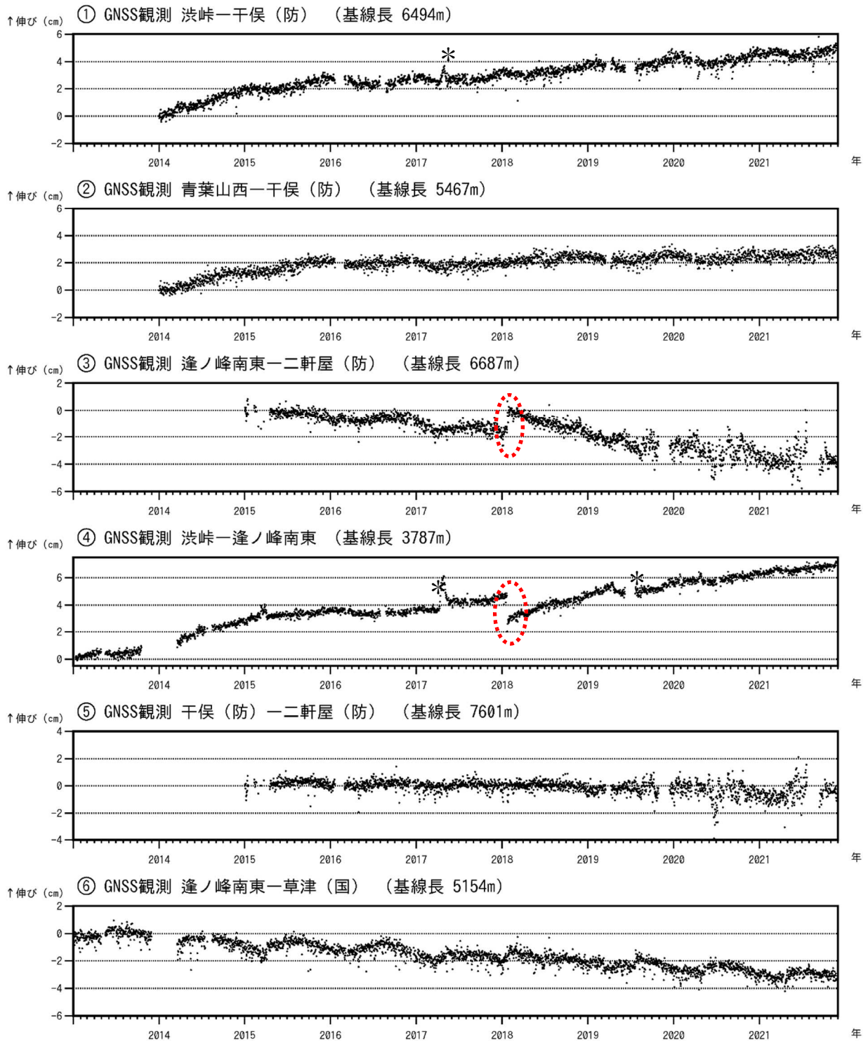
図6 草津白根山 GNSS連続観測の結果 (2013年1月1日~2021年11月30日)
