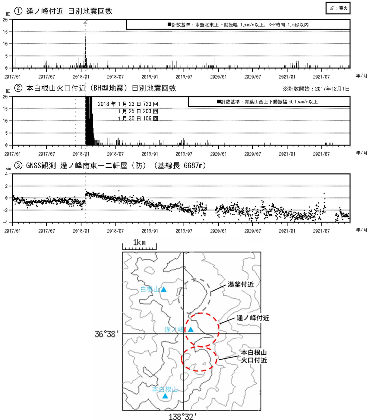
図12 草津白根山（本白根山） 火山活動経過図（2017年1月1日～2021年11月30日）
