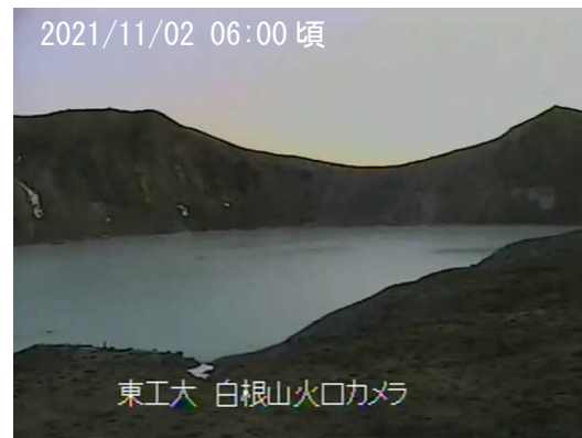
図2 草津白根山（白根山（湯釜付近）） 湯釜付近の状況
