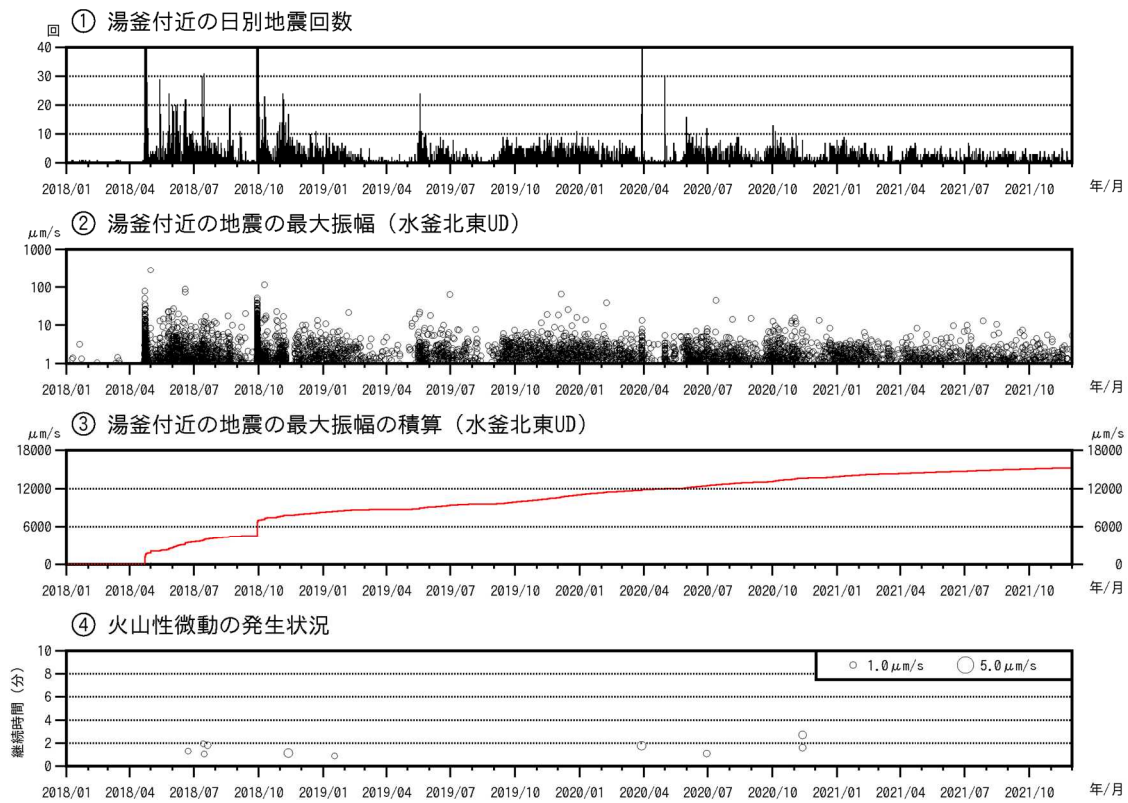
図1 草津白根山（白根山（湯釜付近）） 湯釜付近の地震活動及び火山性微動の発生状況 （2018年1月1日～2021年11月30日）
