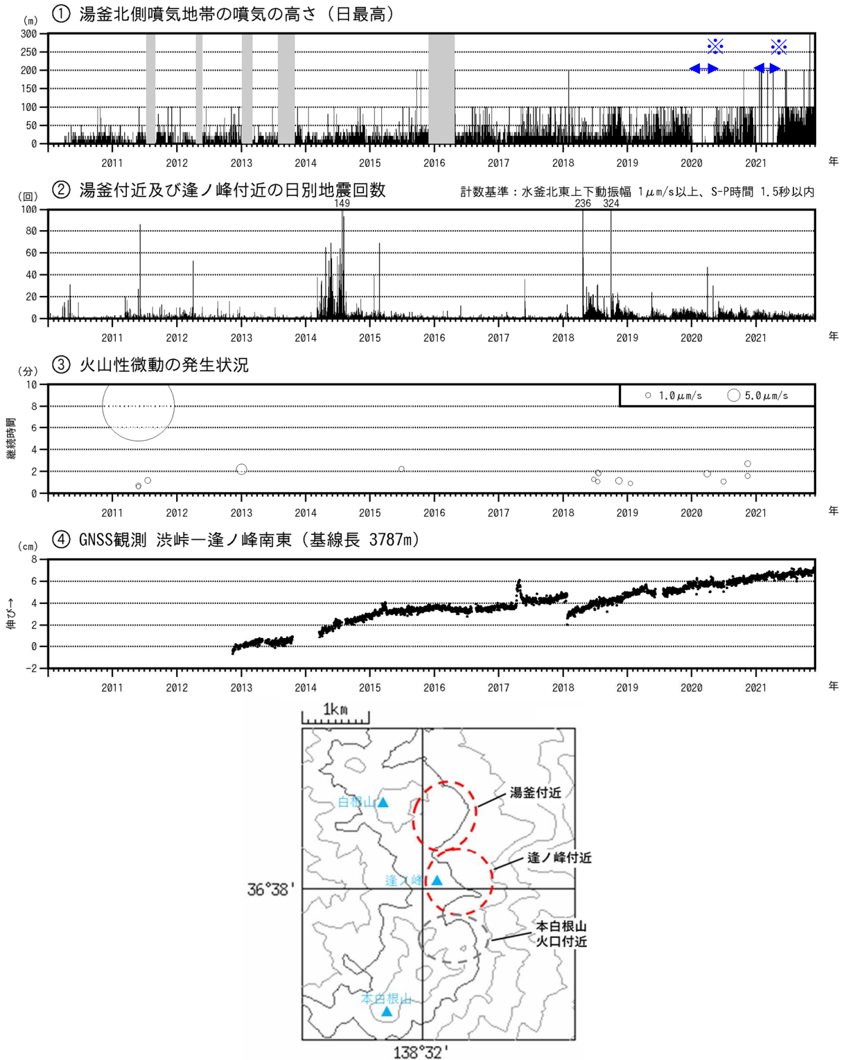
図3 草津白根山（白根山（湯釜付近）） 火山活動経過図（2010年1月1日～2021年11月30日）
