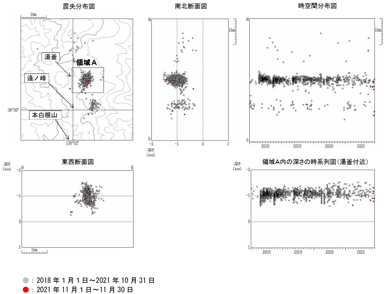
図4 草津白根山 震源分布図（2018年1月1日～2021年11月30日）
