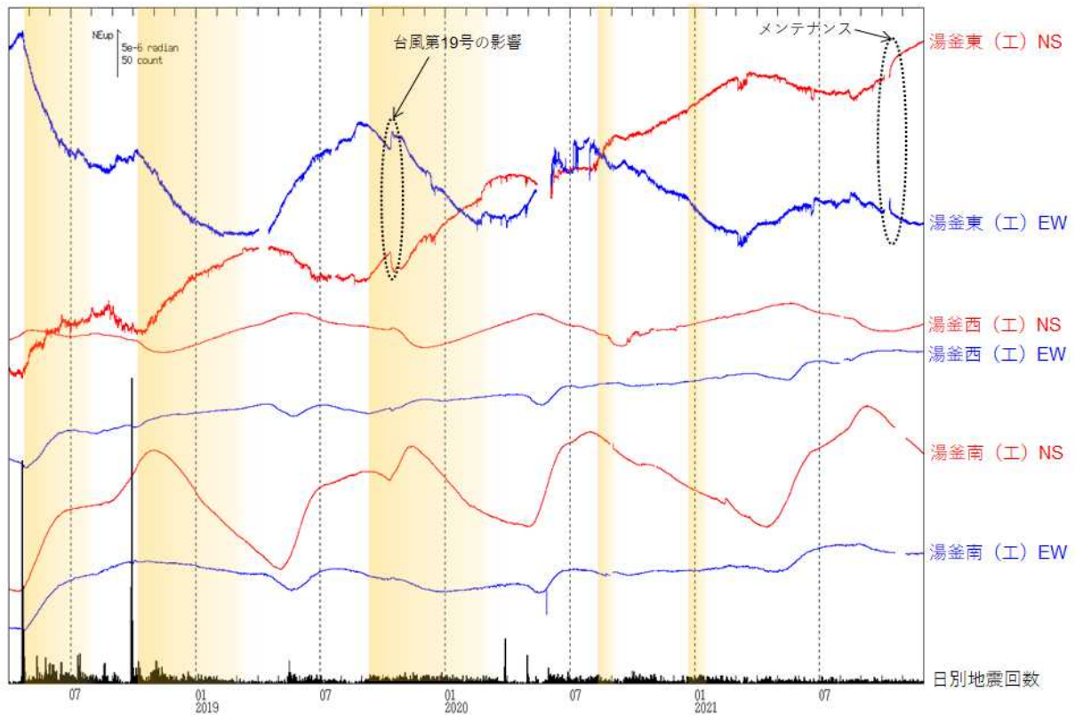
図5 草津白根山（白根山（湯釜付近）） 傾斜変動（2018年4月1日～2021年11月30日）
