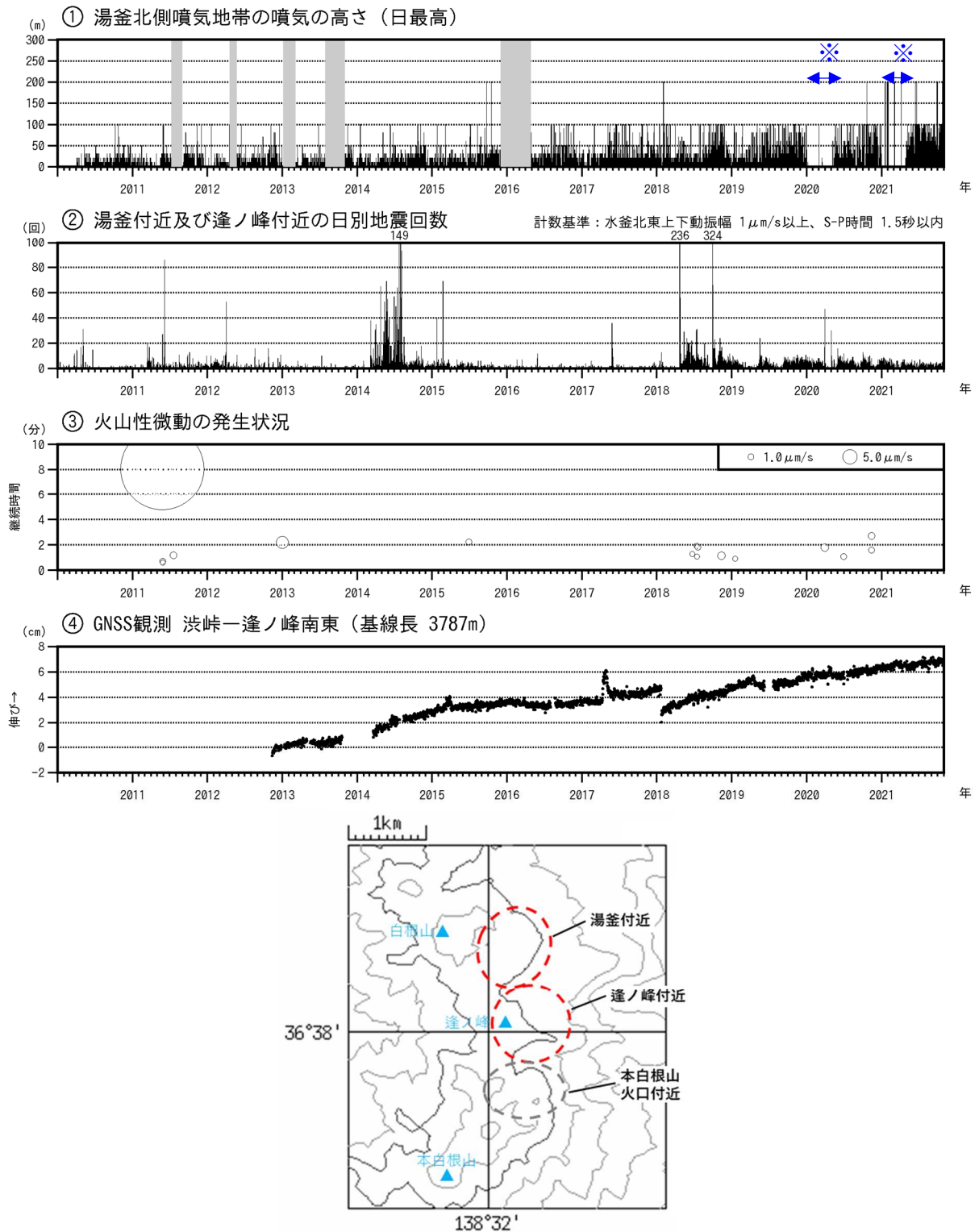
図3 草津白根山（白根山（湯釜付近））火山活動経過図（2010年1月1日～2021年10月31日） ①の灰色部分及び④の空白部分は欠測を示します。また、※の青矢印期間は（2020年1月から4月にかけて、及び2021年1月から4月にかけて）は、一部の観測機器で障害が発生しているため、100m未満の噴気については観測できていない期間があります。 ④は図7の④の基線に対応しています。2013年1月に解析方法を変更しています。 最下段の図は、図1①②③と図3②の地震の震源の概ねの位置を示しています。 ・草津白根山では、2014年や2018年に湯釜付近浅部への火山性流体の著しい供給の増加によると考えられる火山性地震の活発化と浅部の膨張などが観測されました。草津白根山の火山活動は、短期的には活動の消長があるものの、中長期的には活発な状態が継続していると考えられます。 ・GNSS連続観測では、2018年1月の本白根山噴火に伴う変化が認められた後、2020年1月にかけて、噴火後の本白根山の収縮によるものと考えられる変動が見られました。 ・GNSS連続観測では、今期間、火山活動によるとみられる変動は認められません。
