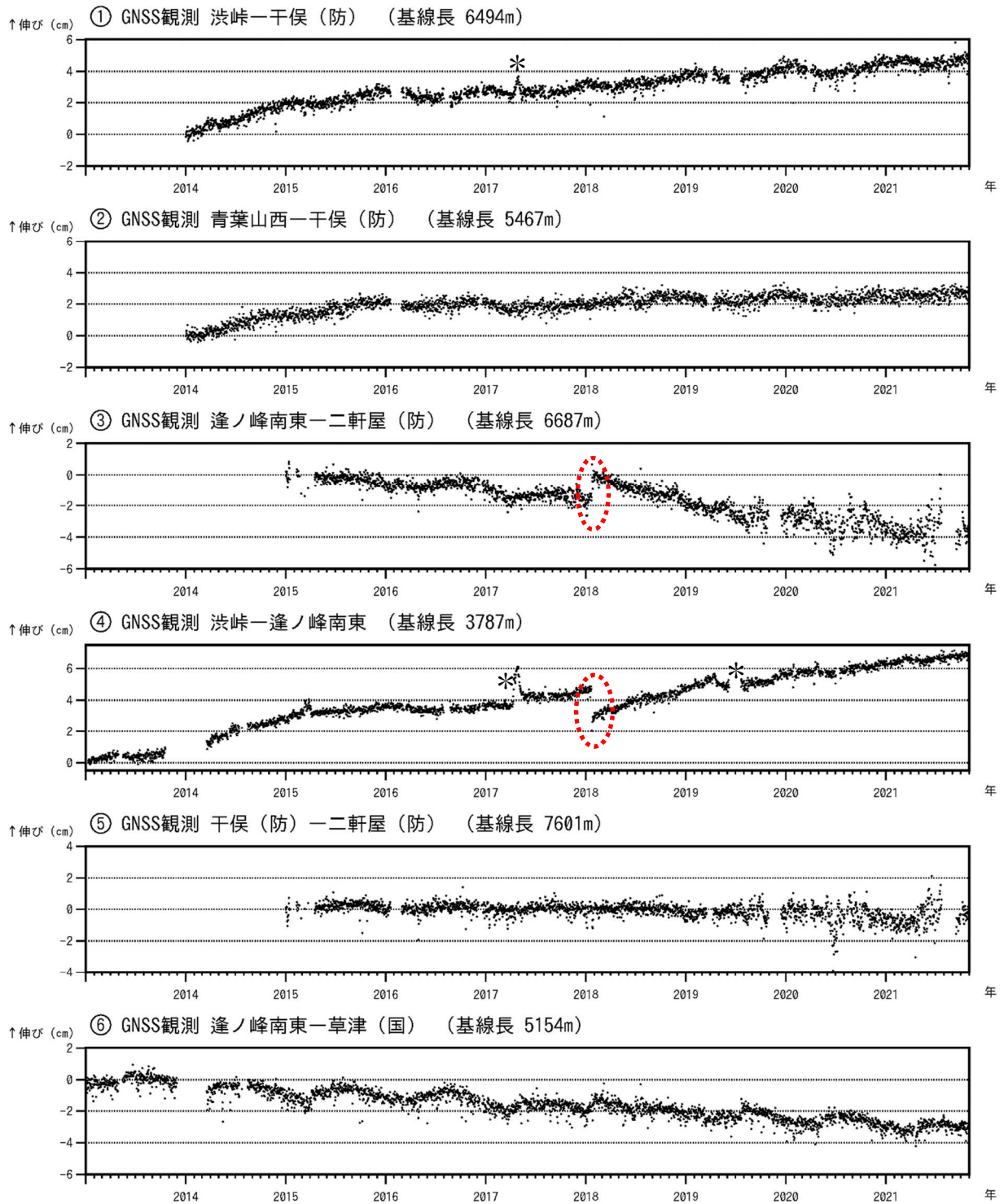
図6 草津白根山 GNSS連続観測の結果（2013年1月1日～2021年10月31日）
