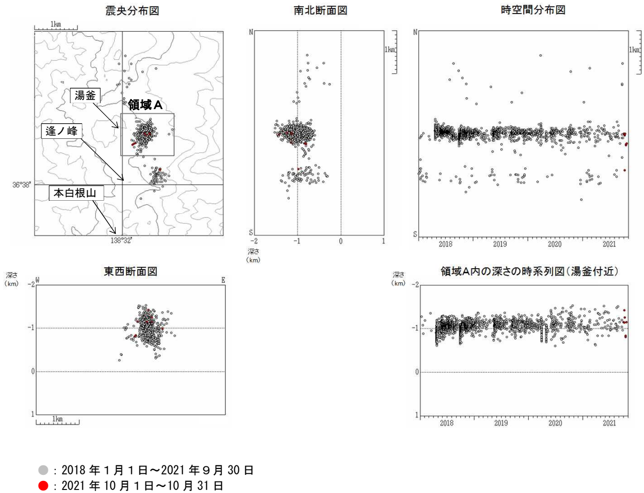
図4 草津白根山 震源分布図（2018年1月1日～2021年10月31日）
