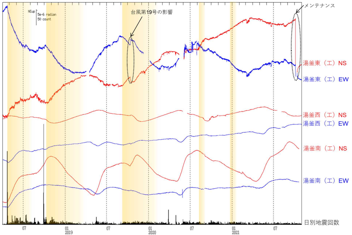
図5 草津白根山（白根山（湯釜付近）） 傾斜変動（2018年4月1日～2021年10月31日） （工）：東京工業大学
