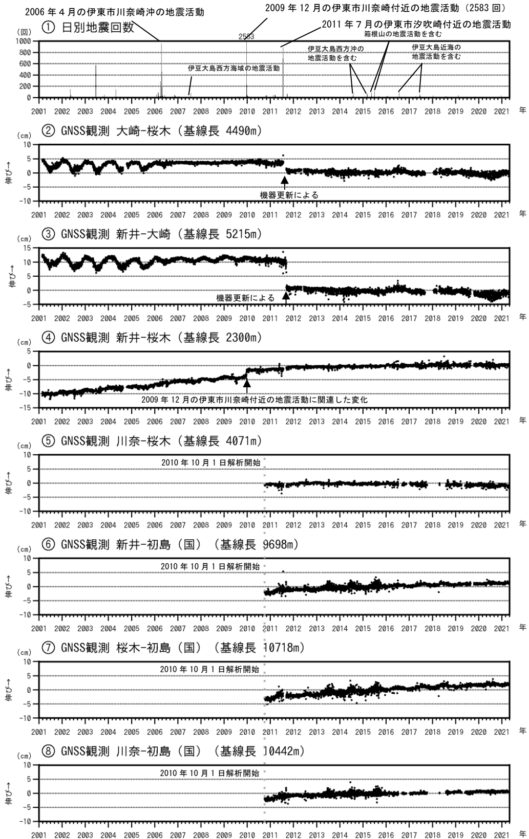
図3 伊豆東部火山群 火山活動経過図（2001年1月1日～2021年4月30日）
