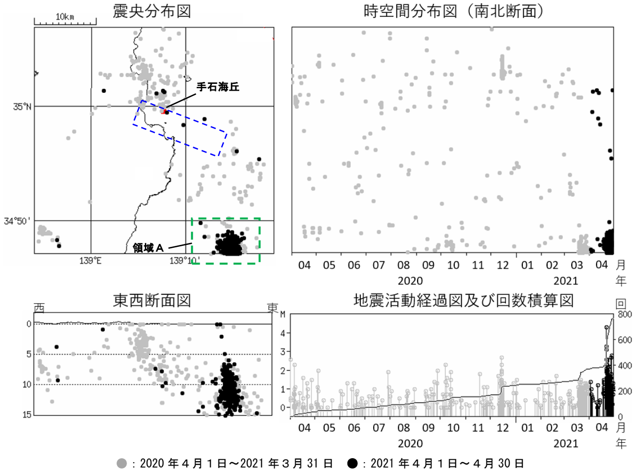
図2 伊豆東部火山群 広域地震観測網による震源分布図（2020年4月1日～2021年4月30日） □の領域は群発地震活動の発生する可能性がある範囲（火口が発生する可能性のある範囲）を示しています。 https://www.data.jma.go.jp/svd/vois/data/tokyo/STOCK/level/PDF/level_316.pdf 広域地震観測網により震源決定したもので、深さは全て海面以下として決定しています。 M（マグニチュード）は地震の規模を表し、M0.0以上を表示しています。 図中の震源要素は一部暫定値が含まれており、後日変更することがあります。 この図では、関係機関の地震波形を一元的に処理し、地震観測点の標高を考慮する等した新手法で得られた震源を用いています（ただし、2020年8月以前の地震については火山活動評価のための参考震源です）。 2021年5月13日現在、次の期間の地震について、暫定的に震源精査の基準を変更しているため、その前後の期間と比較して微小な地震での震源決定数の変化（増減）が見られます。 (1)2020年4月18日から10月23日まで、(2)2021年1月9日から3月7日まで、(3)2021年4月19日以降
