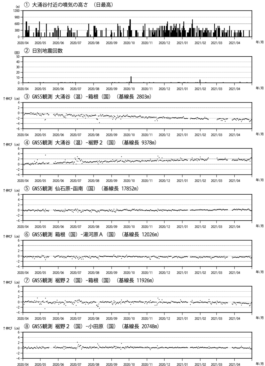
図7 箱根山 火山活動経過図（2020年4月1日～2021年4月30日）
