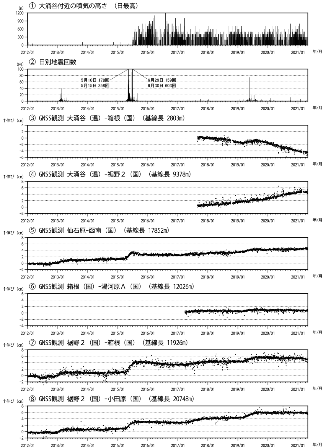
図6 箱根山 火山活動経過図（2012年1月1日～2021年4月30日）
