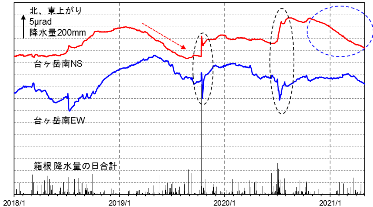
図9 箱根山 台ヶ岳南観測点における傾斜データ（2018年1月1日～2021年4月30日）
