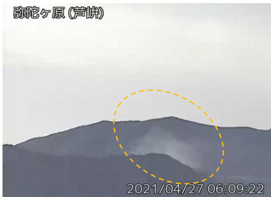
図1 弥陀ヶ原 地獄谷からの噴気の状況（橙丸）（4月27日、芦峠監視カメラによる）
