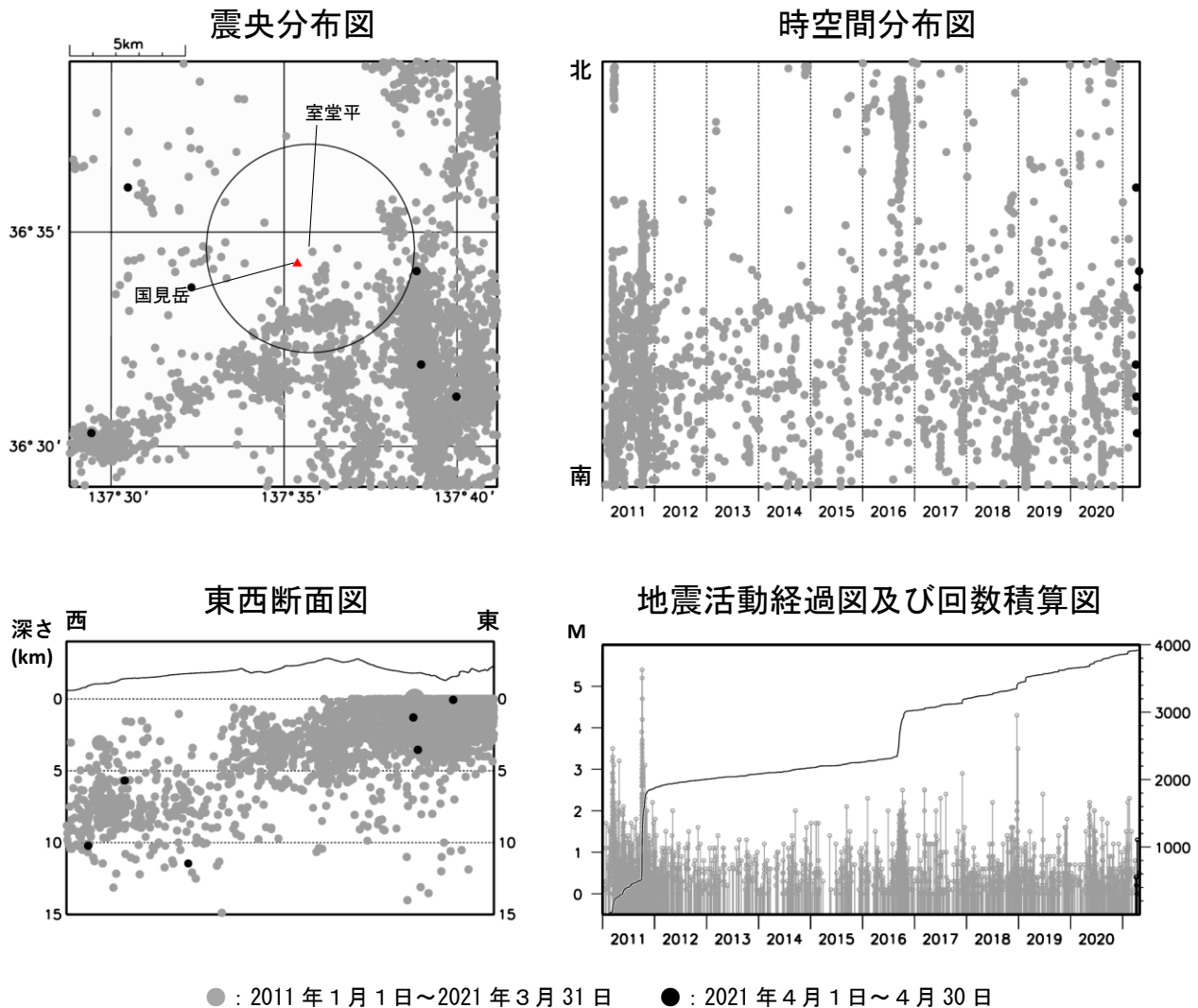
図2 弥陀ヶ原 広域地震観測網による山体・周辺の地震活動（2011年1月1日～2021年4月30日） 震央分布図中の円は弥陀ヶ原の計数対象地震（室堂平でS-P時間1秒以内）のおよその範囲を示しています。 広域地震観測網により震源決定したもので、深さは全て海面以下として決定しています。 図中の震源要素は一部暫定値が含まれており、後日変更することがあります。 この図では、関係機関の地震波形を一元的に処理し、地震観測点の標高を考慮する等した新手法で得られた震源を用いています（ただし、2020年8月以前の地震については火山活動評価のための参考震源です）。 2021年5月13日現在、次の期間の地震について、暫定的に震源精査の基準を変更しているため、その前後の期間と比較して微小な地震での震源決定数の変化（増減）が見られます。 (1) 2020年4月18日から10月23日まで、(2) 2021年1月9日から3月7日まで、(3) 2021年4月19日以降
