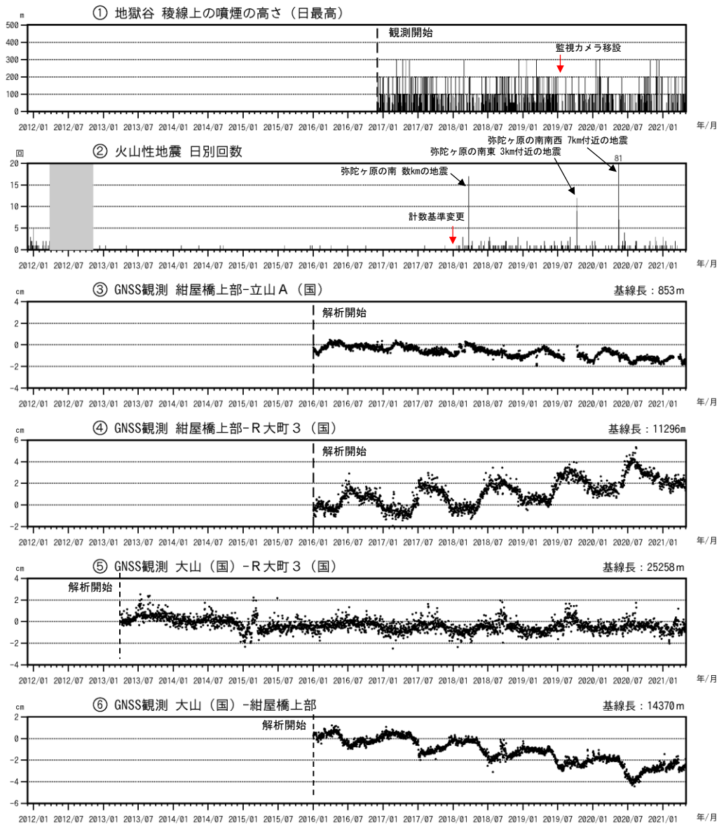
図3 弥陀ヶ原 火山活動経過図（2011年12月1日～2021年4月30日）
