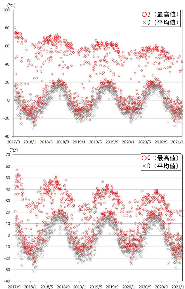
図2 御嶽山 奥の院赤外熱映像カメラによる剣ヶ峰南西側における最高温度の推移
