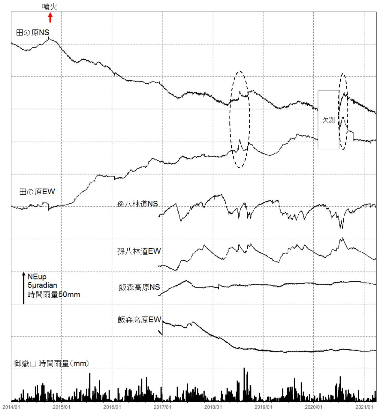
図7 御嶽山 傾斜変動（2014年1月1日～2021年3月31日）
