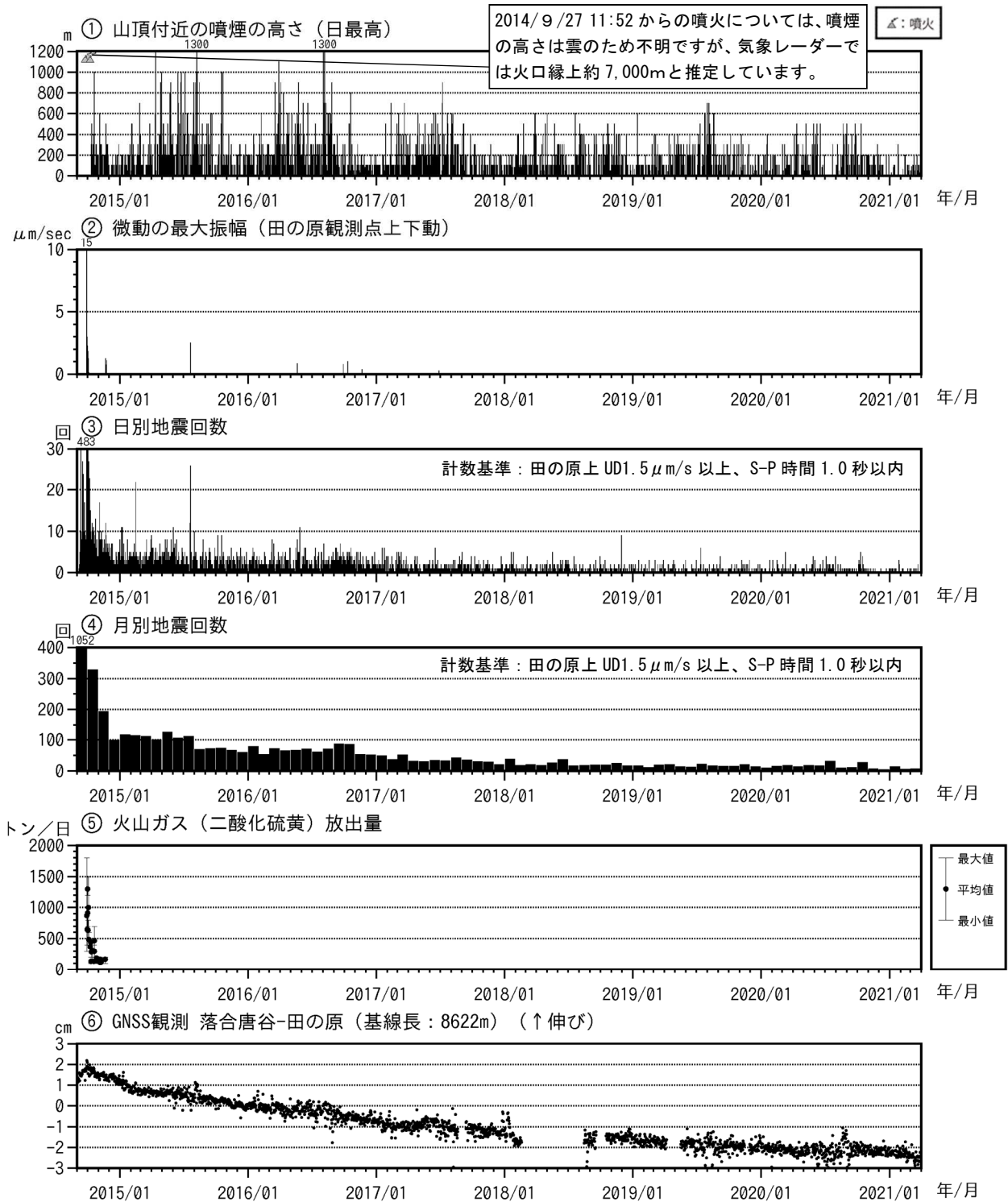
図4 御嶽山 最近の火山活動経過図（2014年9月1日～2021年3月31日）
