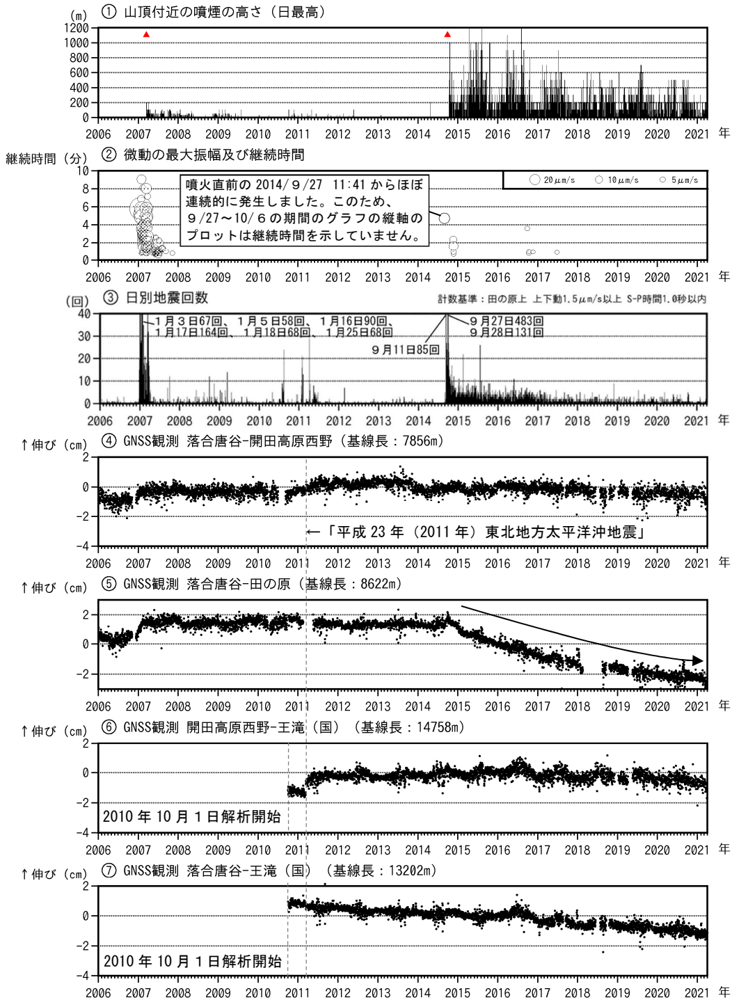
図5 御嶽山 長期間の火山活動経過図（2006年1月1日～2021年3月31日）
