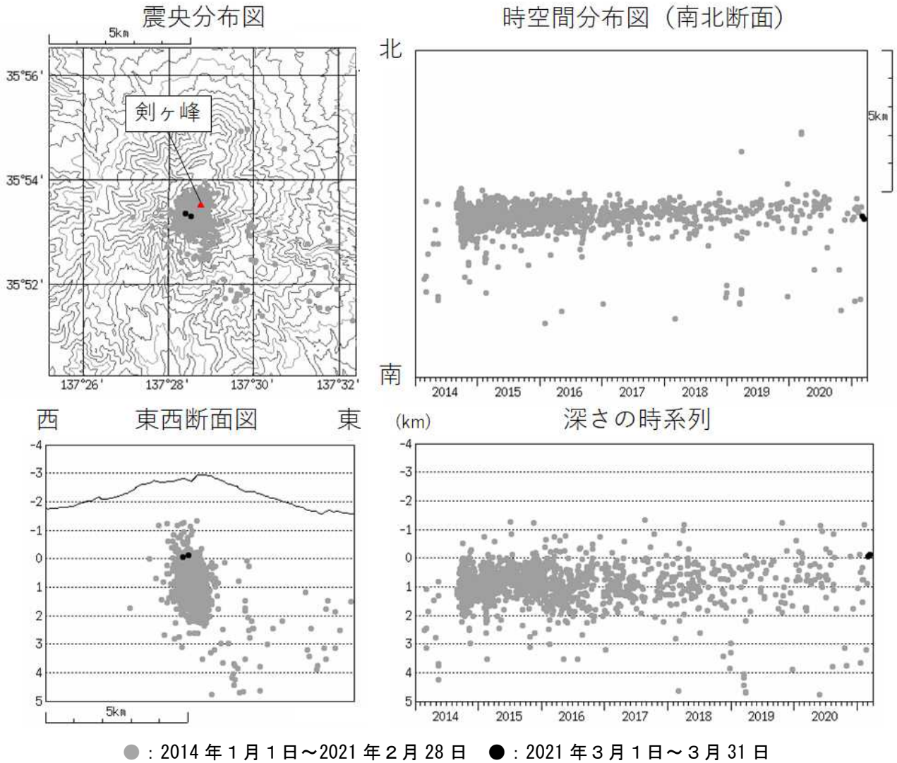
図3 御嶽山 震源分布図（2014年1月1日～2021年3月31日）
