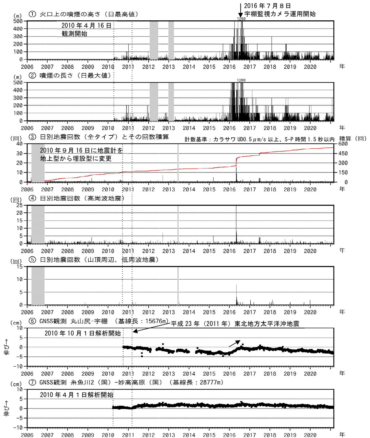
図2 新潟焼山 火山活動経過図（2006年1月1日～2021年2月28日）
