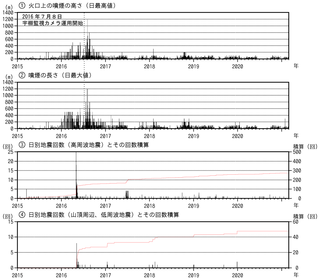
図3 新潟焼山 火山活動経過図（短期）（2015年1月1日～2021年2月28日）
