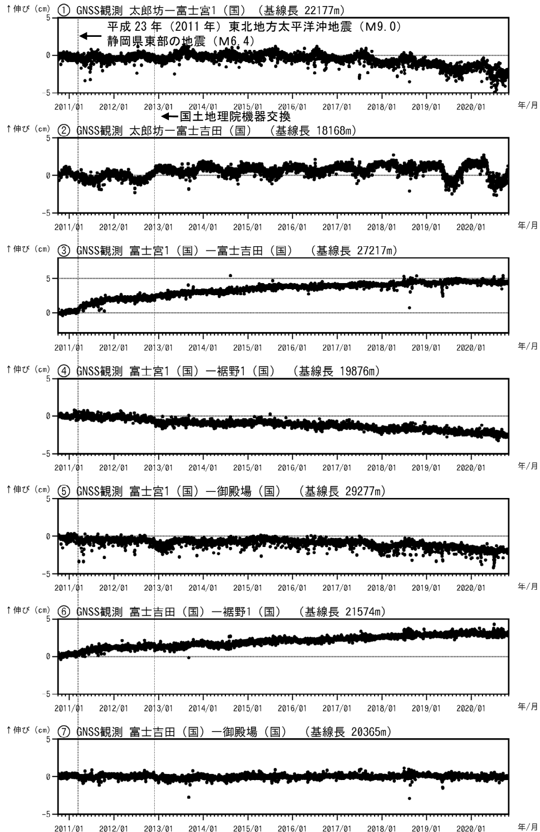
図4 富士山 GNSS連続観測による基線長変化（2010年10月1日～2020年10月31日）
