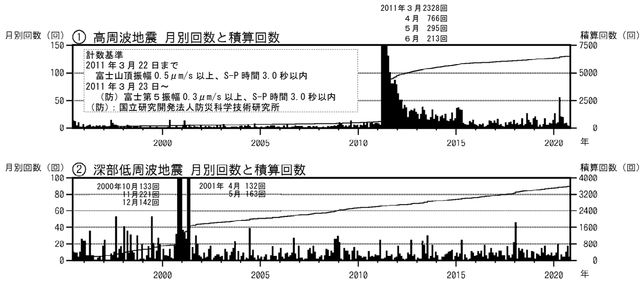
図2 富士山 月別地震回数（1995年6月1日～2020年10月31日）
