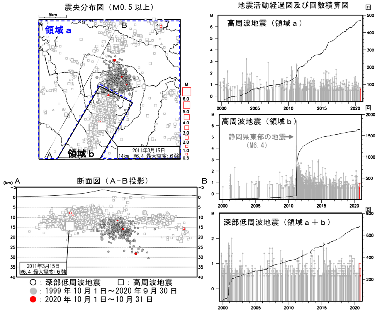
図3 富士山 広域地震観測網による山体及び周辺の地震活動(1999年10月1日～2020年10月31日) 広域地震観測網により震源決定したもので、深さは全て海面以下として決定しています。 M（マグニチュード）は地震の規模を表します。図中の震源要素は一部暫定値が含まれており、後日変更することがあります。 2020年11月10日現在、2020年4月18日から10月23日までの地震について、暫定的に震源精査の基準を変更しているため、その前後の期間と比較して微小な地震での震源決定数の変化（増減）が見られます。 2020年9月以降の震源は、地震観測点の標高を考慮する等した新手法で求められています。
