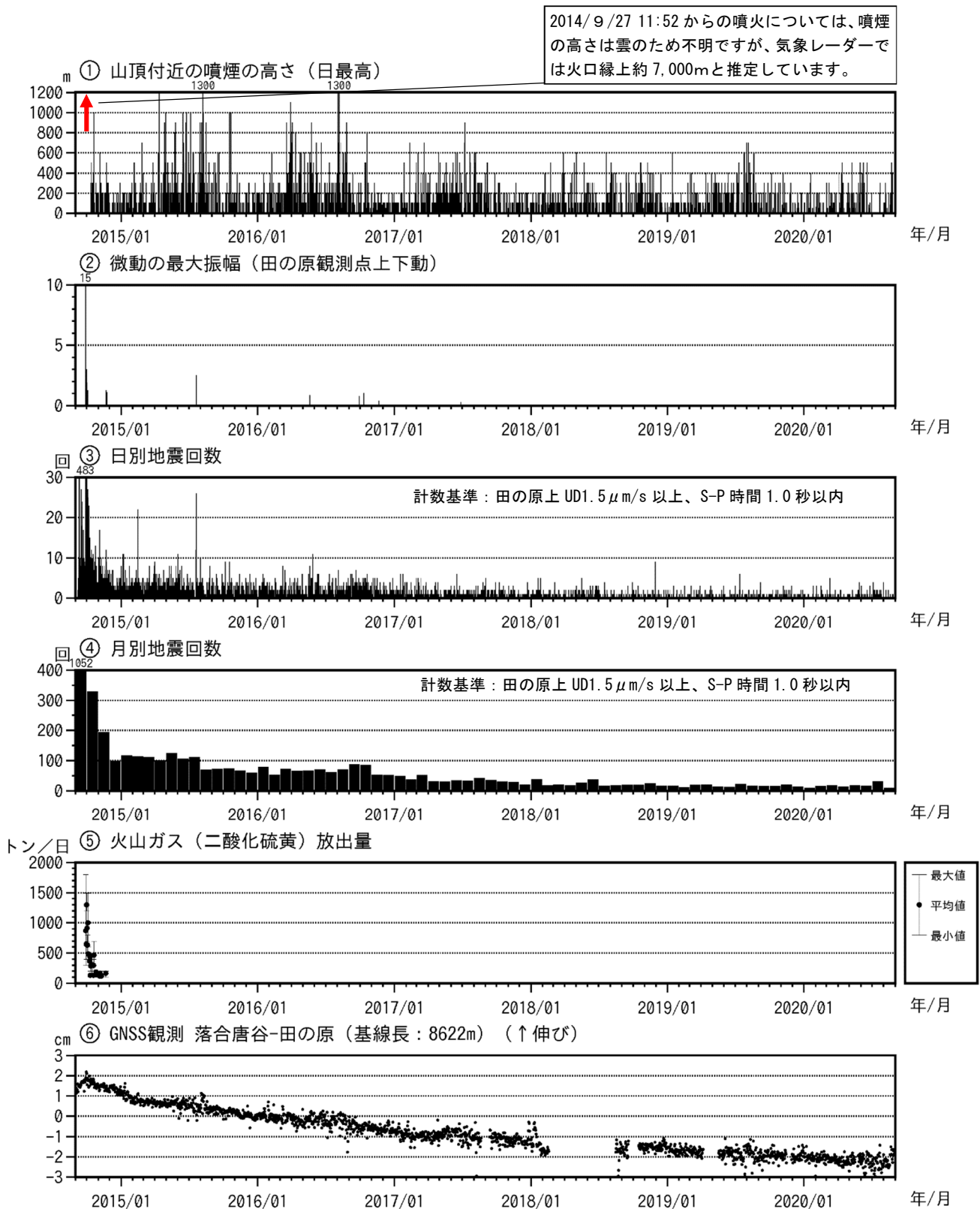
図4 御嶽山 最近の火山活動経過図（2014年9月1日～2020年8月31日）
