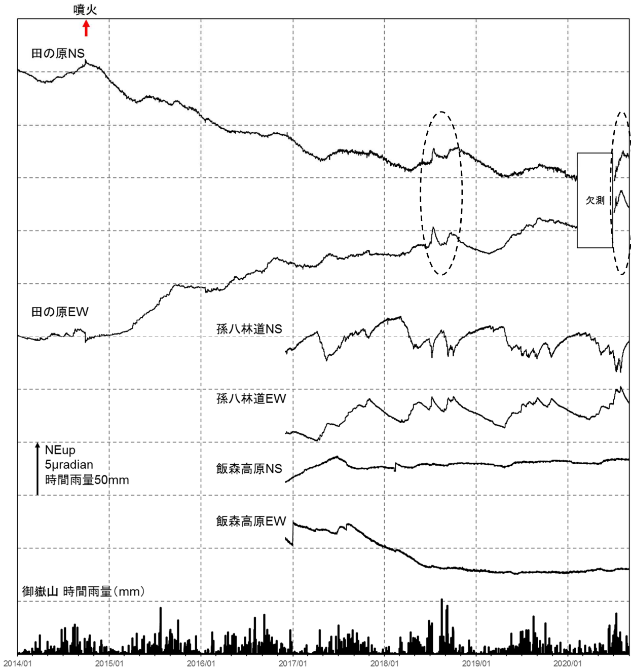
図7 御嶽山 傾斜変動（2014年1月1日～2020年8月31日）
