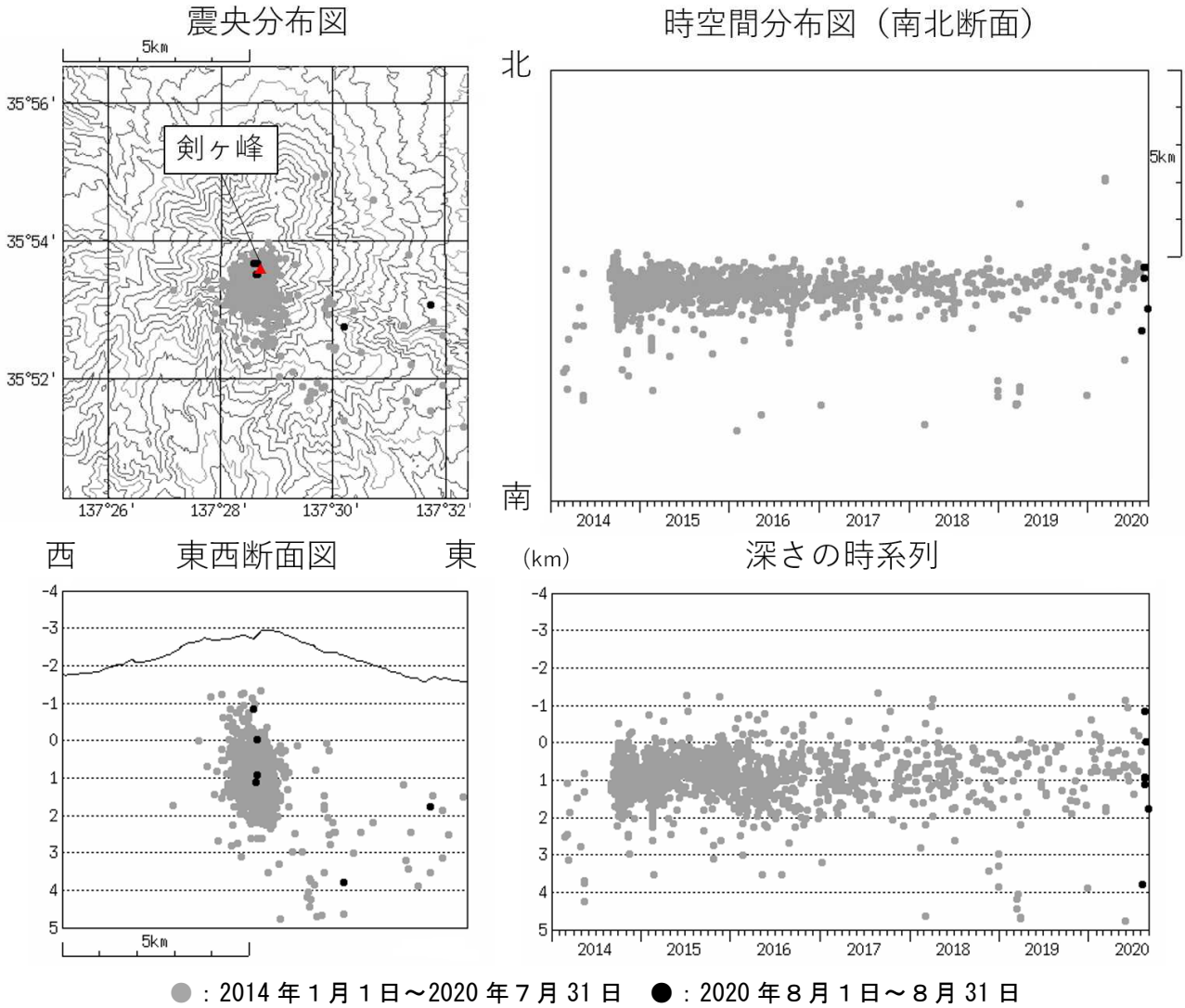
図3 御嶽山 震源分布図（2014年1月1日～2020年8月31日）
