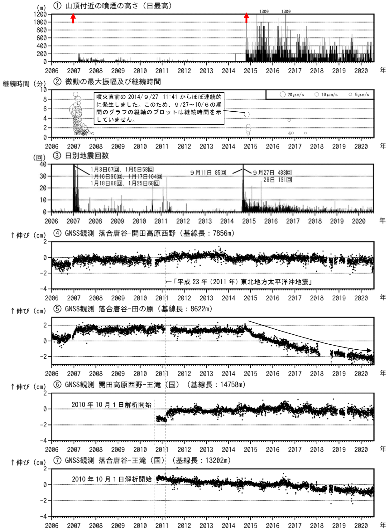
図5 御嶽山 長期間の火山活動経過図（2006年1月1日～2020年8月31日）
