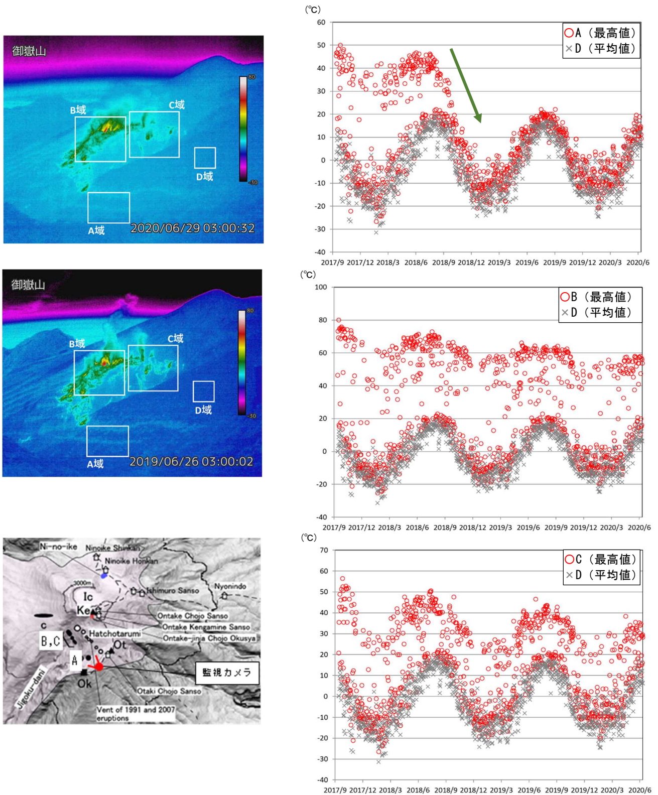
図3 御嶽山 奥の院赤外熱映像カメラによる剣ヶ峰南西側における最高温度の推移 (2017年9月13日～2020年6月30日)と同カメラの位置(左下図はOikawa et al., 2016に加筆) A～Cは地熱域、Dは非地熱域を示します。 ・年周変化はみられるものの、B及びC領域については長期的な低下傾向となっています。 ・A領域の温度は2018年秋頃から明瞭に低下し、非地熱域と同程度の温度となっています(緑矢印)。
