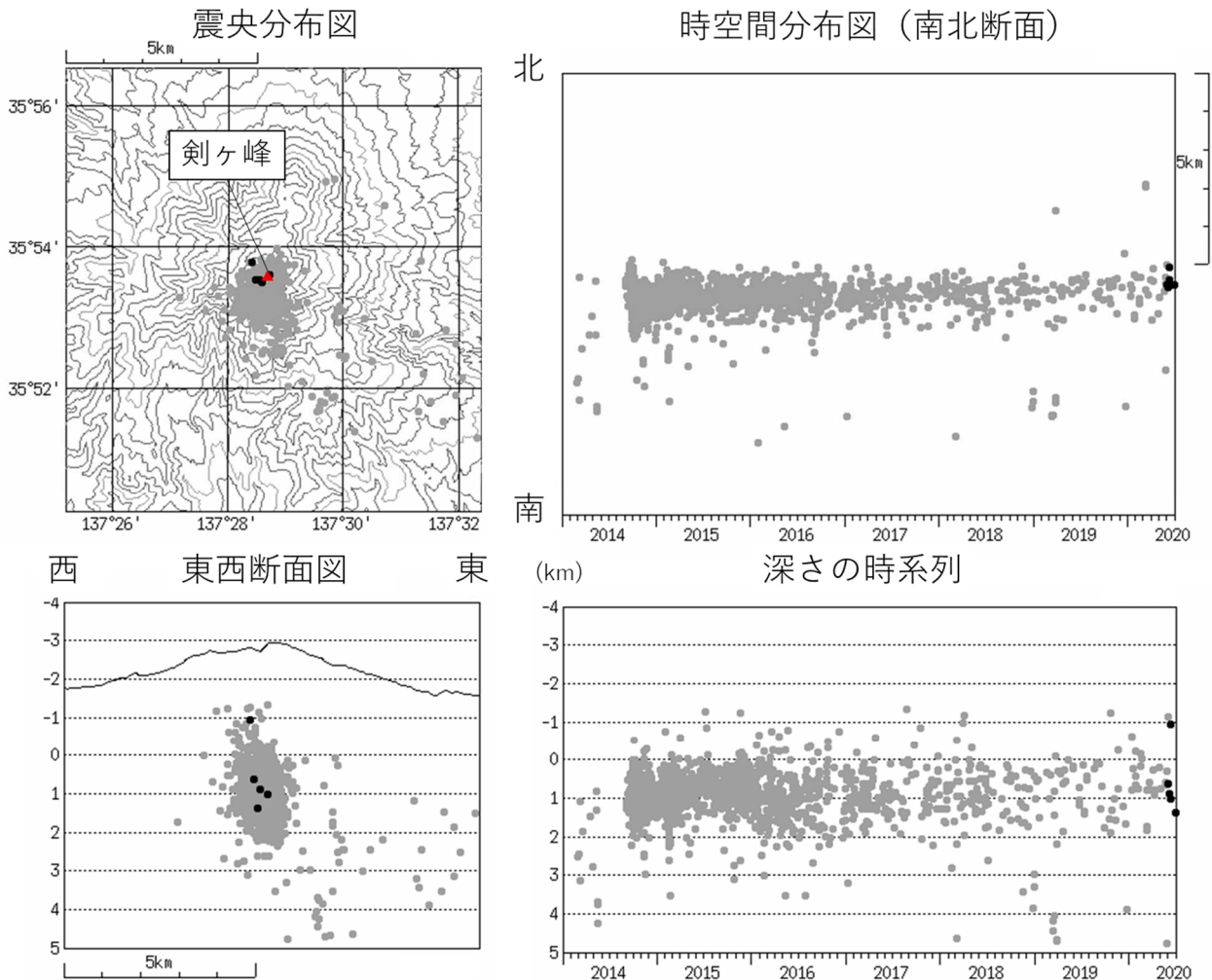
図2 御嶽山 震源分布図（2014年1月1日～2020年6月30日）
