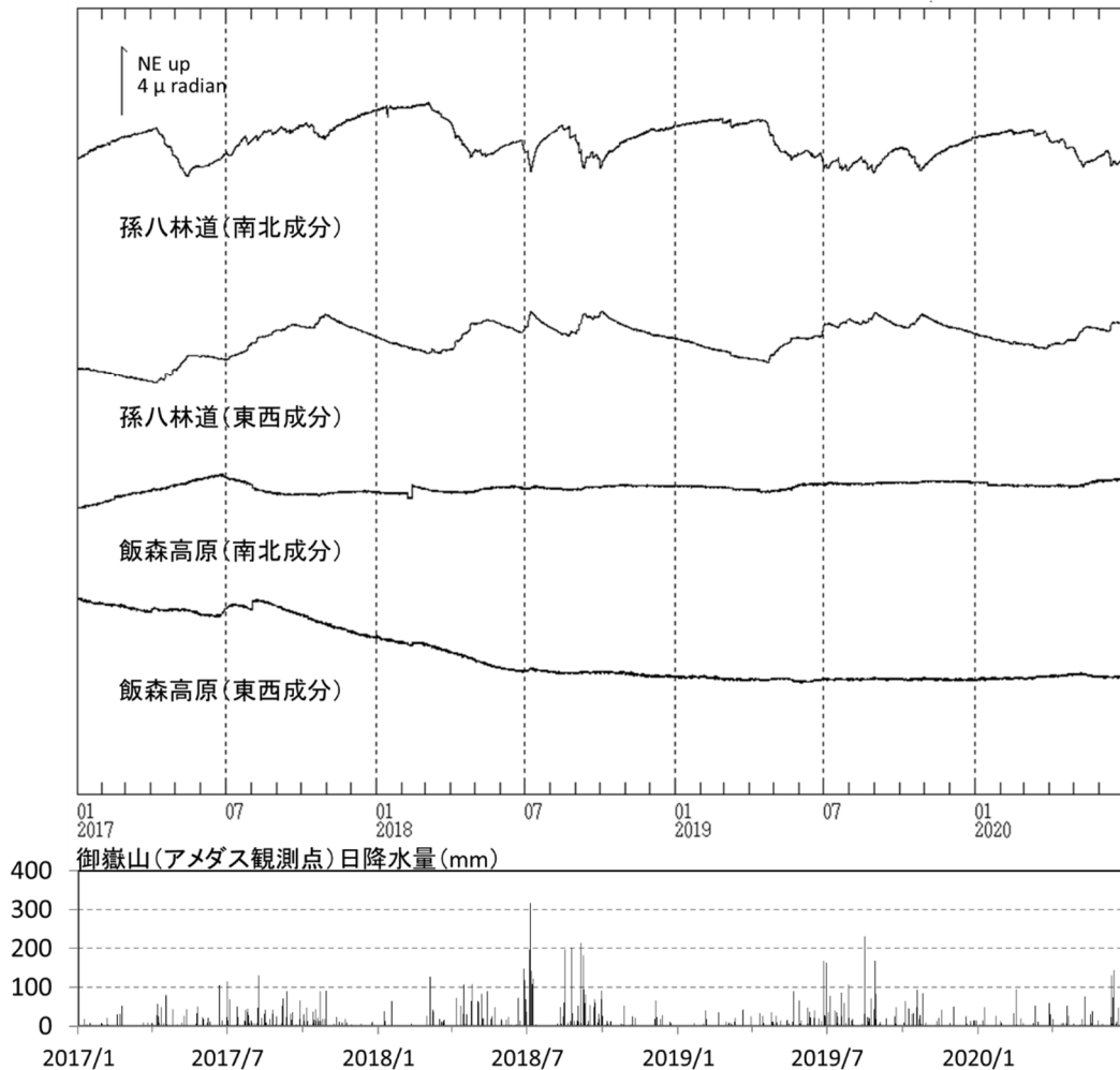
図7 御嶽山 傾斜変動（2017年1月1日～2020年6月30日）
