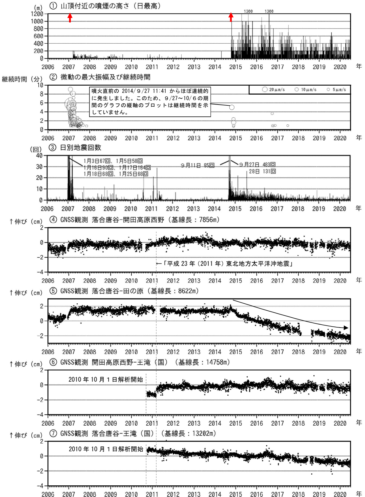
図5 御嶽山 長期間の火山活動経過図（2006年1月1日～2020年6月30日）
