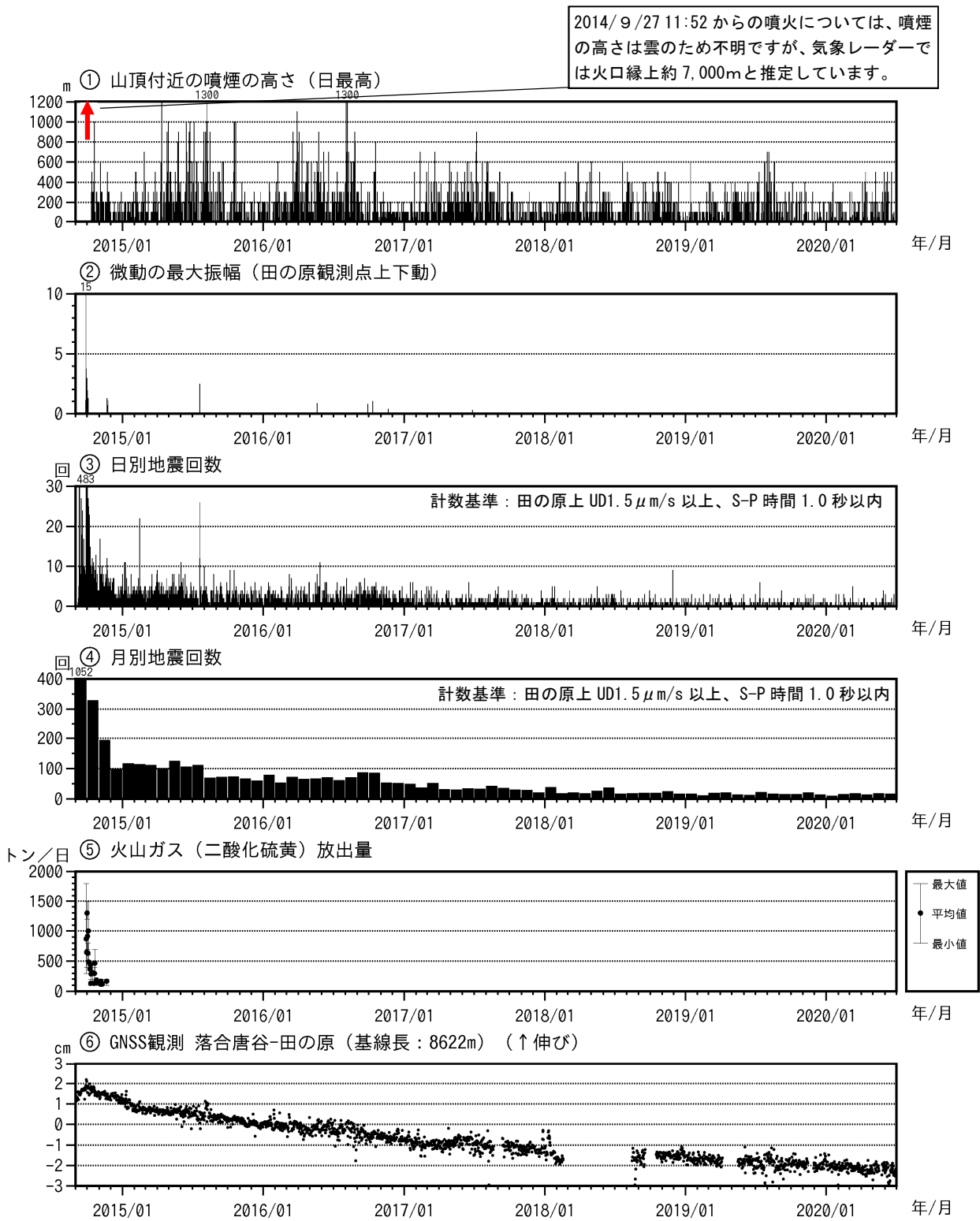
図4 御嶽山 最近の火山活動経過図（2014年9月1日～2020年6月30日）
