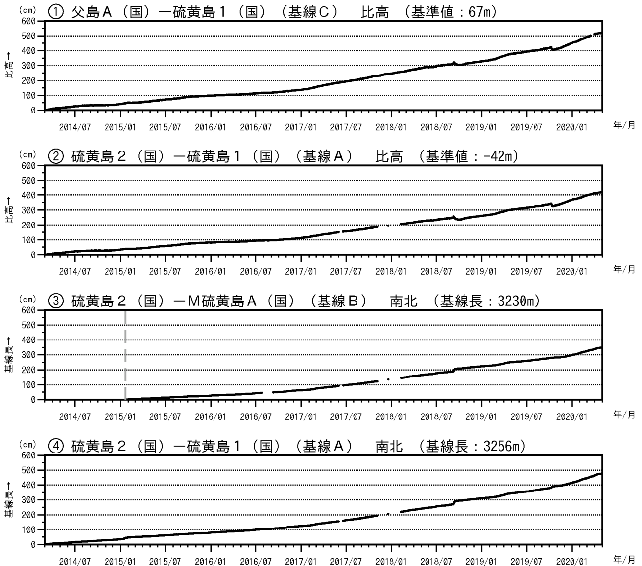
図5 硫黄島 GNSS 連続観測結果（2014年3月1日～2020年4月30日）
