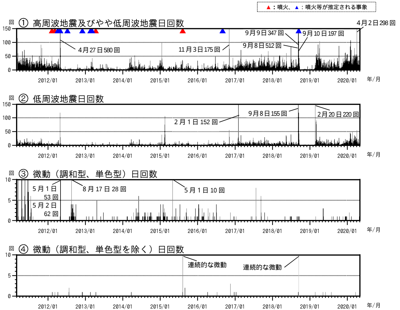
図4 硫黄島 火山活動経過図（2011年3月8日～2020年4月30日）
