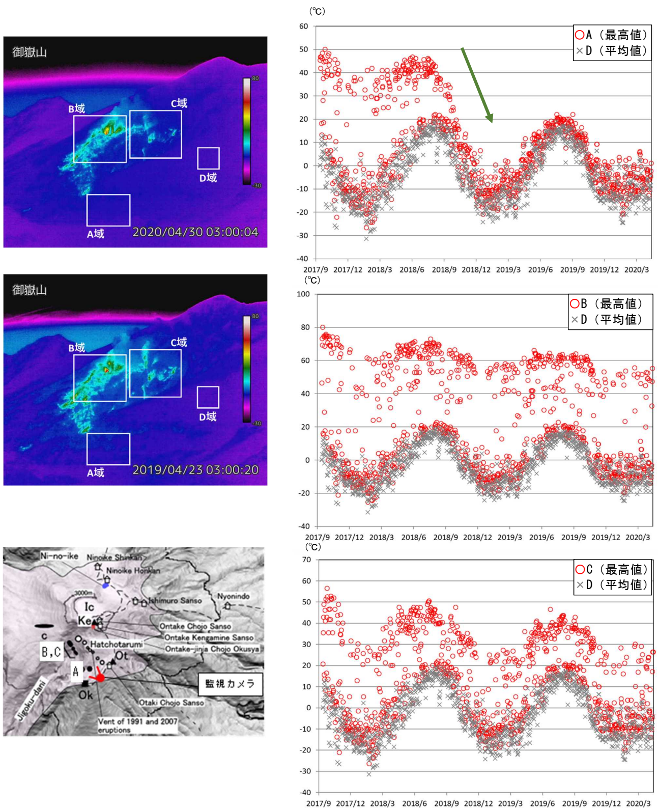
図3 御嶽山 奥の院赤外線熱映像カメラによる剣ヶ峰南西側における最高温度の推移
