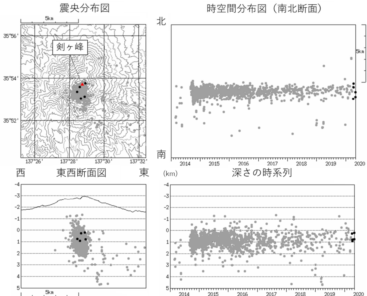
図2 御嶽山 震源分布図（2014年1月1日～2020年4月30日）
