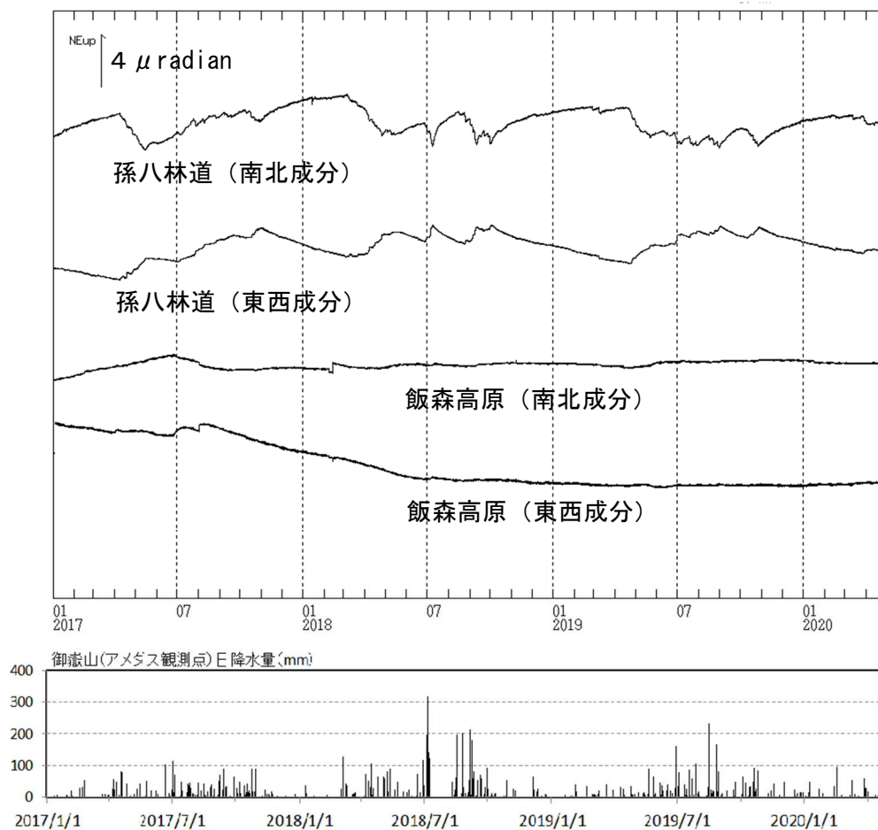
図7 御嶽山 傾斜変動（2017年1月1日～2020年4月30日）
