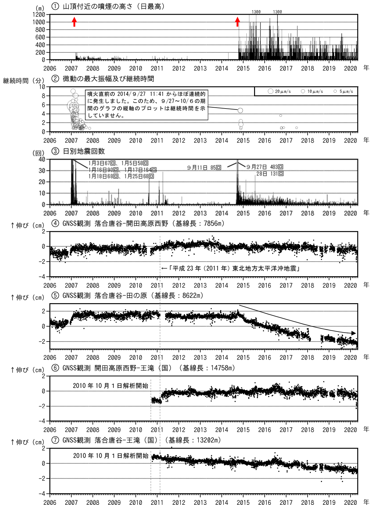
図5 御嶽山 長期間の火山活動経過図（2006年1月1日～2020年4月30日）
