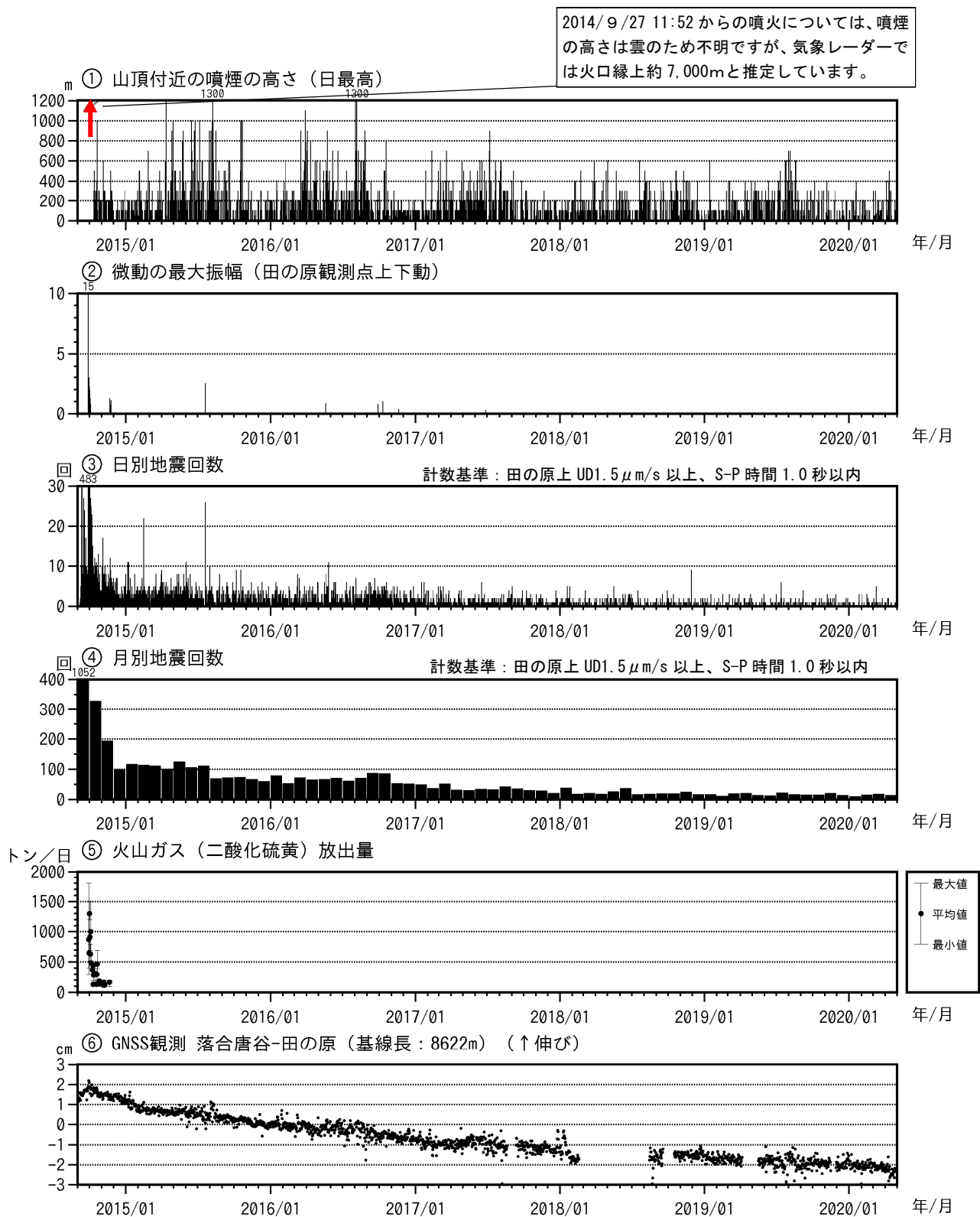
図4 御嶽山 最近の火山活動経過図（2014年9月1日～2020年4月30日）
