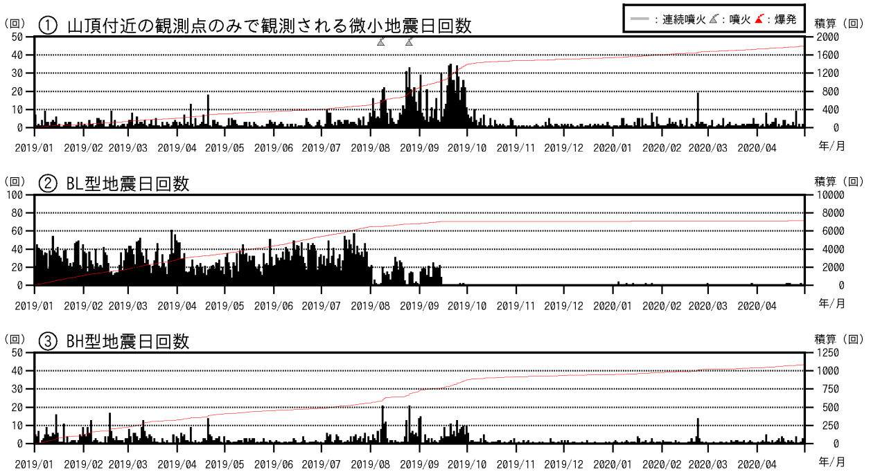
図5 浅間山 火山性地震の発生状況（2019年1月1日～2020年4月30日）
