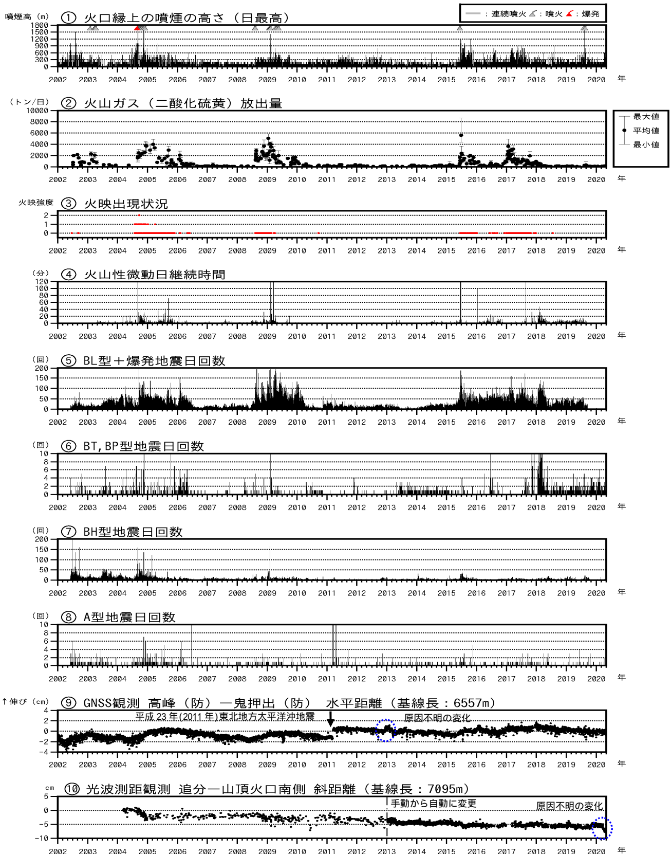
図3 浅間山 火山活動経過図（2002年1月1日～2020年4月30日）
