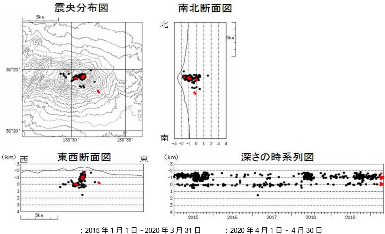
図6 浅間山 震源分布図（2015年1月1日～2020年4月30日）
