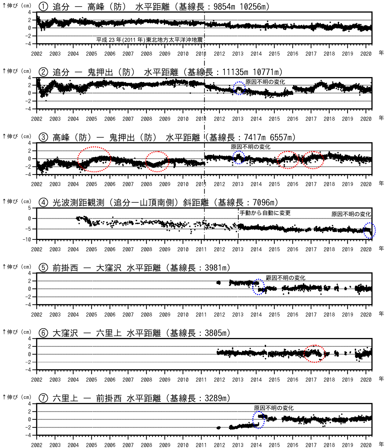
図7-1 浅間山 GNSS連続観測及び光波測距観測の結果(2002年1月1日~2020年4月30日) 2010年10月及び2016年1月に、解析方法を変更しています。
