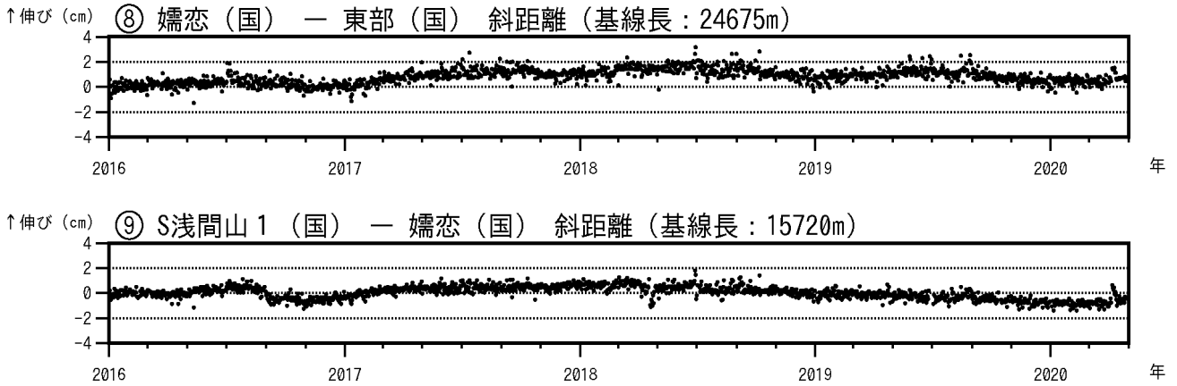
図7 - 2 浅間山 GNSS連続観測結果(2016年1月1日~2020年4月30日) (国): 国土地理院 、 は図8の にそれぞれ対応しています。 、 の空白部分は欠測を示します。
