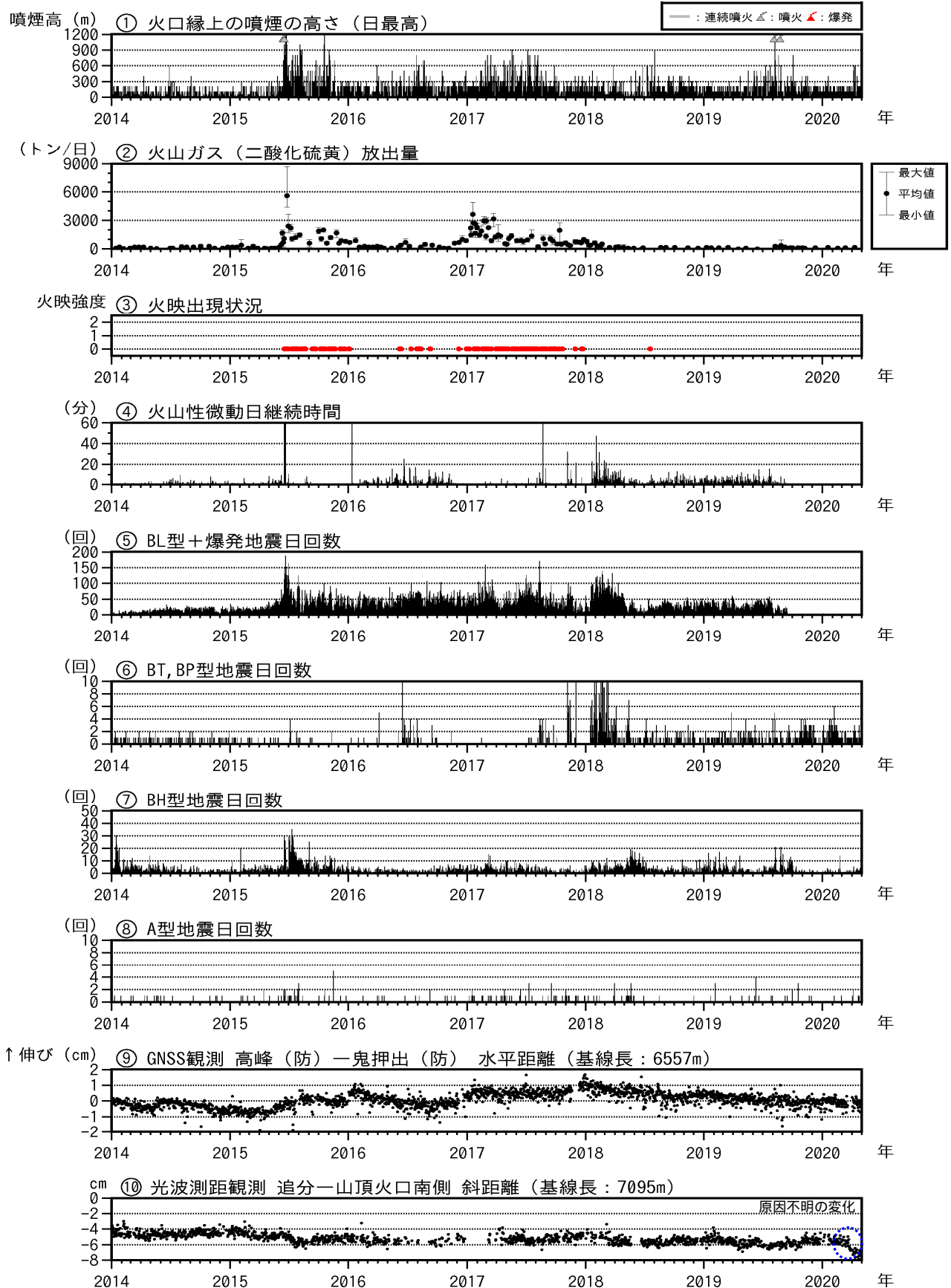
図4 浅間山 最近の火山活動経過図（2014年1月1日～2020年4月30日）
