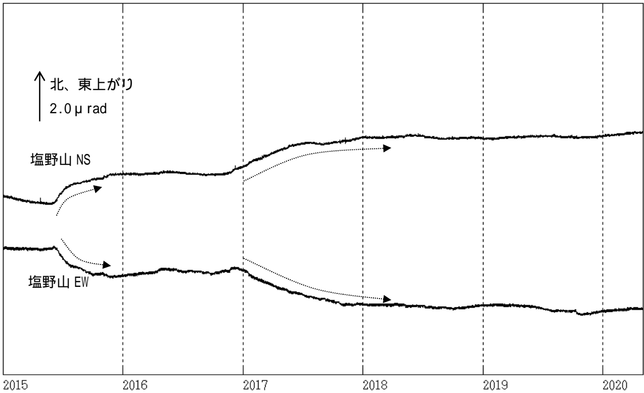
図9 浅間山 塩野山観測点における傾斜データ（2015年1月1日～2020年4月30日）
