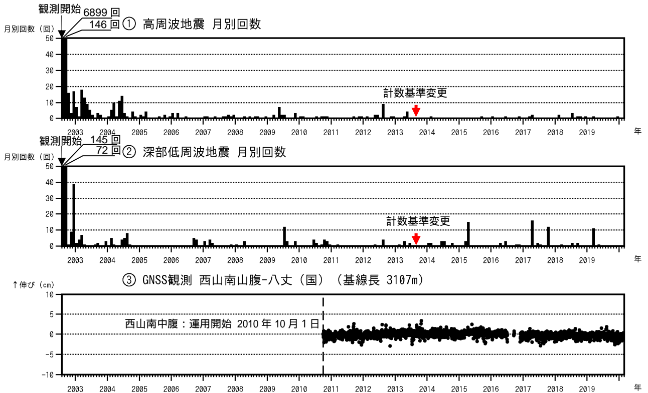
図2 八丈島 火山活動経過図（2002年8月13日～2020年2月29日）
