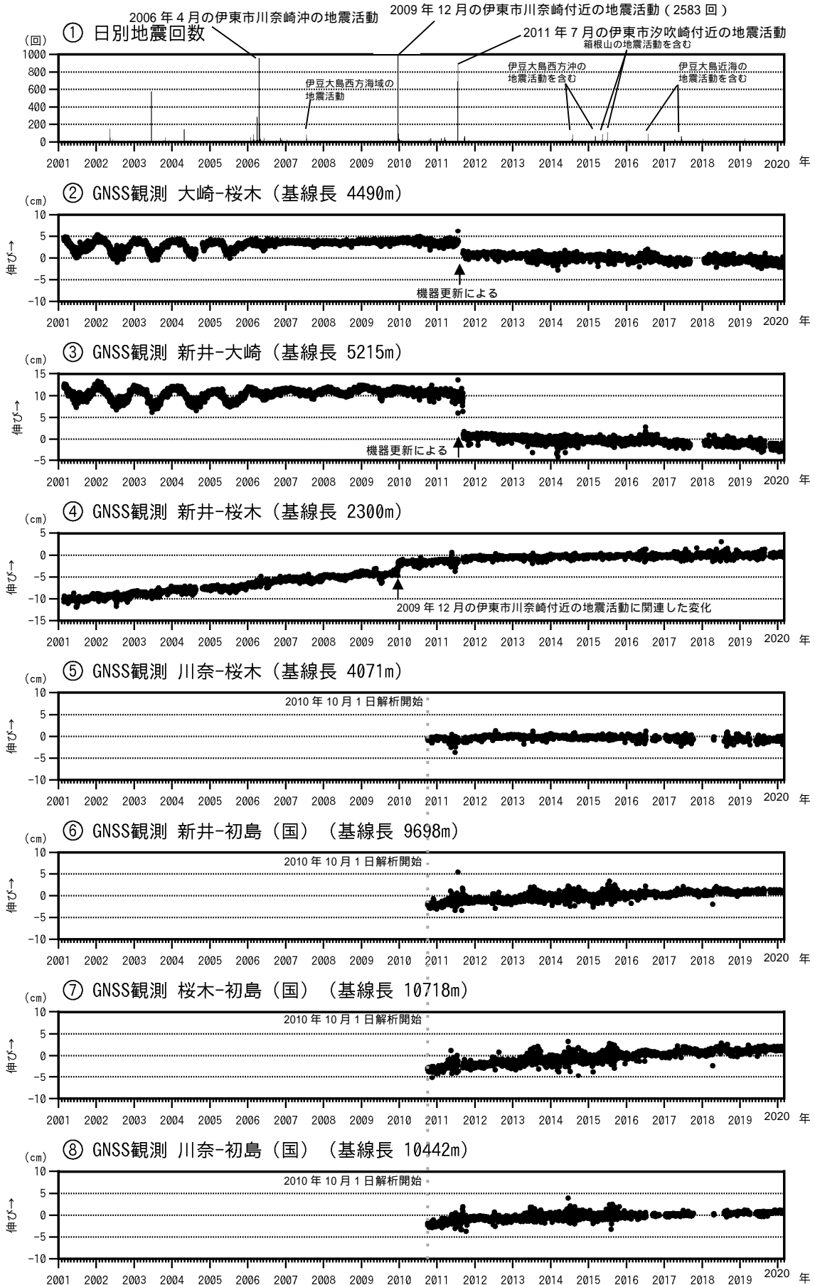
図3 伊豆東部火山群 火山活動経過図（2001年1月1日～2020年2月29日） : 2012年7月23日までは鎌田2、それ以降は鎌田3地震観測点による。 ~ (国): 国土地理院。図4のGNSS基線 ~ に対応。グラフの空白部分は欠測を示す。 2010年10月及び2016年1月以降のデータは解析方法を変更しています。 基線長変化に見られる周期的な変動は季節変動と考えられます。
