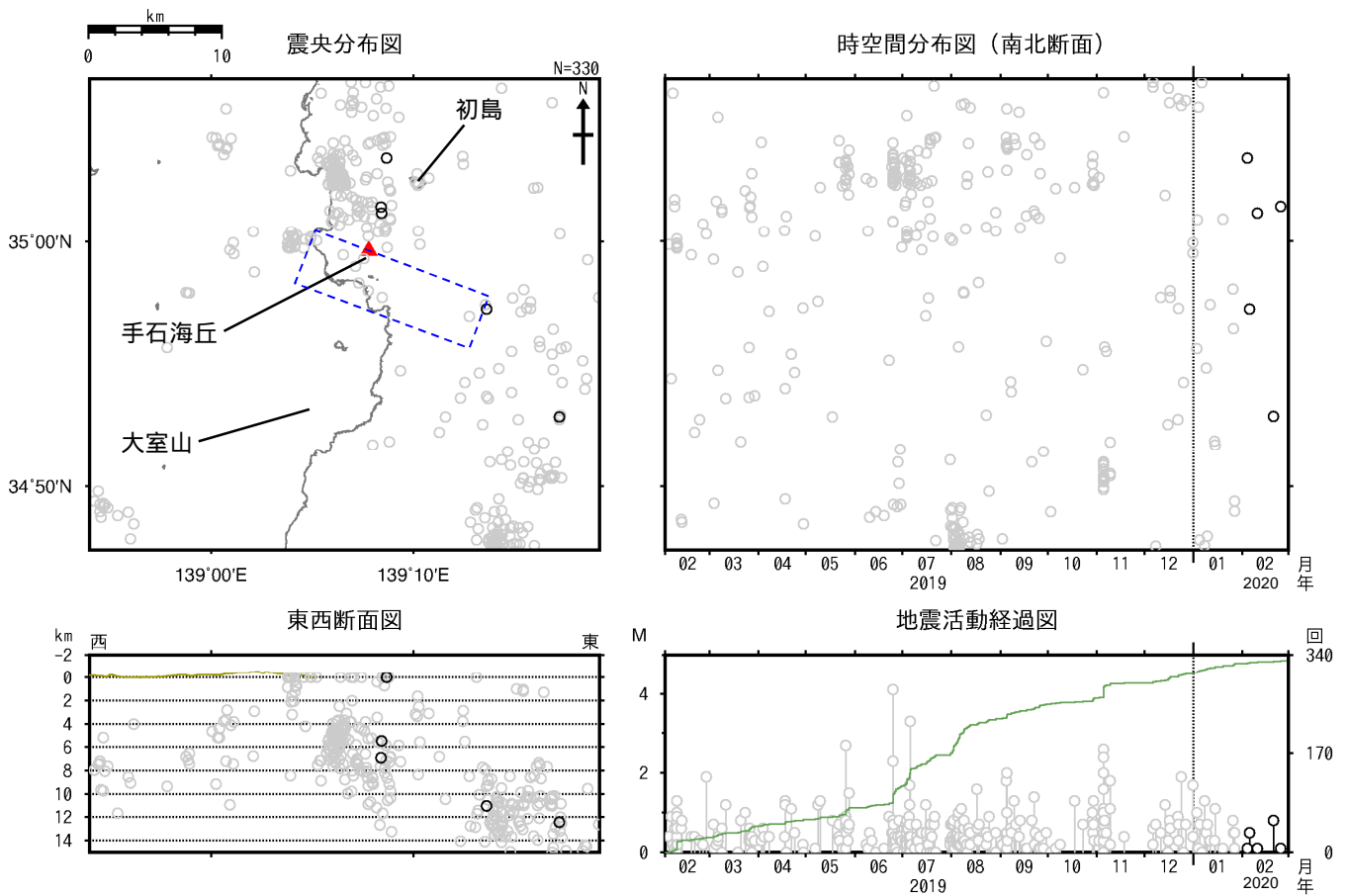
図2 伊豆東部火山群 広域地震観測網による震源分布図（2019年2月1日～2020年2月29日）
