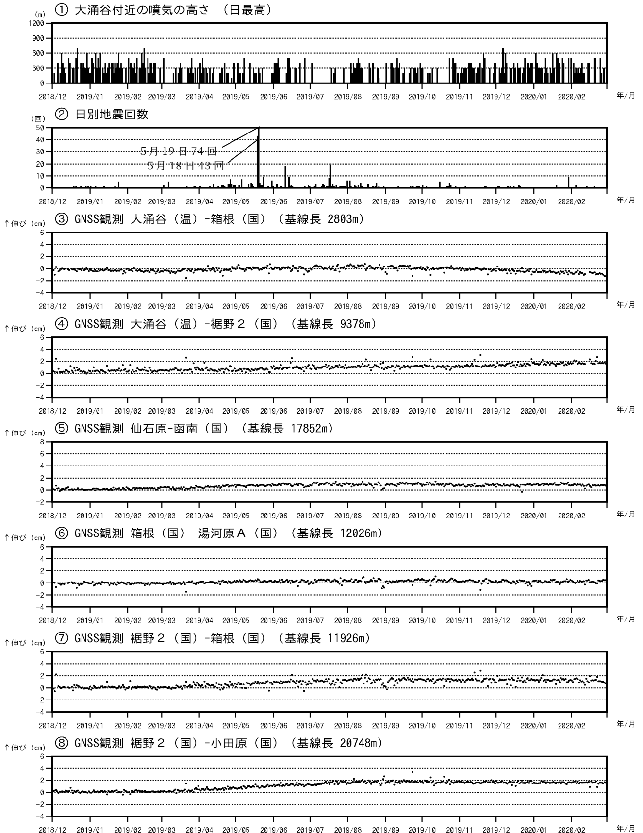
図7 箱根山 火山活動経過図（2018年12月1日～2020年2月29日）
