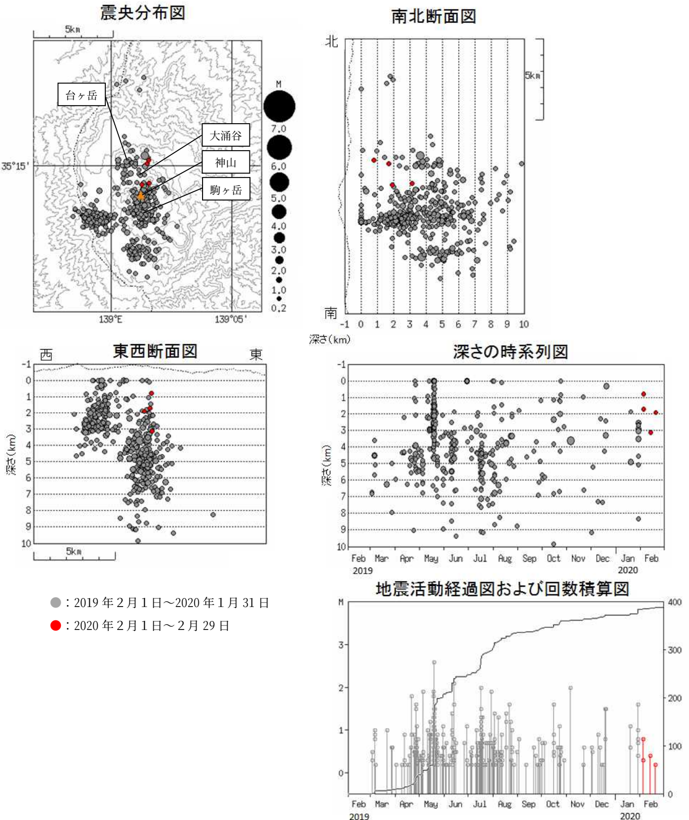
図8 箱根山 広域地震観測網による山体周辺の震源分布図(2019年2月1日～2020年2月29日)
