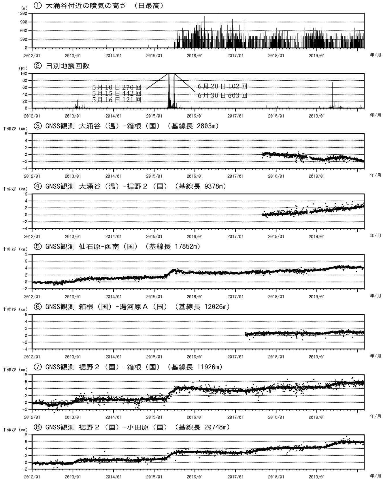
図6 箱根山 火山活動経過図（2012年1月1日～2020年2月29日）
