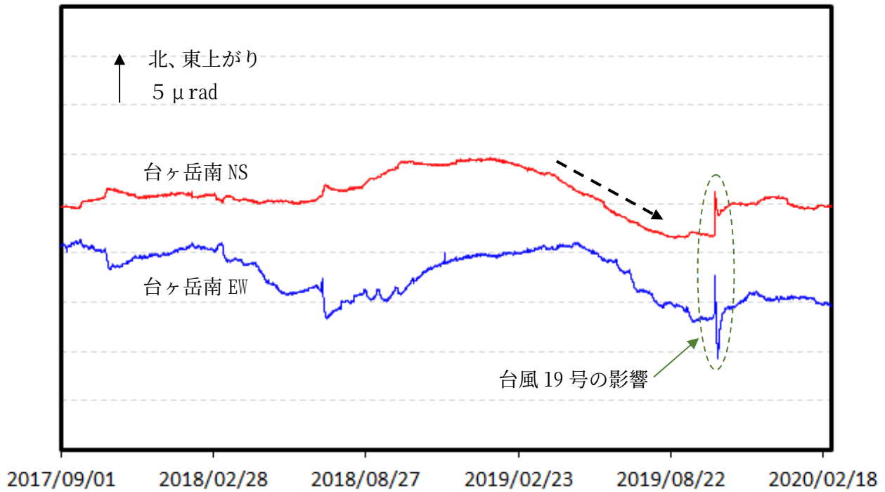
図9 箱根山 台ヶ岳南観測点における傾斜データ（2017年9月1日～2020年2月29日）
