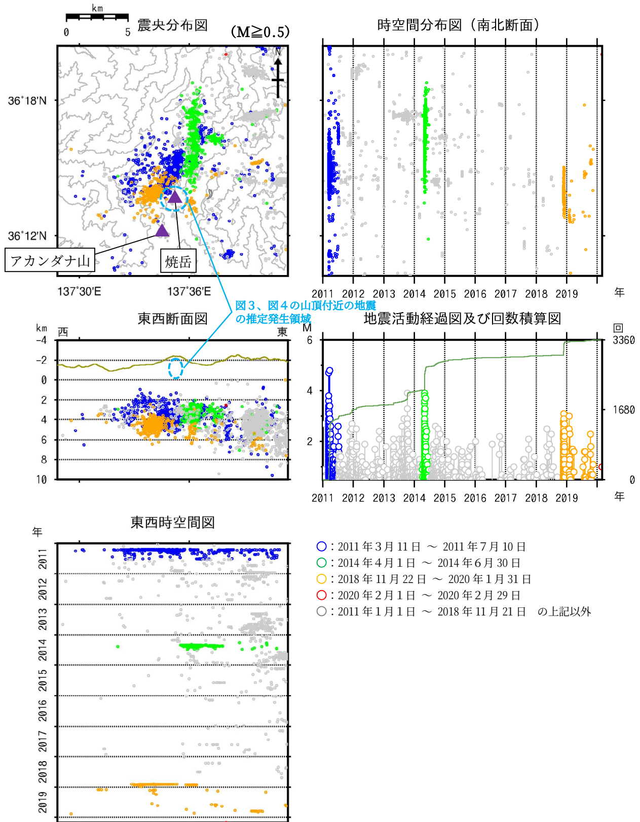
図5 焼岳 広域地震観測網による山体及び周辺の地震活動(2011年1月1日～2020年2月29日)
