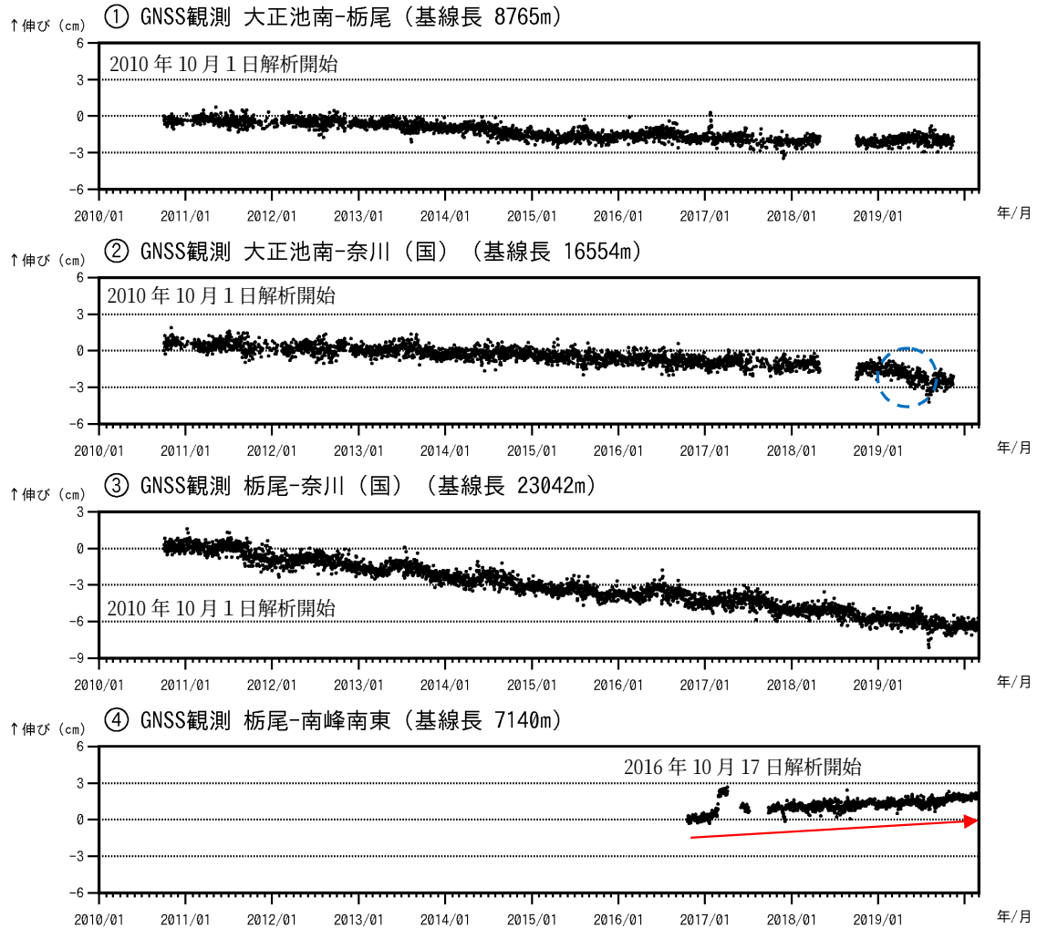
図6 焼岳 GNSS 連続観測による基線長変化（2010年10月1日～2020年2月29日）
