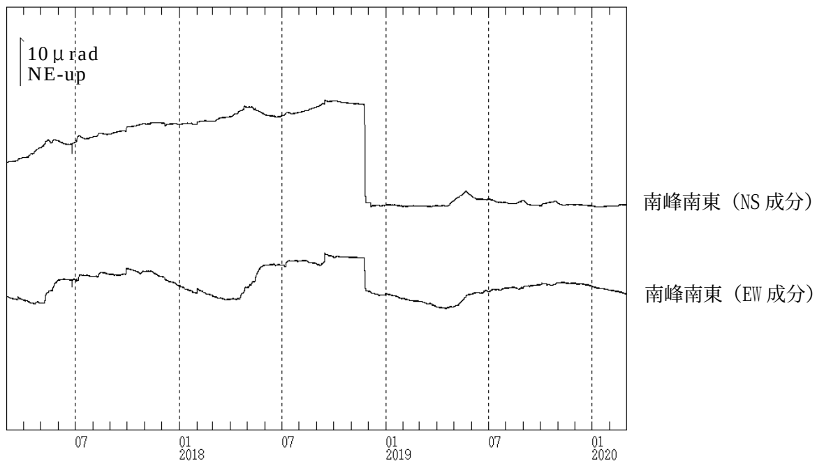
図7 焼岳 南峰南東観測点における傾斜データ（2017年3月1日～2020年2月29日）
