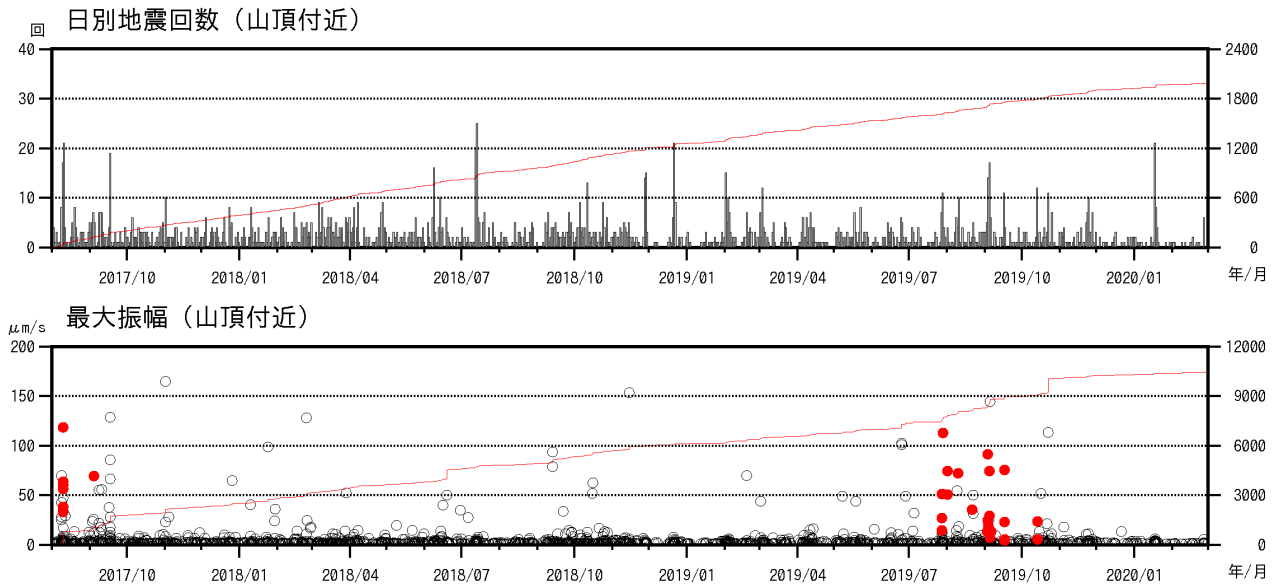
図4 焼岳 山頂付近の地震回数、および南峰南東観測点上下動最大振幅 (2017年8月1日～2020年2月29日)
