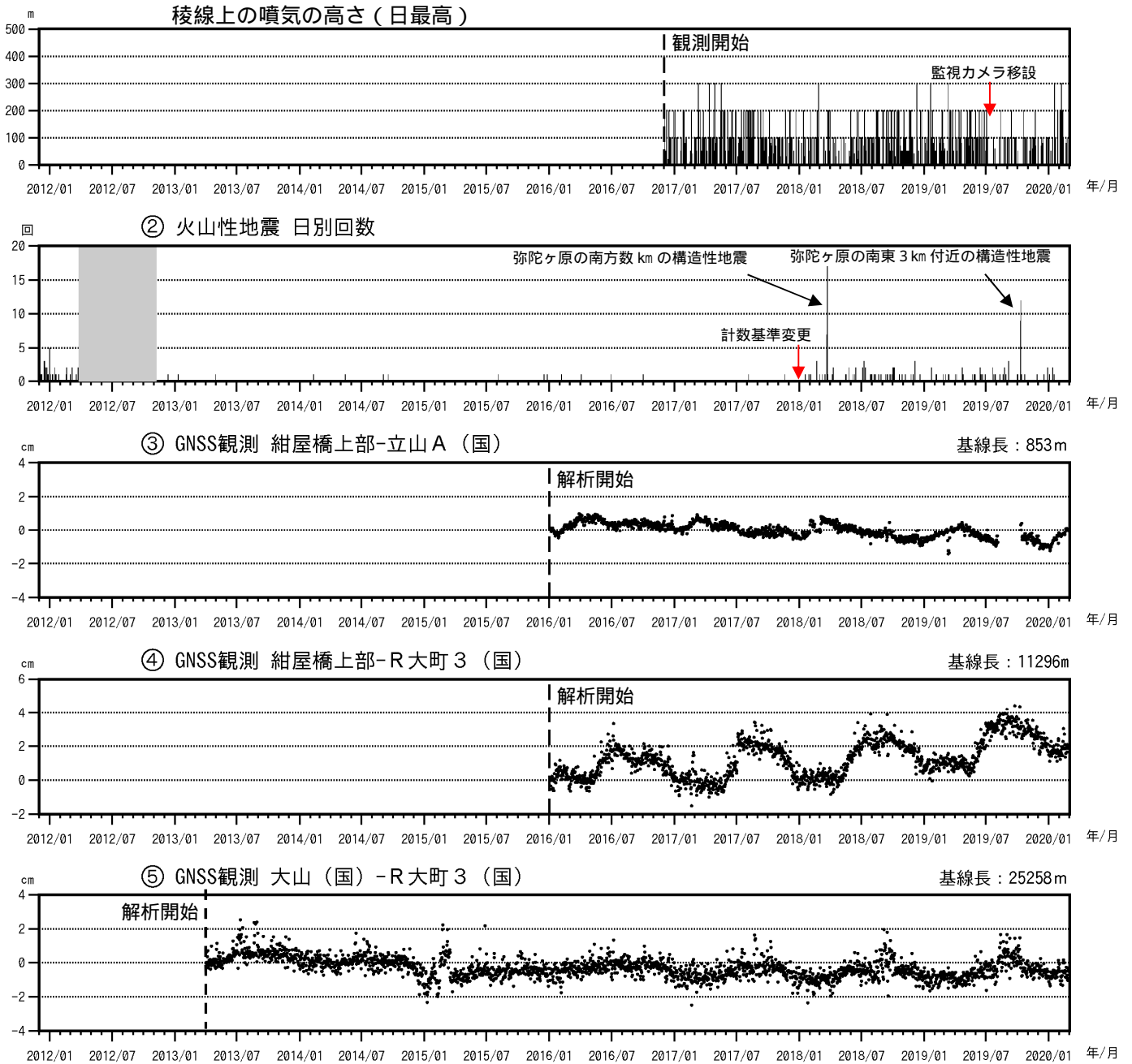
図2 弥陀ヶ原 火山活動経過図（2011年12月1日～2020年2月29日）
