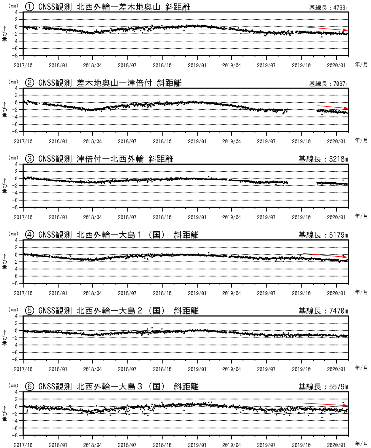
図3-2 伊豆大島 GNSS連続観測による基線長変化(2017年10月～2020年1月31日)
