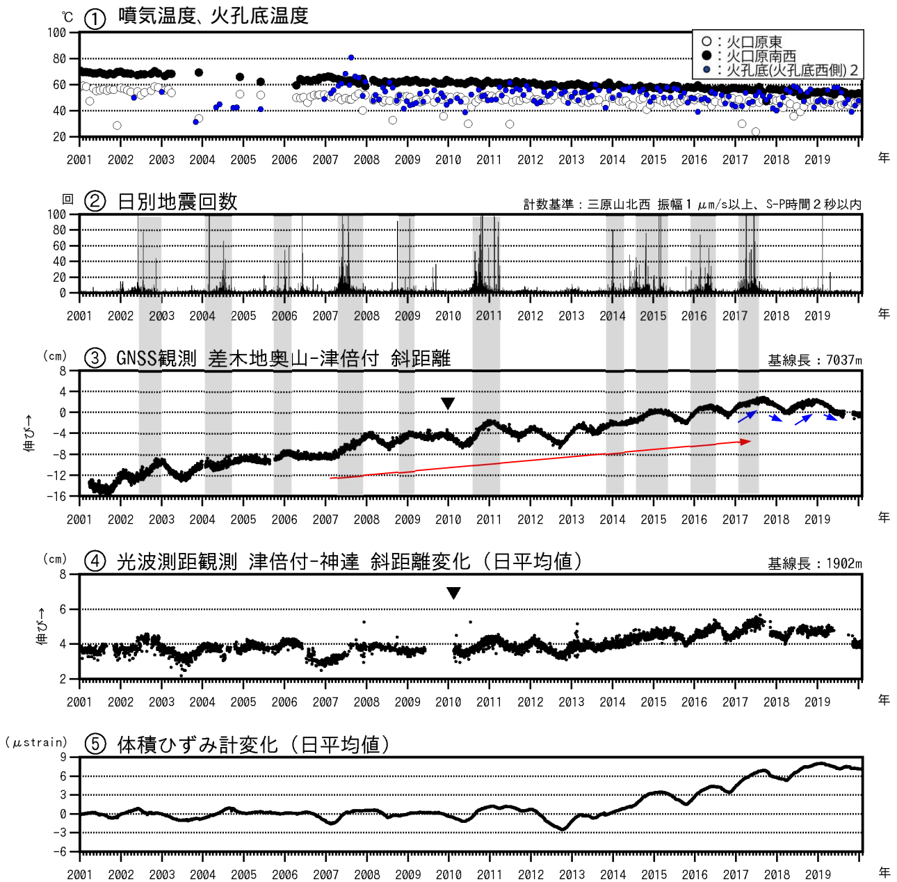
図2 伊豆大島 最近の火山活動経過図（2001年1月～2020年1月31日）
