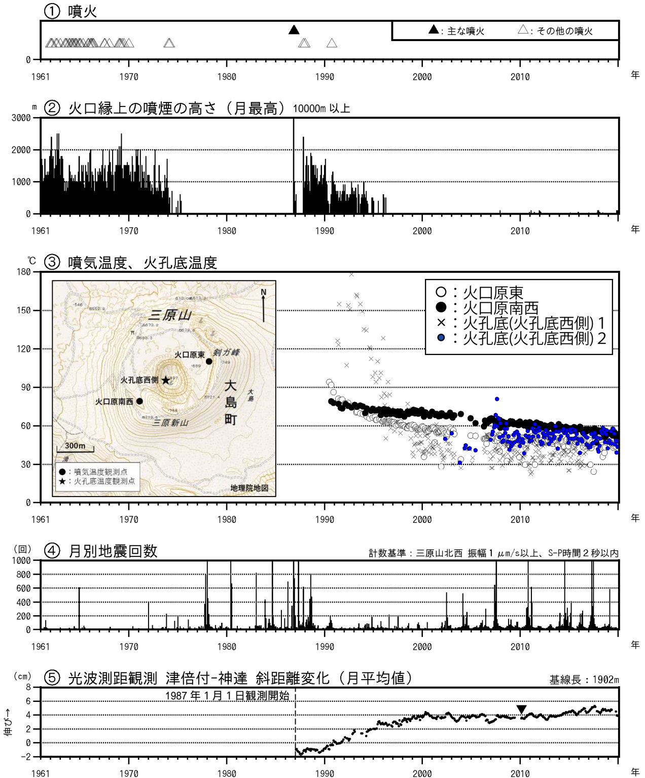
図1 伊豆大島 長期間の火山活動経過図 (1961年1月~2020年1月31日)
