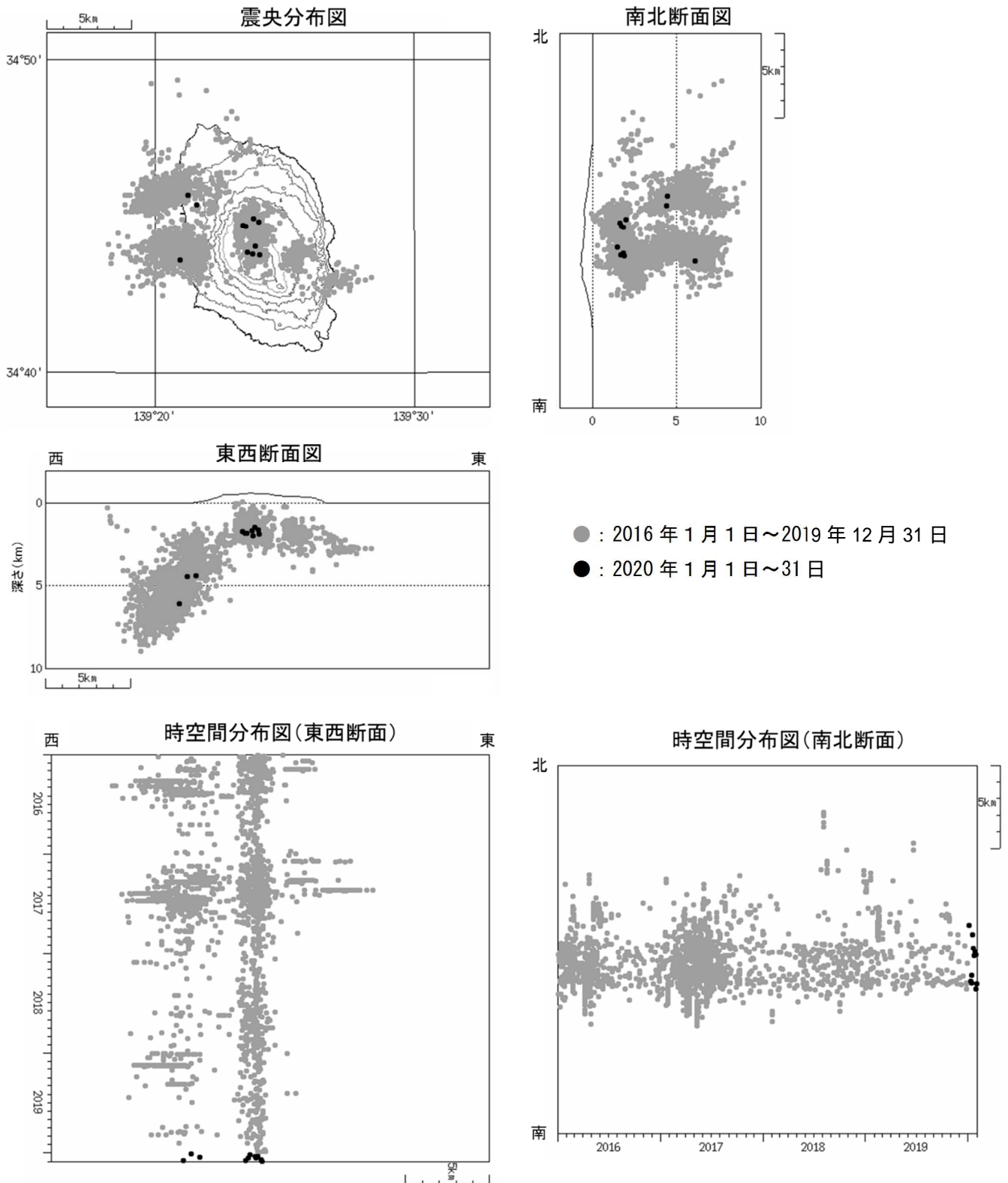
図4 伊豆大島 震源分布図（2016年1月1日～2020年1月31日）
