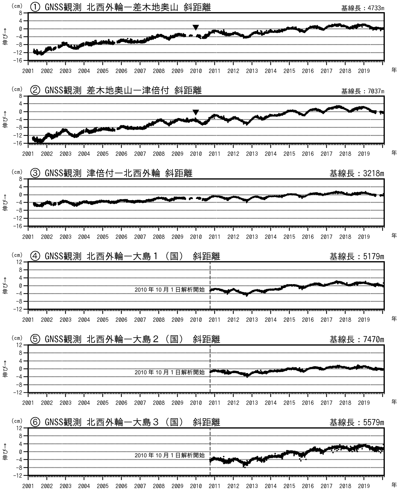
図3-1 伊豆大島 GNSS連続観測による基線長変化(2001年1月~2020年1月31日)
