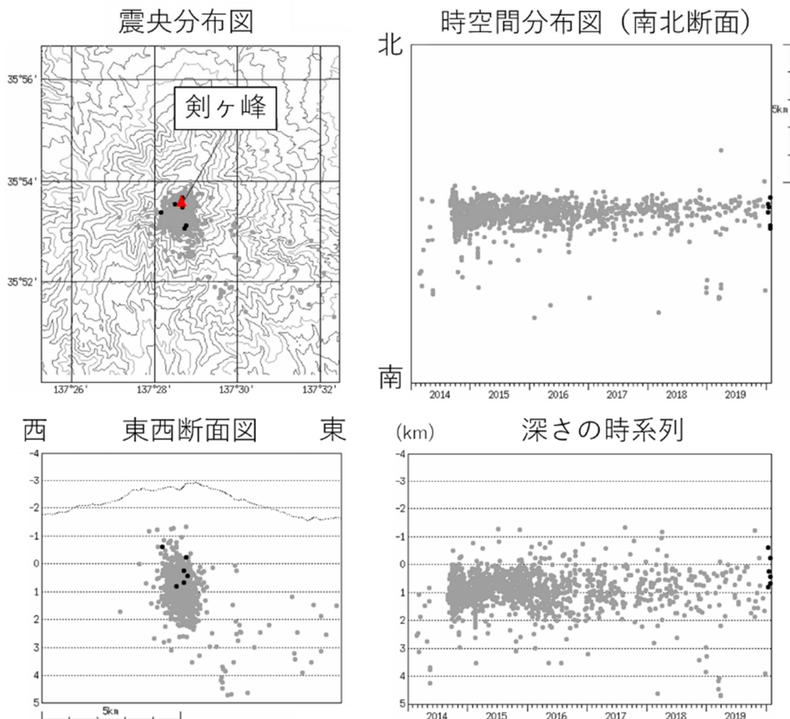
図2 御嶽山 震源分布図（2014年1月1日～2020年1月31日）
