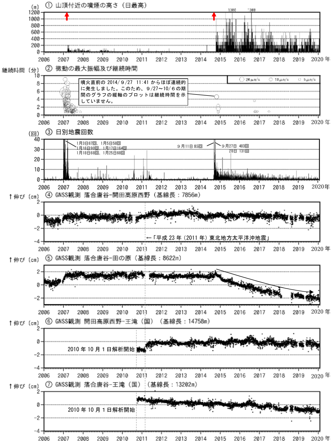
図5 御嶽山 長期間の火山活動経過図（2006年1月1日～2020年1月31日）
