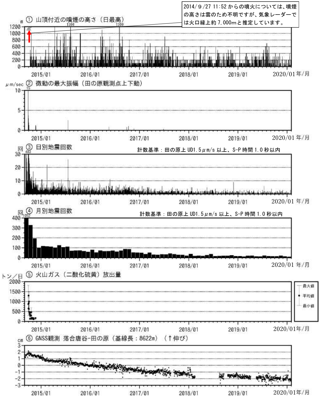
図4 御嶽山 最近の火山活動経過図（2014年9月1日～2020年1月31日）
