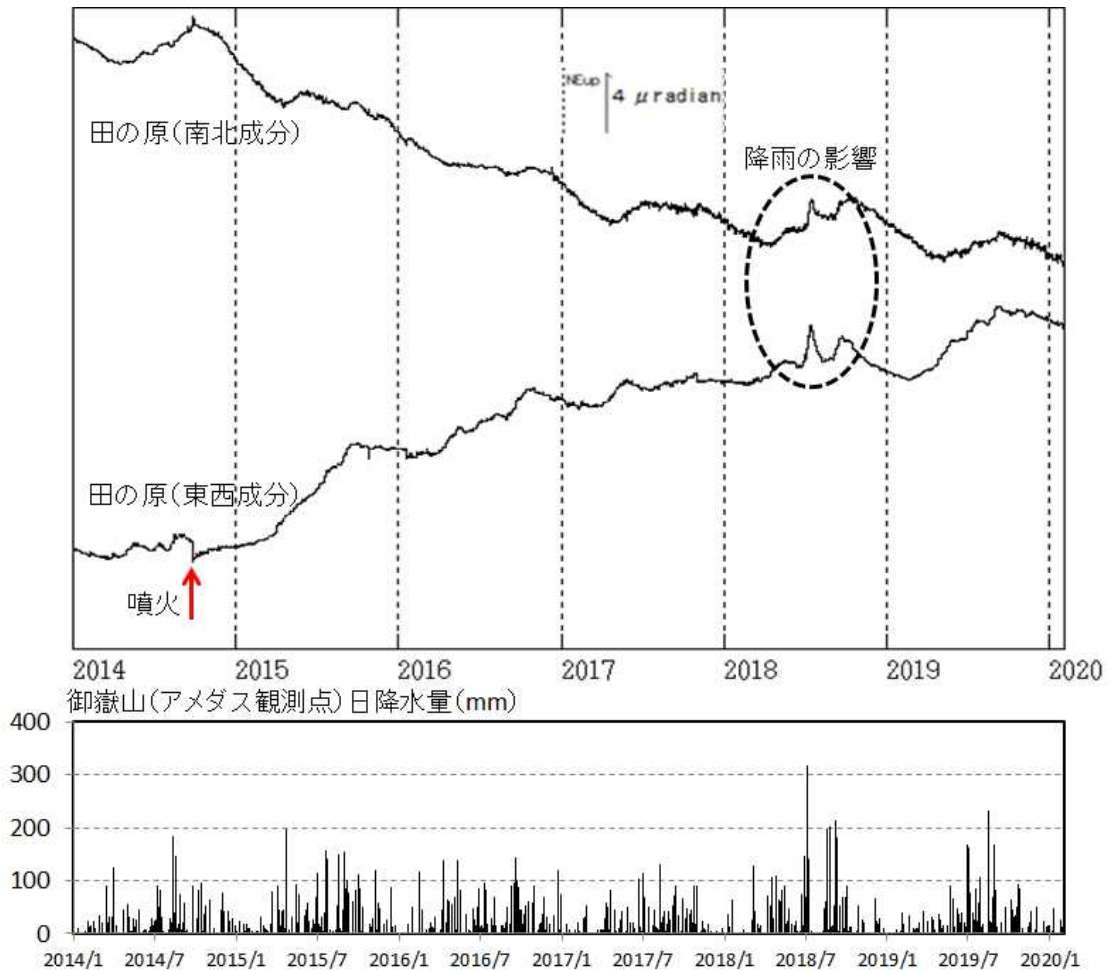
図7 御嶽山 田の原観測点の傾斜変動（2014年1月1日～2020年1月31日）
