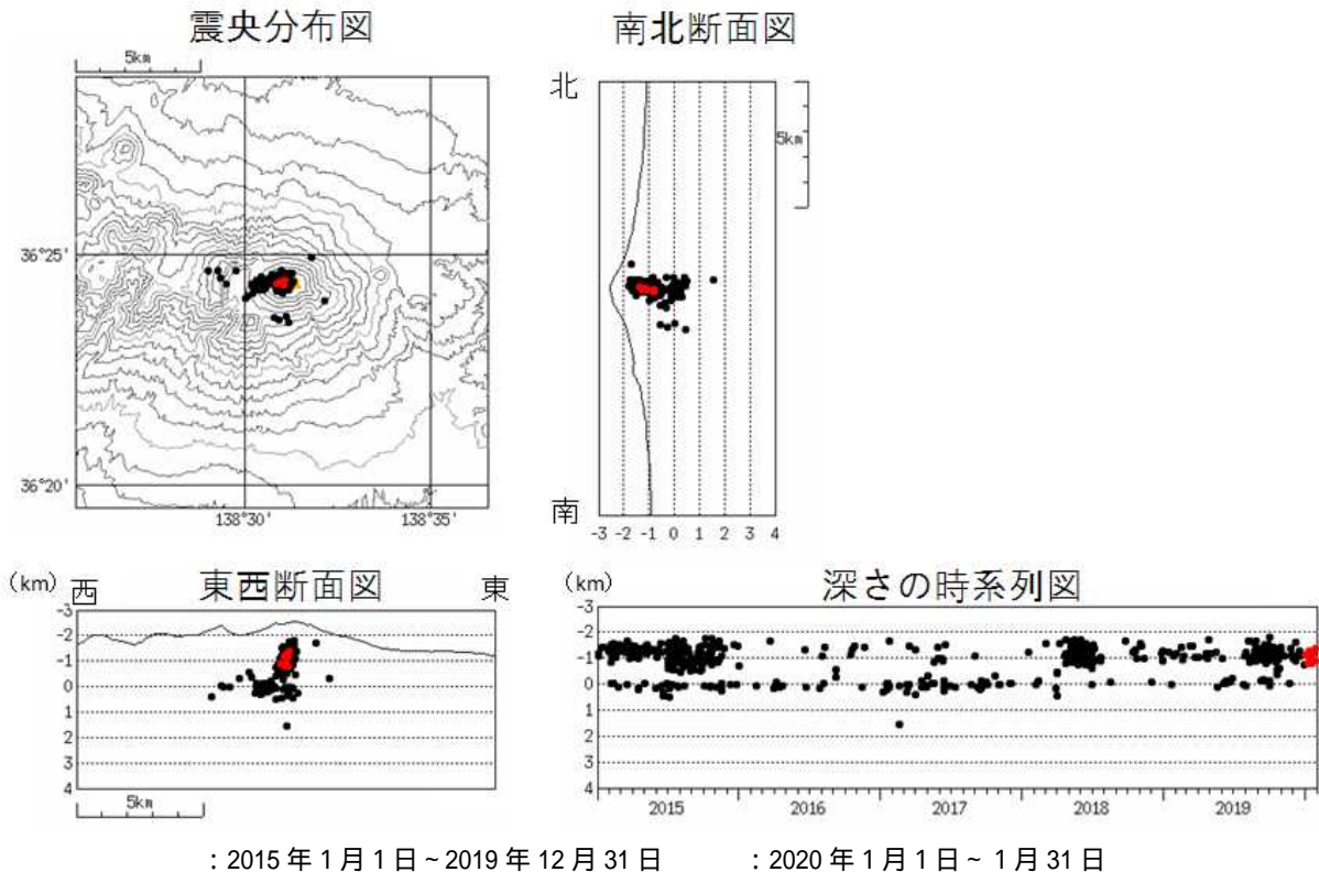
図6 浅間山 震源分布図（2015年1月1日～2020年1月31日）
