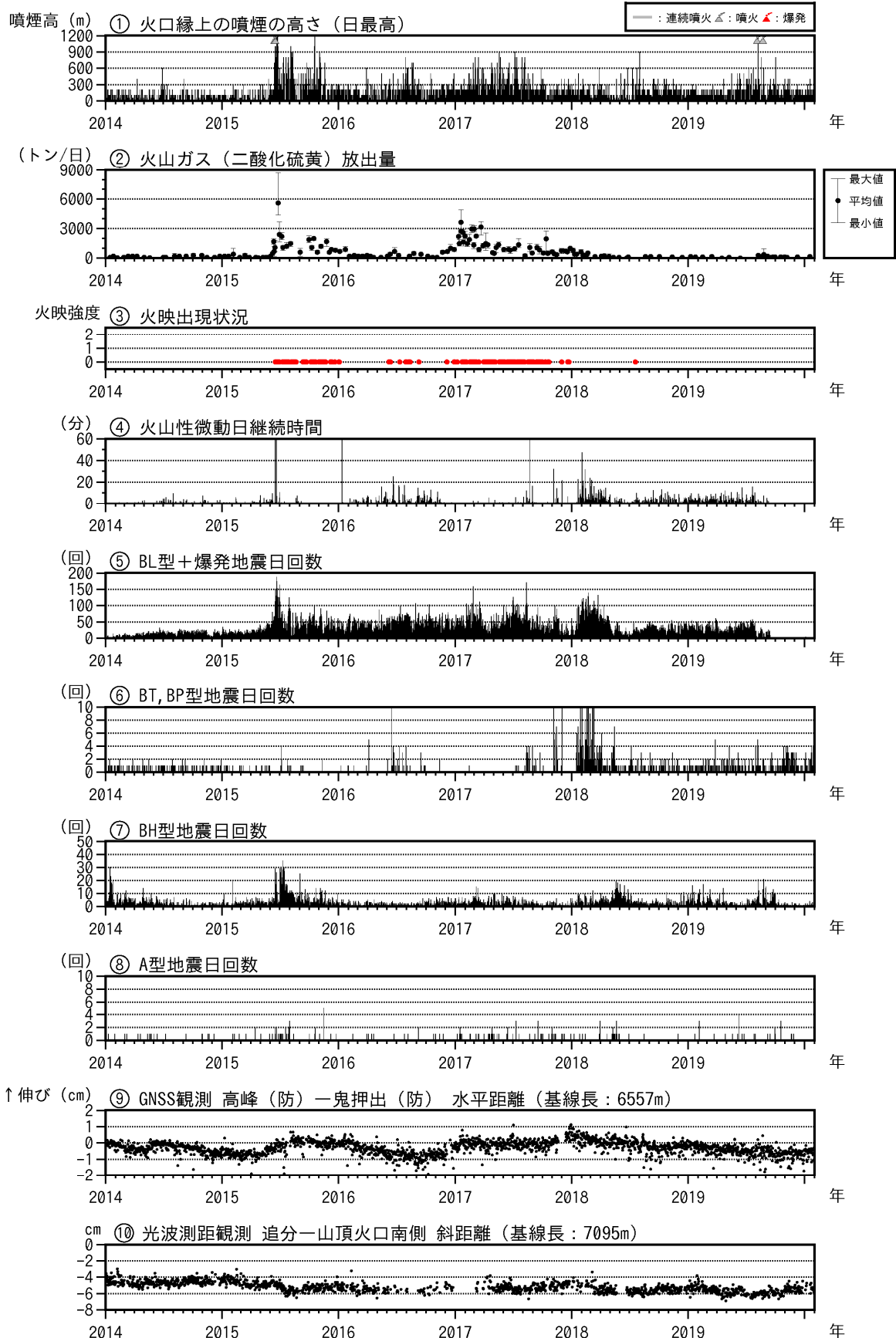
図4 浅間山 最近の火山活動経過図（2014年1月1日～2020年1月31日）
