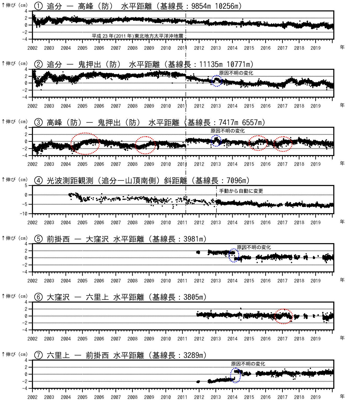
図7-1 浅間山 GNSS 連続観測及び光波測距観測の結果(2002年1月1日~2020年1月31日) 2010年10月及び2016年1月に、解析方法を変更しています。
