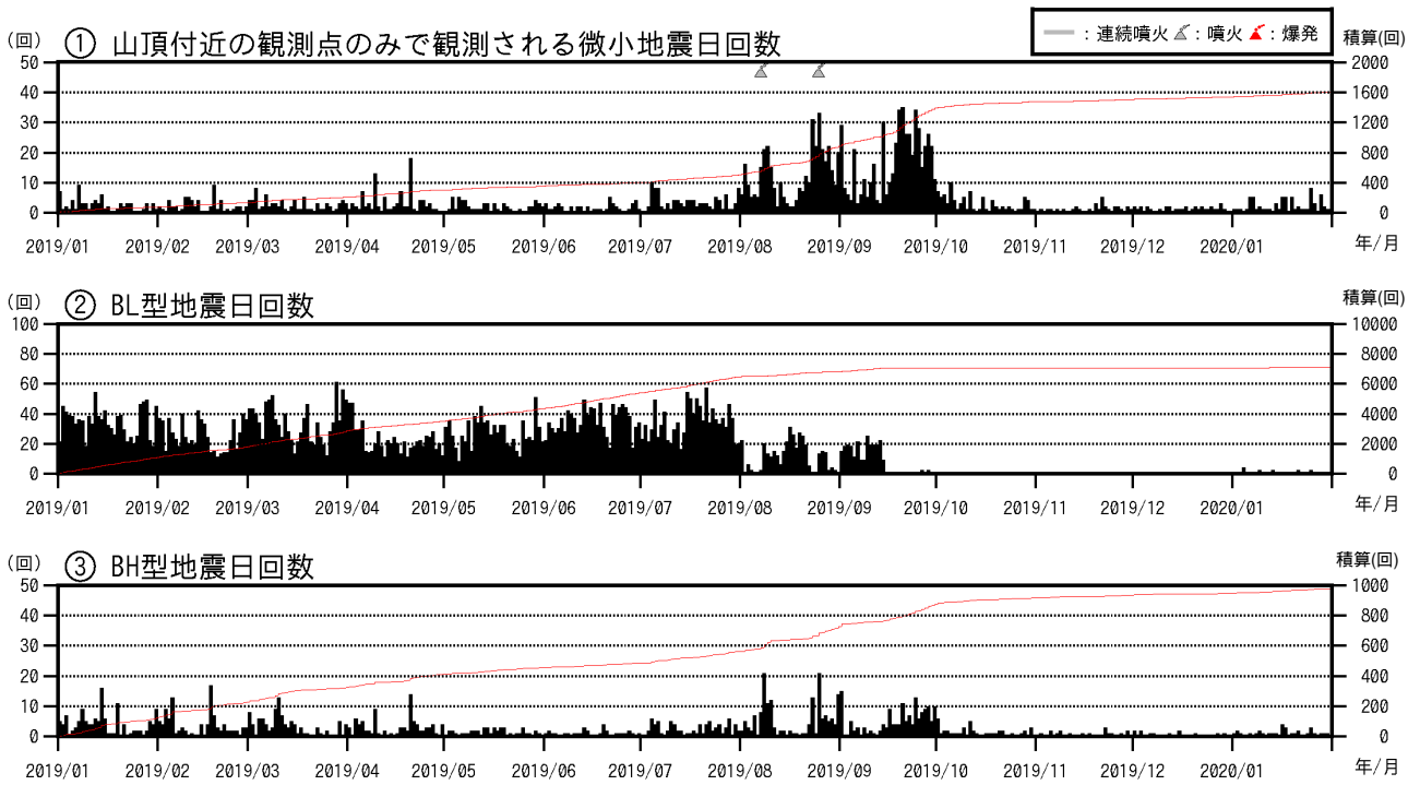
図5 浅間山 火山性地震の発生状況（2019年1月1日～2020年1月31日）
