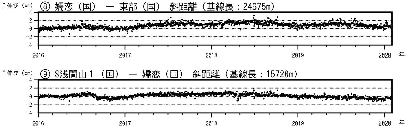
図7 - 2 浅間山 GNSS 連続観測結果(2016年1月1日~2020年1月31日)
