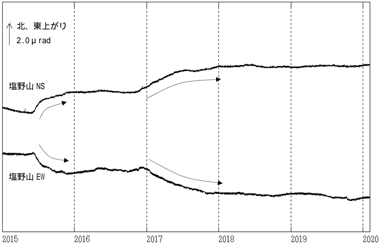
図9 浅間山 塩野山観測点における傾斜データ（2015年1月1日～2020年1月31日）
