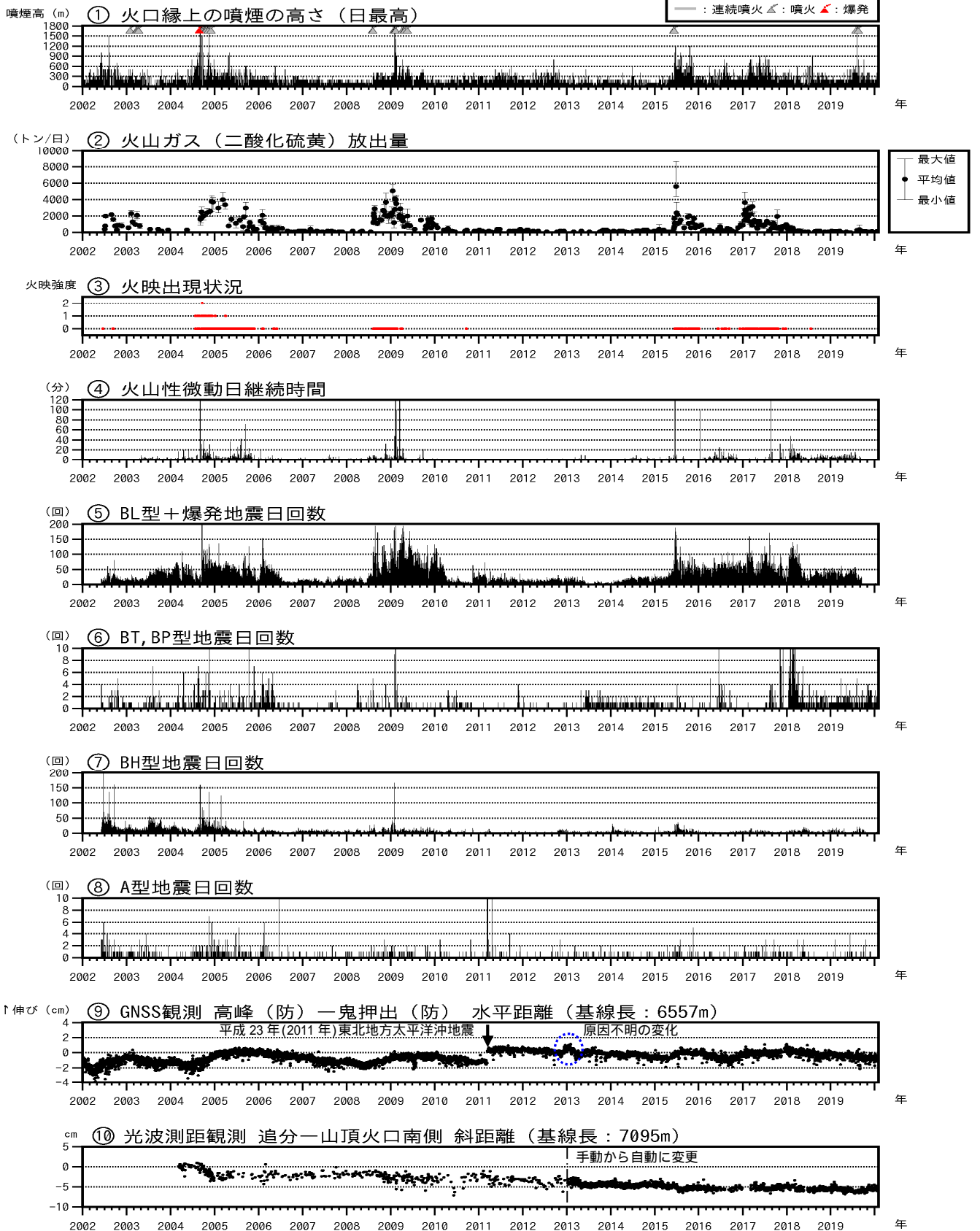
図3 浅間山 火山活動経過図（2002年1月1日～2020年1月31日）
