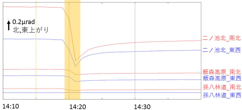
②傾斜計（分値）
