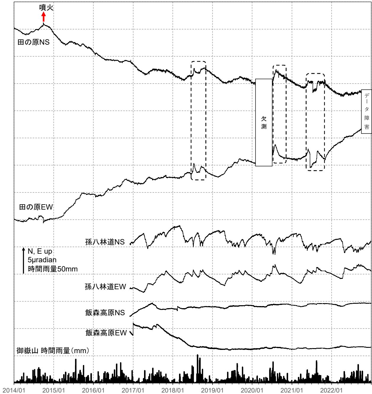
図 14 御嶽山 傾斜変動 (2014年1月1日～2022年12月31日)
