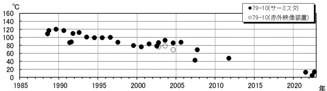
図6-2 御嶽山 79-10 火口の可視画像（上段）と火口底の温度変化（下段）
