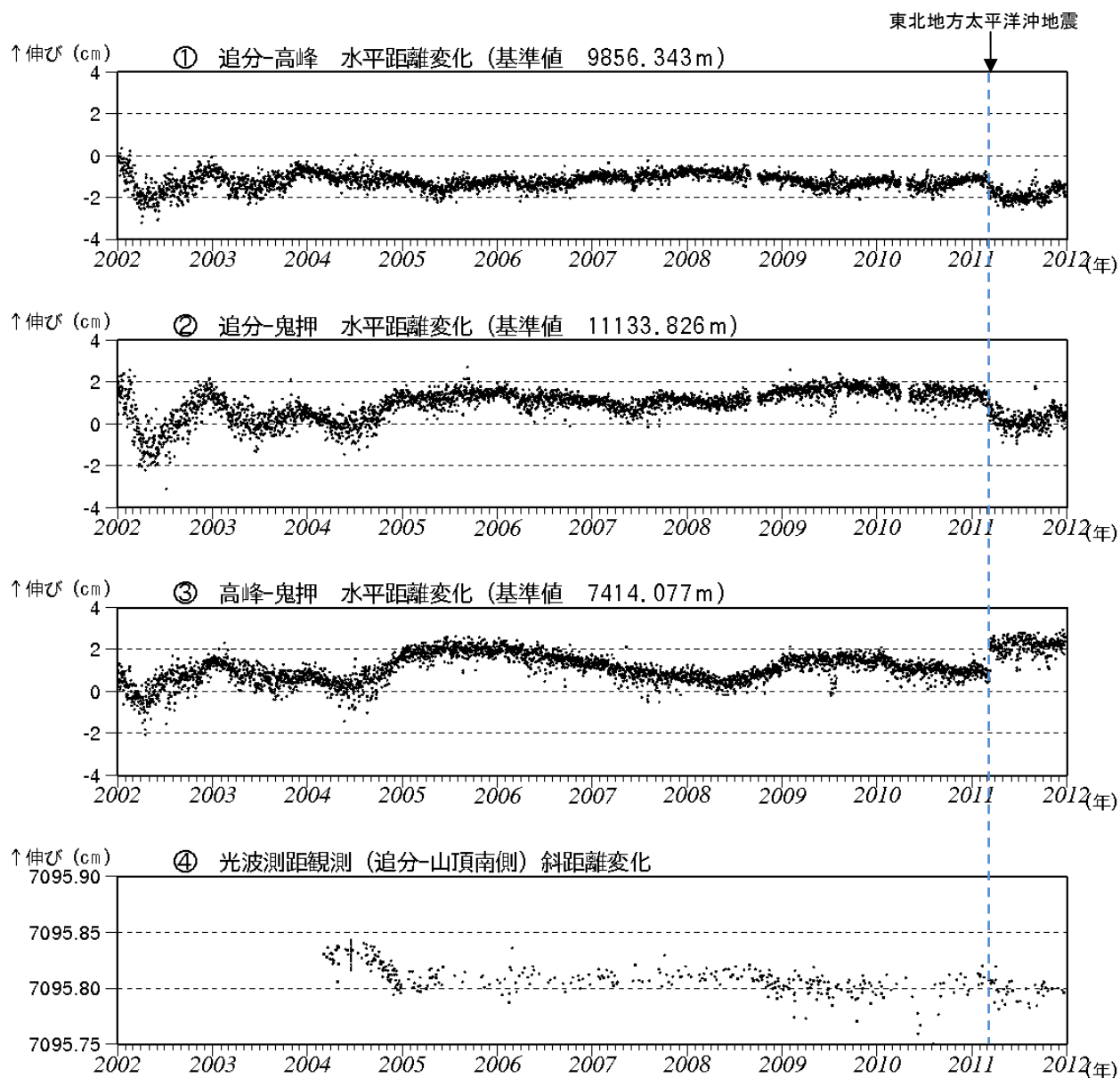
図7 浅間山 GPS 連続観測による水平距離変化及び光波測距観測 4) による変化
