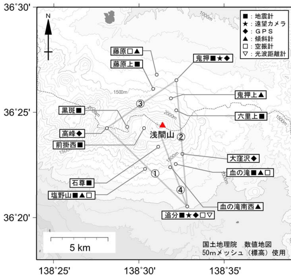
図 9 浅間山 気象庁の観測点配置図（小さな白丸は観測点位置を示しています） GPS 基線①～③は図 7 の①～③に対応しています。 光波測距測線④は図 4 の 10 及び図 7 の④に対応しています。
