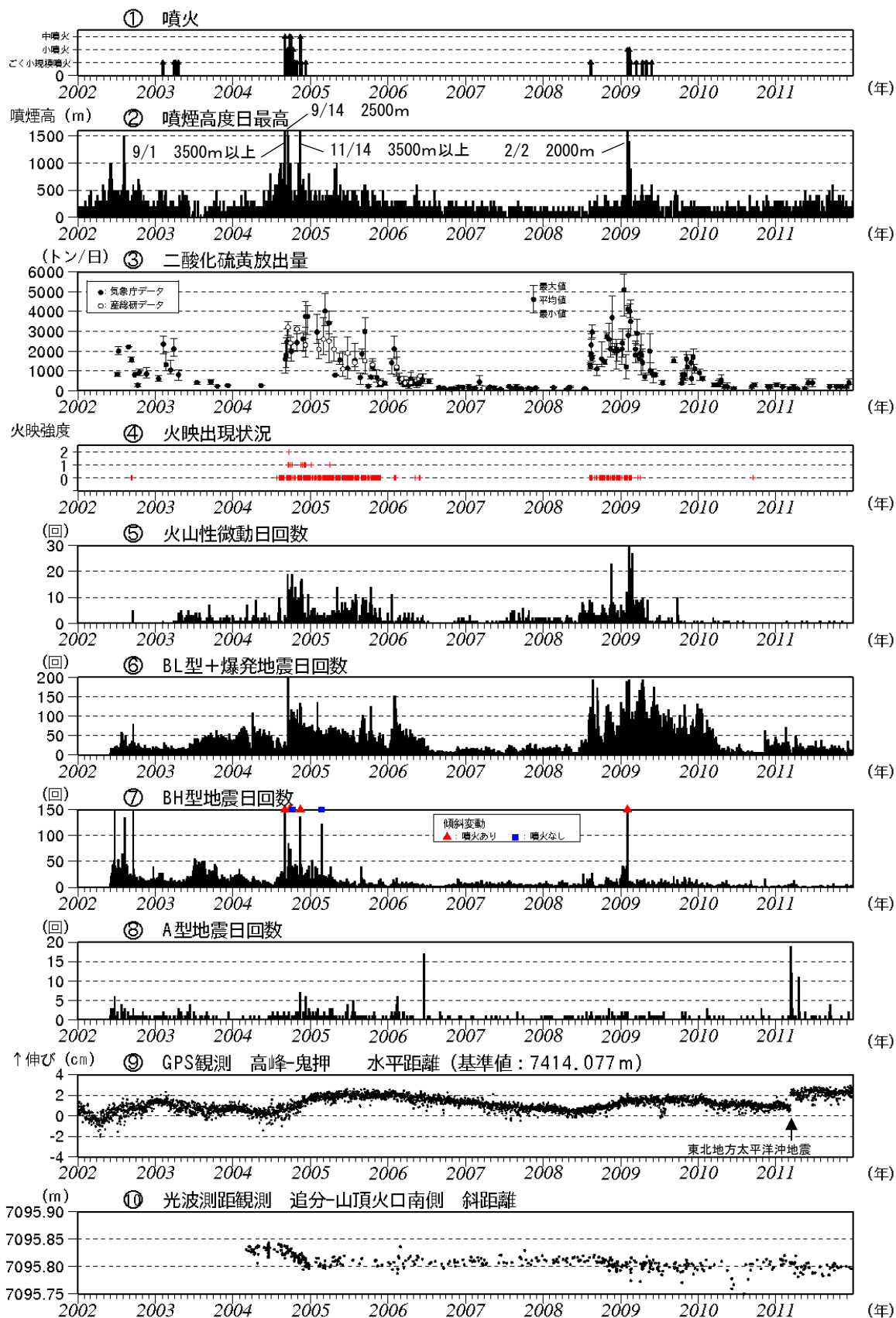
図4※ 浅間山 最近の火山活動の推移 (2002年1月1日～2011年12月31日) (注釈は次ページに示します)
