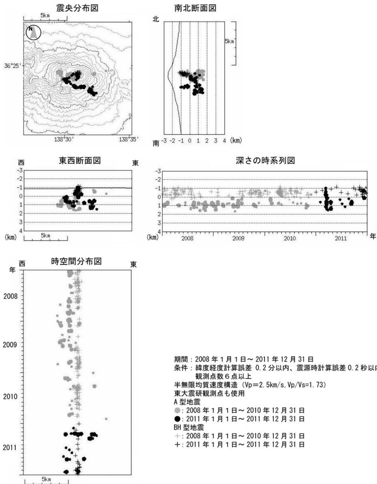
図 6※ 浅間山 火山性地震の震源分布 (2008 年 1 月 1 日～2011 年 12 月 31 日)
