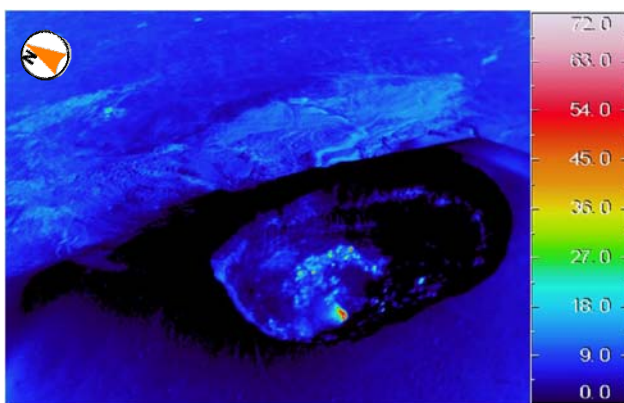
図 2 南西側上空から撮影した山頂火口内の地表面温度分布 1)
