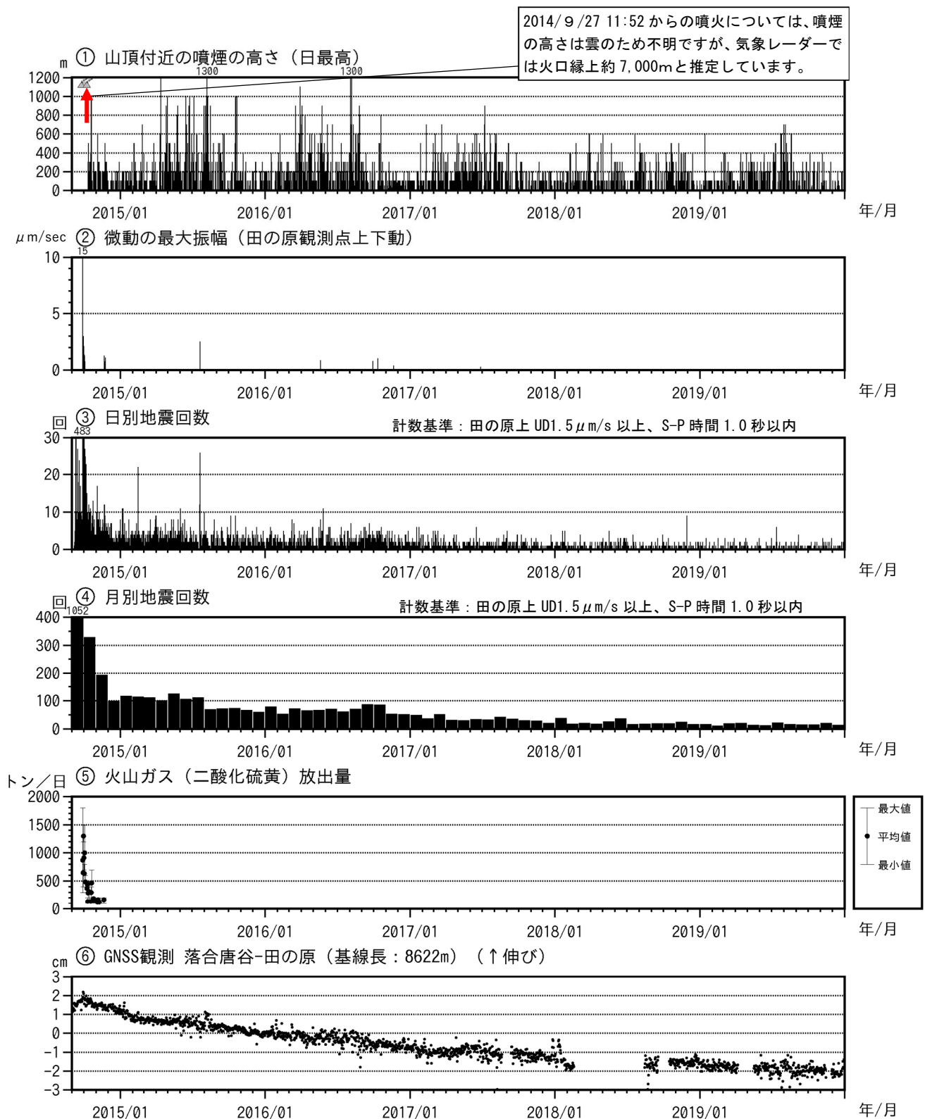
図4 御嶽山 最近の火山活動経過図（2014年9月1日～2019年12月31日）
