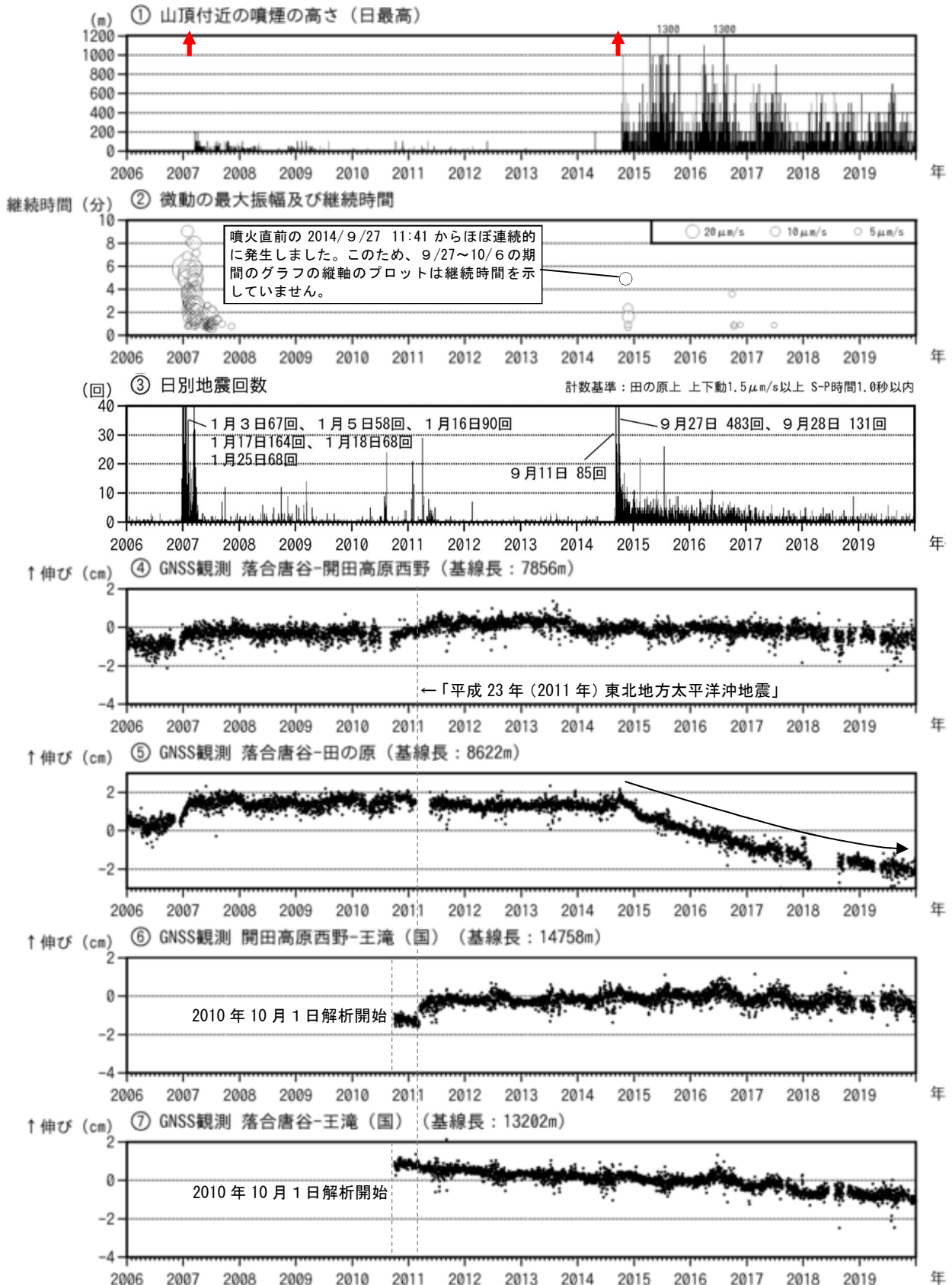
図5 御嶽山 長期間の火山活動経過図（2006年1月1日～2019年12月31日）
