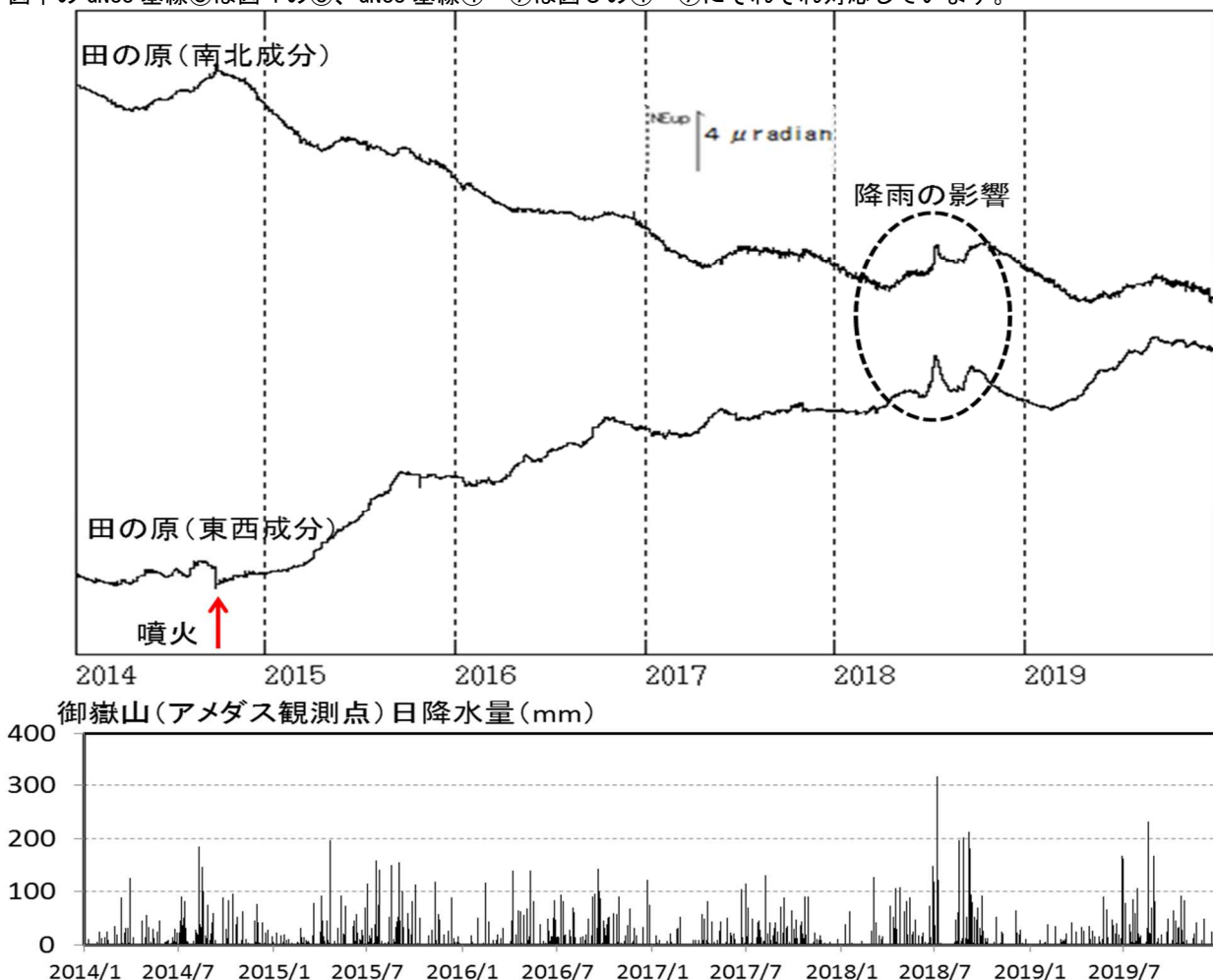
図7 御嶽山 田の原観測点の傾斜変動（2014年1月1日～2019年12月31日）
