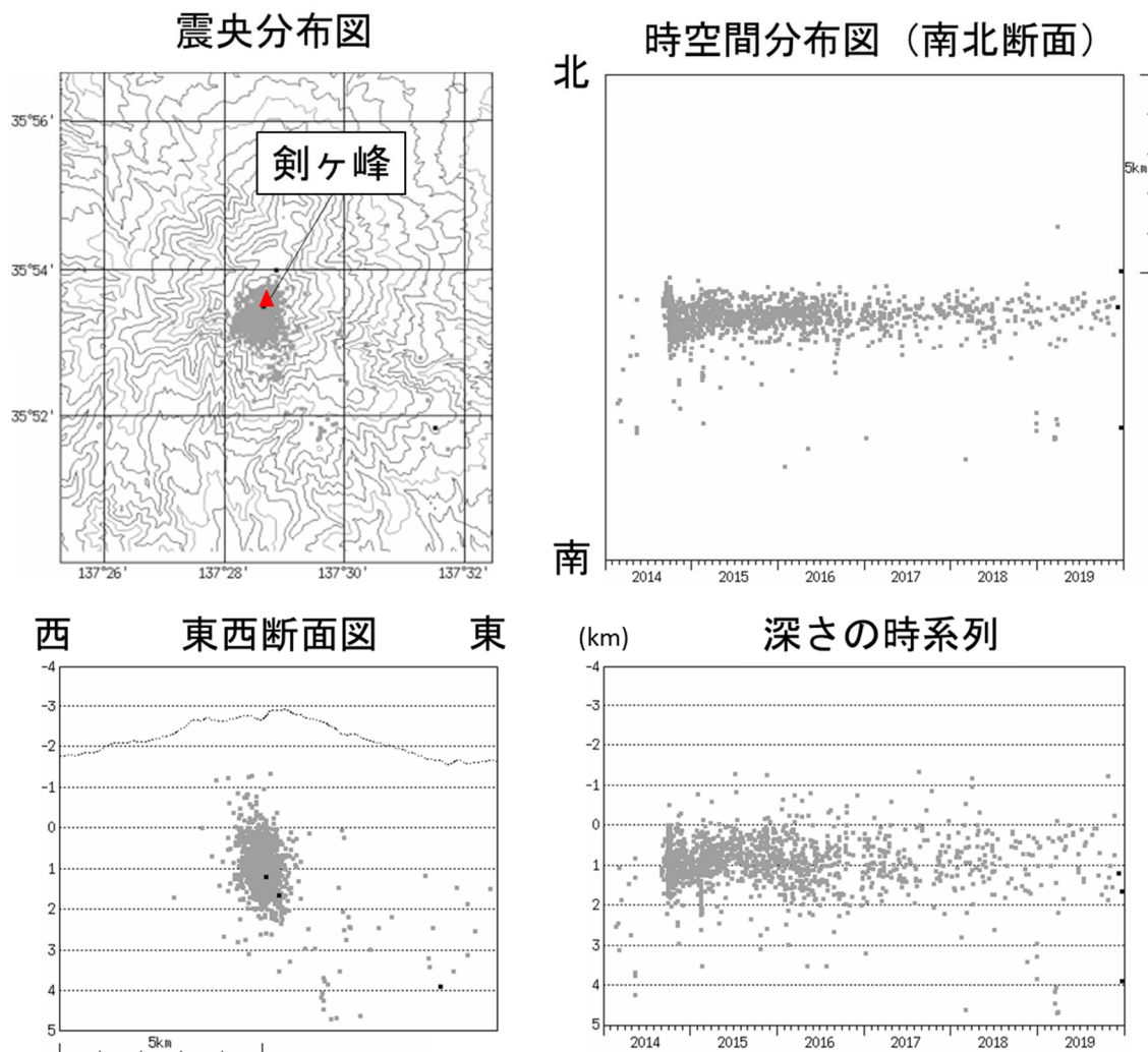
図 2 御嶽山 震源分布図（2014 年 1 月 1 日～2019 年 12 月 31 日）
