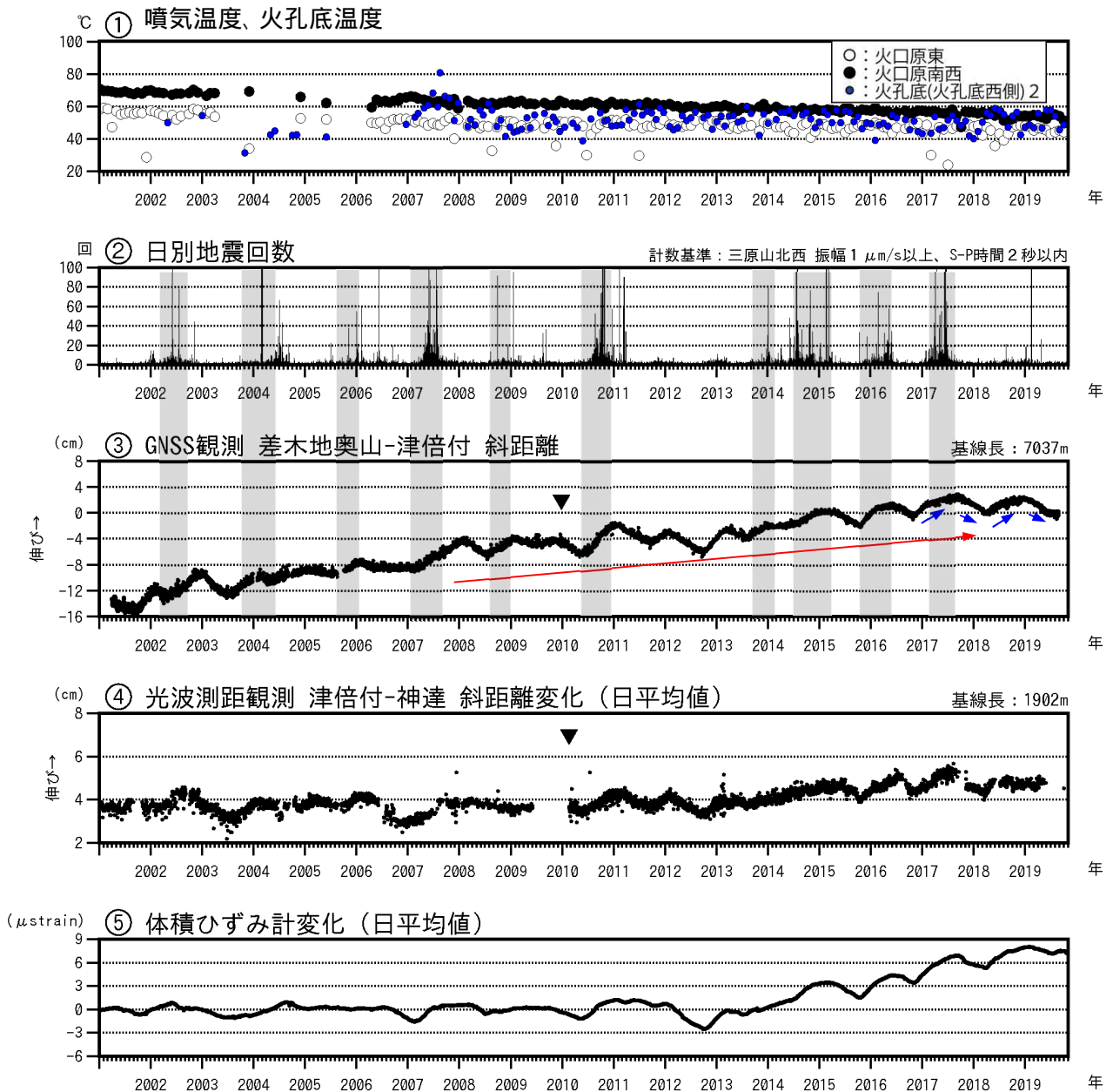
図2 伊豆大島 最近の火山活動経過図（2001年1月～2019年10月31日）
