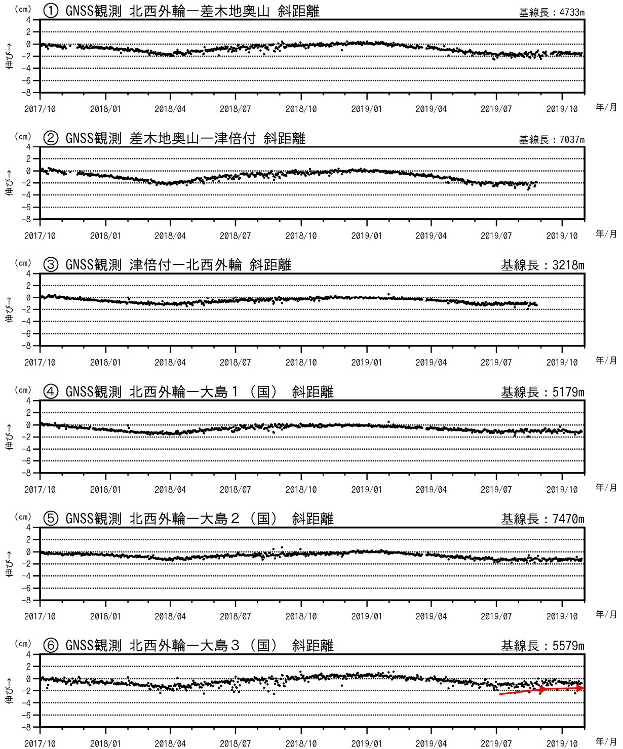
図 3 - 2 伊豆大島 GNSS 連続観測による基線長変化(2017 年 8 月 ~ 2019 年 10 月 31 日) (国): 国土地理院、 ~ は図 10 の GNSS 基線 ~ に対応、グラフの空白部分は欠測。 2010 年 10 月及び 2016 年 1 月以降のデータについては、解析方法を変更しています。 ・長期的な島全体の膨張傾向は継続しています。約 1 年周期で膨張と収縮を繰り返す短期的な地殻変動がみられ、最近では、一部の基線で 7 月頃から膨張に転じていましたが、9 月頃からは鈍化がみられています(赤矢印)。
