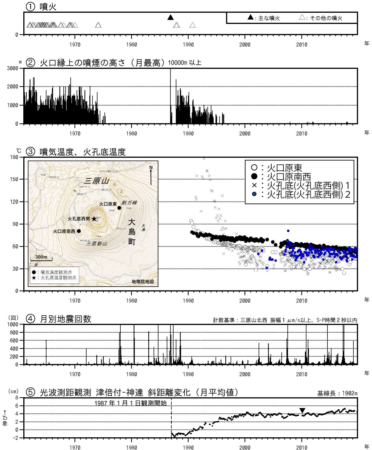
図1 伊豆大島 長期間の火山活動経過図（1961年1月～2019年10月31日） 1991年12月18日までは火口縁上130m以上、2002年2月28日までは火口縁上300m以上の噴煙の高さを観測していました。 火口原東、火口原南西：サーミスタ温度計により直接測定した噴気温度。 火孔底(火孔底西側)1：赤外放射温度計により離れた場所から測定した火孔底温度。 火孔底(火孔底西側)2：赤外熱映像装置により離れた場所から測定した火孔底温度。 地震回数には伊豆大島周辺海域で発生した地震も一部含まれています。 グラフの空白部分は欠測、 は機器更新。
