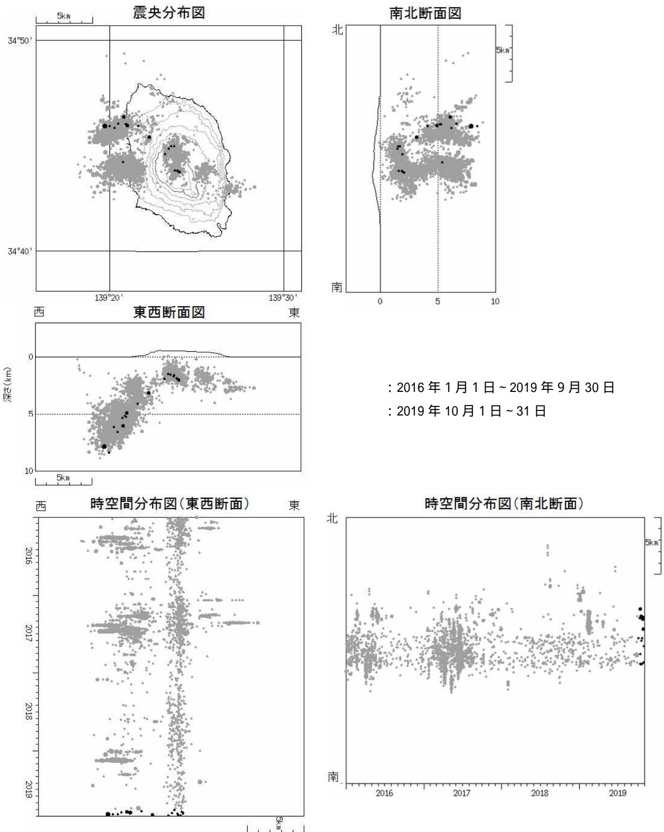
図4 伊豆大島 震源分布図（2016年1月1日～2019年10月31日）
