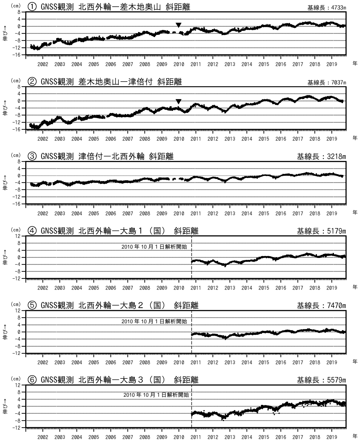
図3-1 伊豆大島 GNSS連続観測による基線長変化(2001年1月~2019年10月31日)
