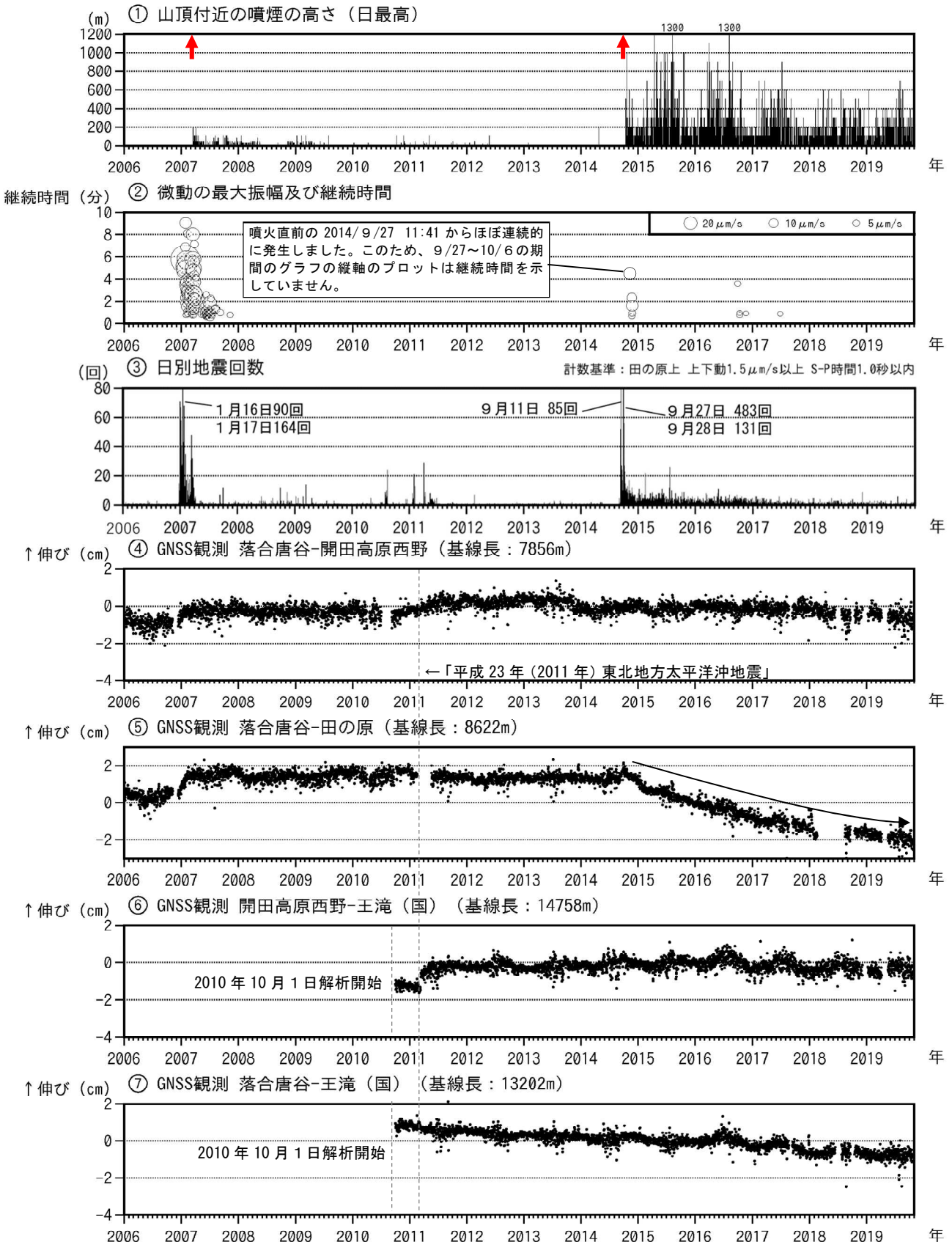
図5 御嶽山 長期間の火山活動経過図（2006年1月1日～2019年10月31日）
