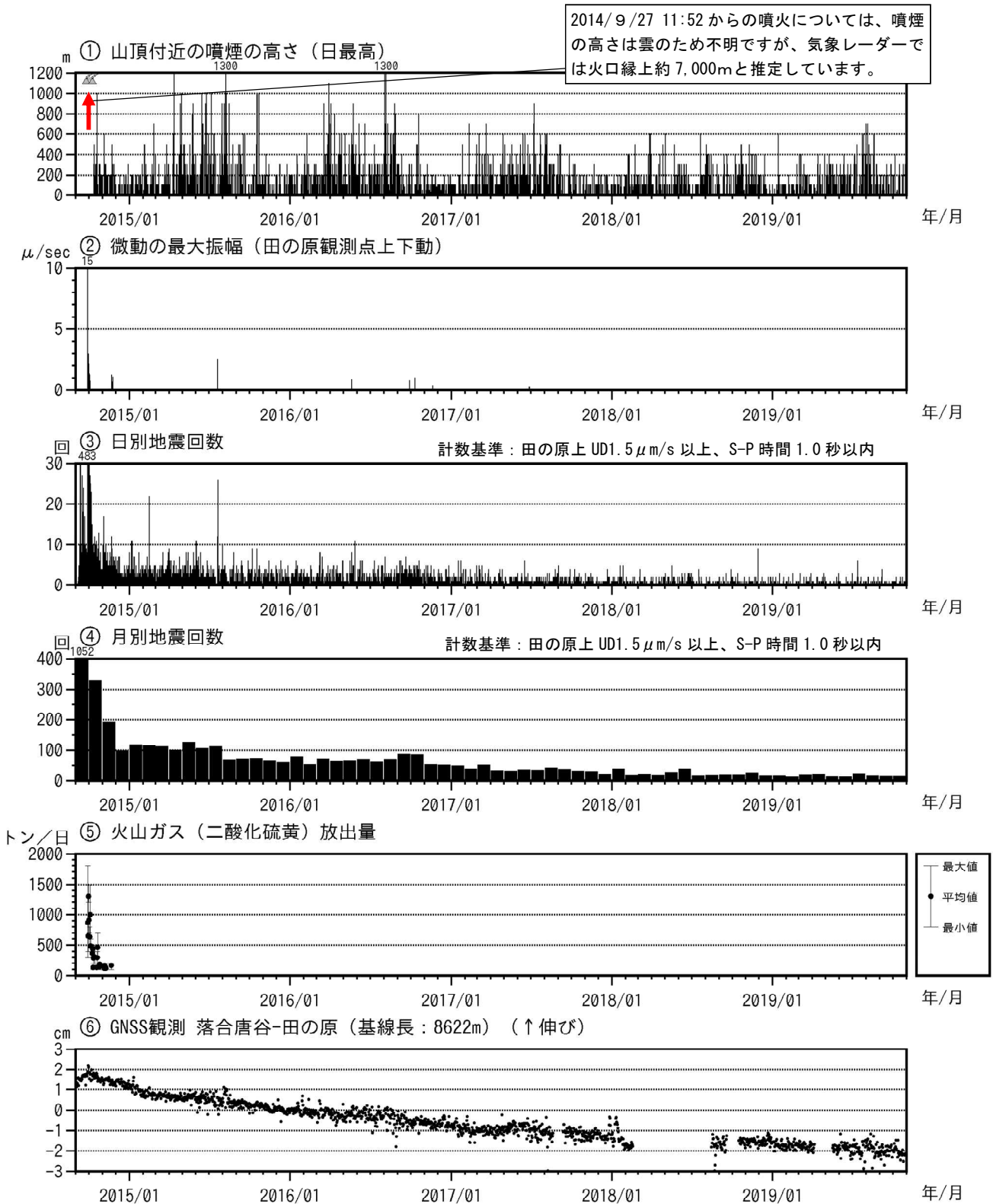
図4 御嶽山 最近の火山活動経過図（2014年9月1日～2019年10月31日）
