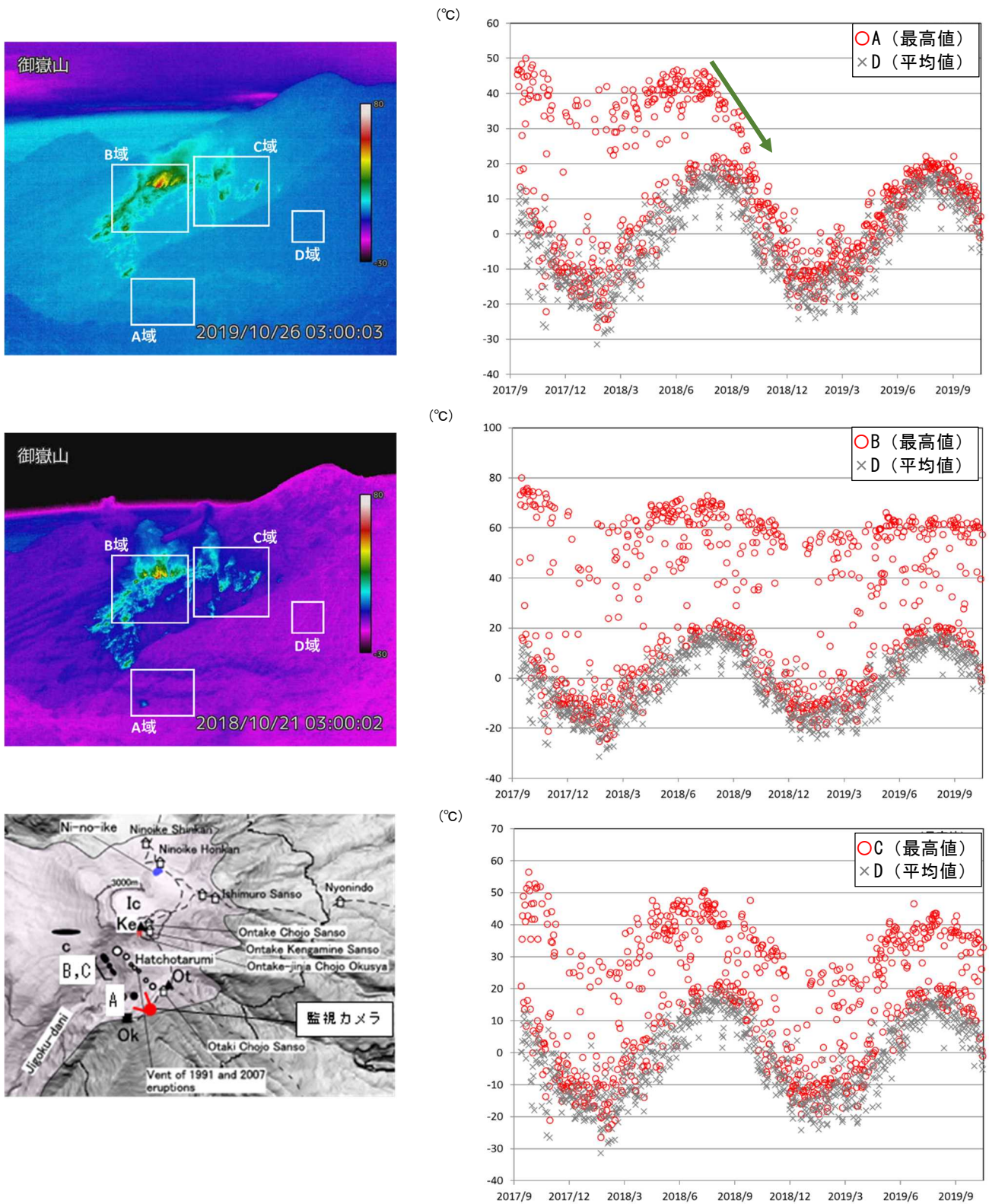
図3 御嶽山 奥の院赤外熱映像カメラによる剣ヶ峰南西側における最高温度の推移 （2017年9月13日～2019年10月31日）と同カメラの位置（左下図はOikawa et al., 2016に加筆） A～Cは地熱域、Dは非地熱域を示します。
