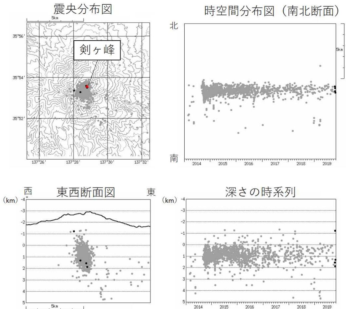
図2 御嶽山 震源分布図（2014年1月1日～2019年10月31日）
